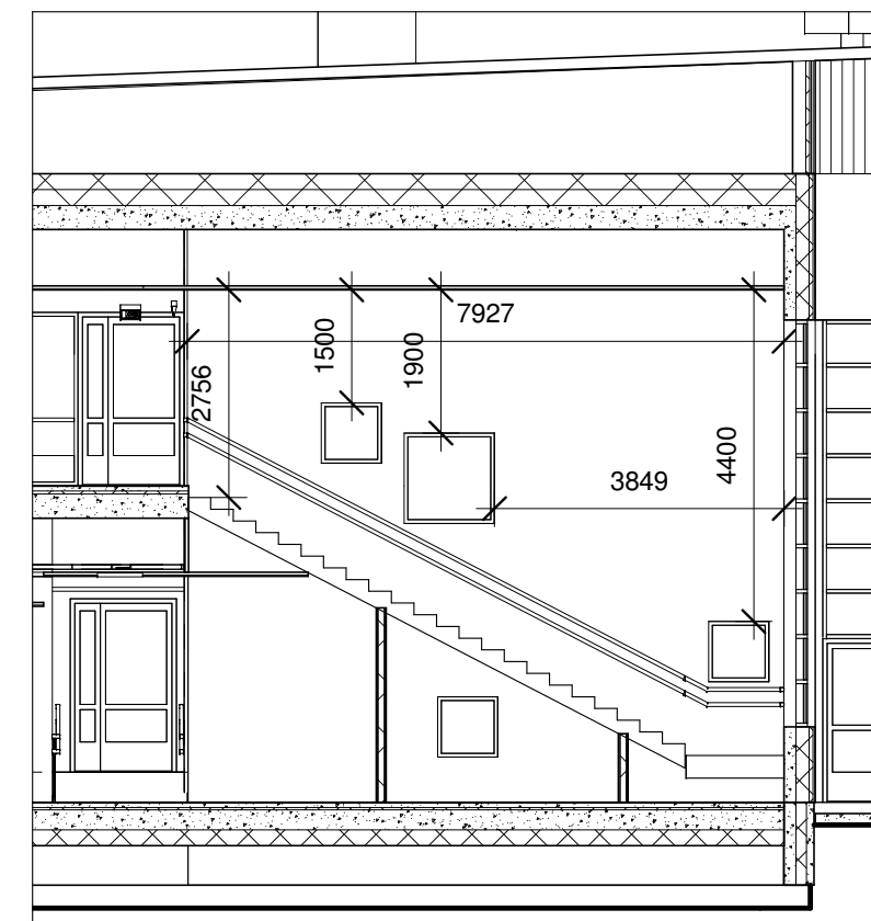
LEIKKAUS A-K 1/100
