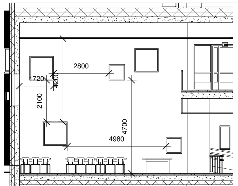
LEIKKAUS A-J 1/100
