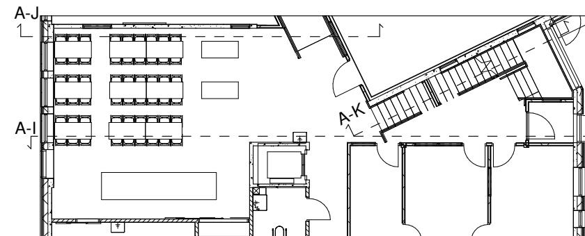
POHJAPIIRROS 1.KRS 1/200
