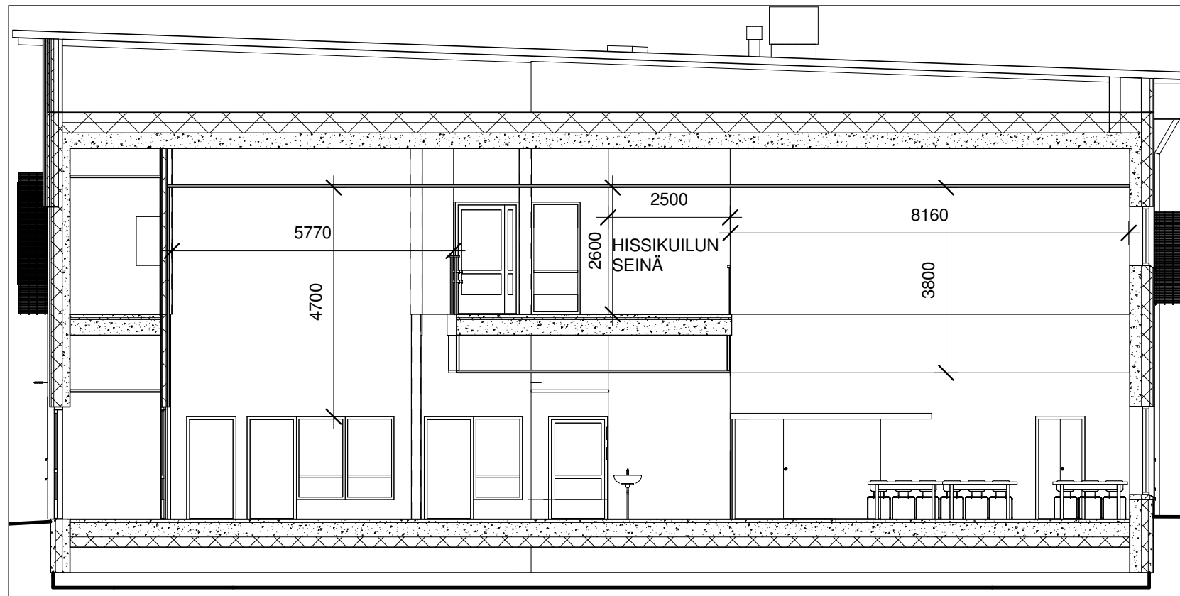
LEIKKAUS A-I 1/100
