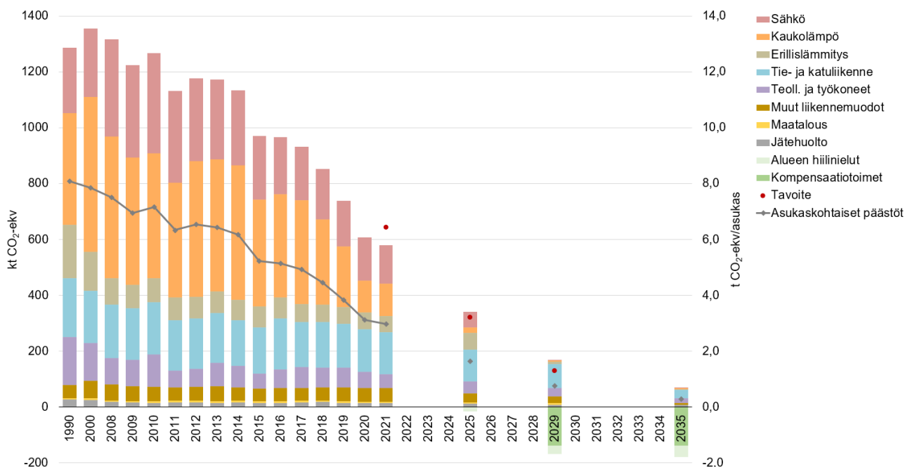
Bild 6. De normerade utsläppen som beräknats med metoden CO2-rapport i Åbo 1990, 2000 och 2008–2021, den beräknade utsläppsökningen, kolsänkorna och kompensationsåtgärderna för 2025, 2029 och 2035 samt utsläppsmålen för 2021, 2025 och 2029 (längdaxel i vänster); de invånarspecifika utsläppen (längdaxel i höger).
