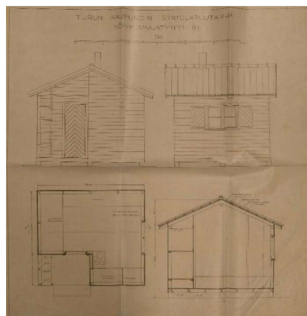
A2-päivämajatyypin ja B1-yöpymismajatyypin piirustukset vuodelta 1934, tilapalveluiden arkisto.
