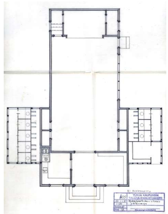
Kalustovajan laajennus kerhorakennukseksi, toteutumaton suunnitelma 13.1.1941, tilapalveluiden arkisto.
