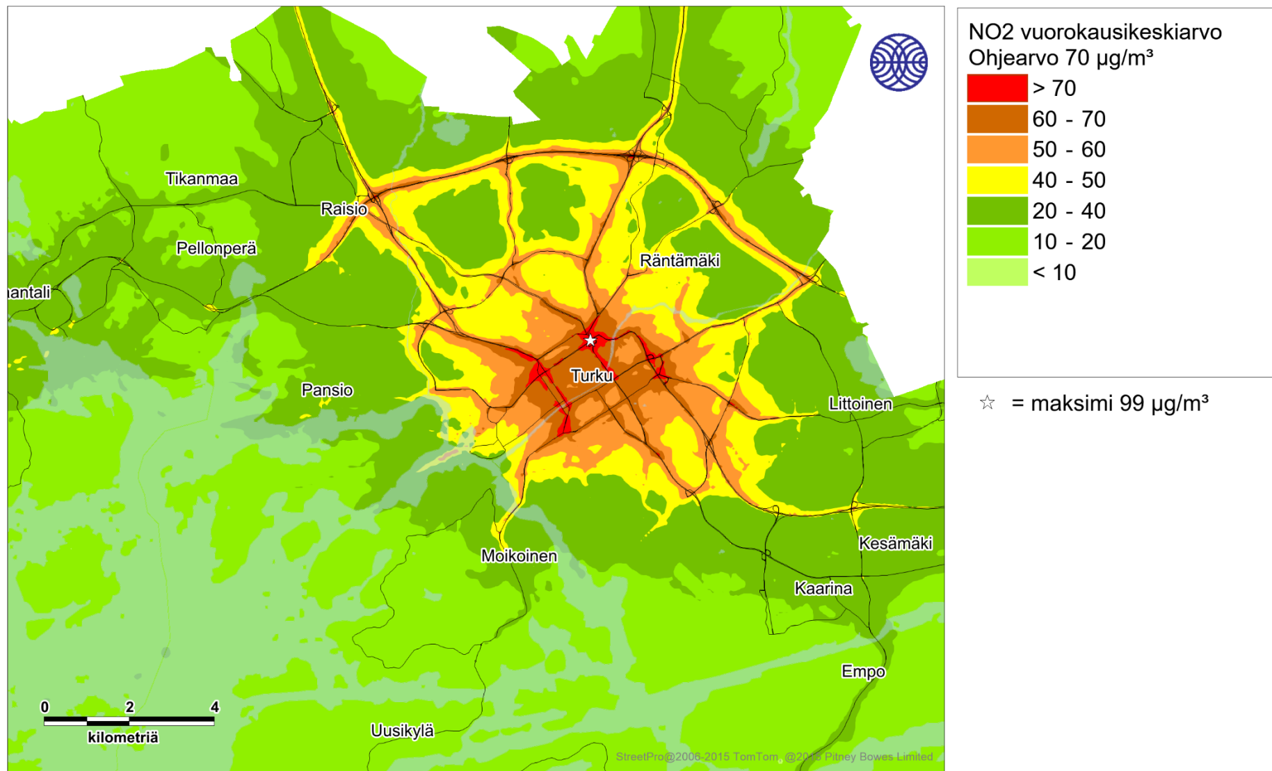
Kuva 4. Kaikkien päästölähteiden ja taustapitoisuuden yhdessä aiheuttama typpidioksidin korkein vuorokausiohjearvoon verrannollnen pitoisuus (µg/m³) tarkastelujaksolla 2016-2018.
