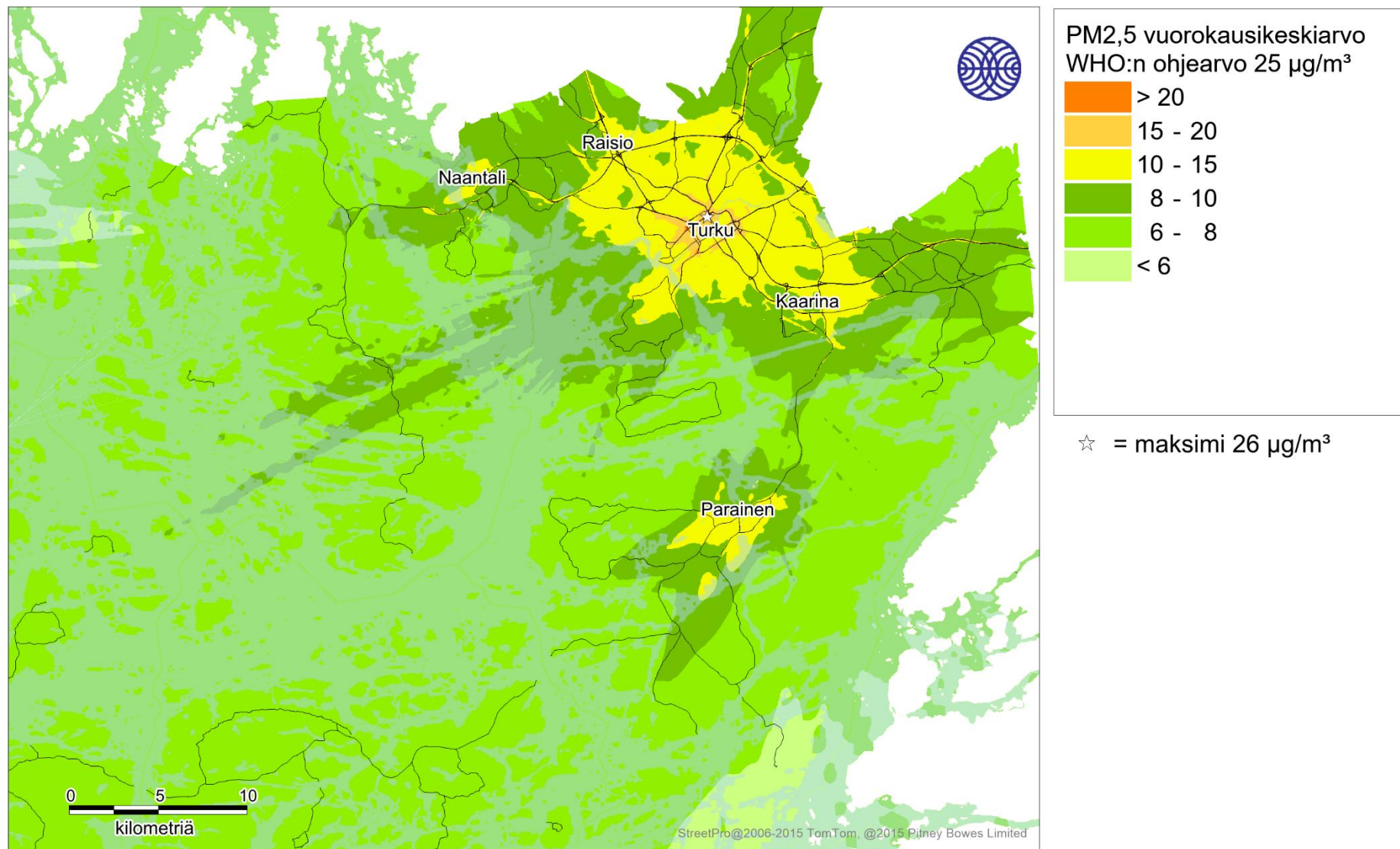
Kuva 21. Kaikkien päästölähteiden ja taustapitoisuuden aiheuttama pienhiukkasten korkein WHO:n vuorokausiohjearvoon verrannollinen pitoisuus (µg/m³) tarkastelujaksolla 2016-2018.
