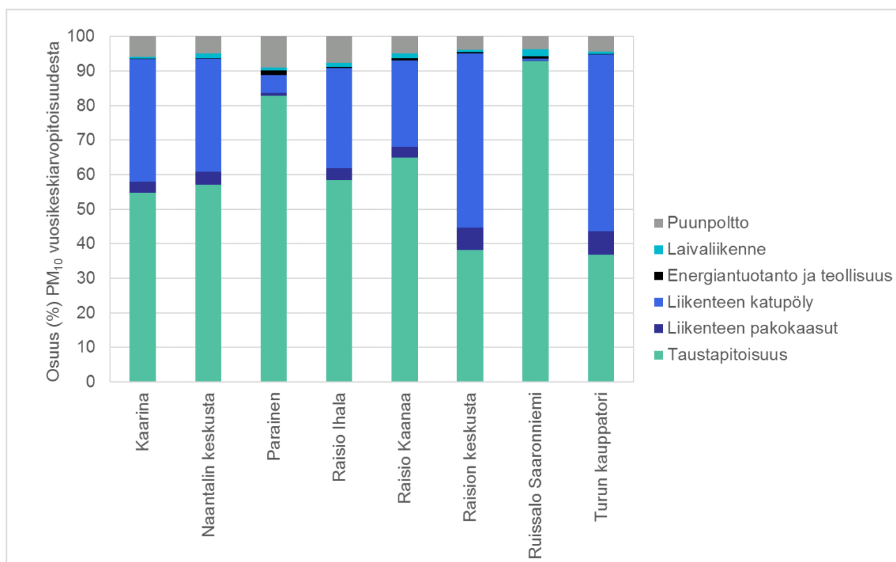
Kuva 33. Eri päästölähdesektoreiden osuus mallinnetuista hengitettävien hiukkasten vuosikeskiarvopitoisuuksista ilmanlaadun mittauspisteissä vuonna 2018.
