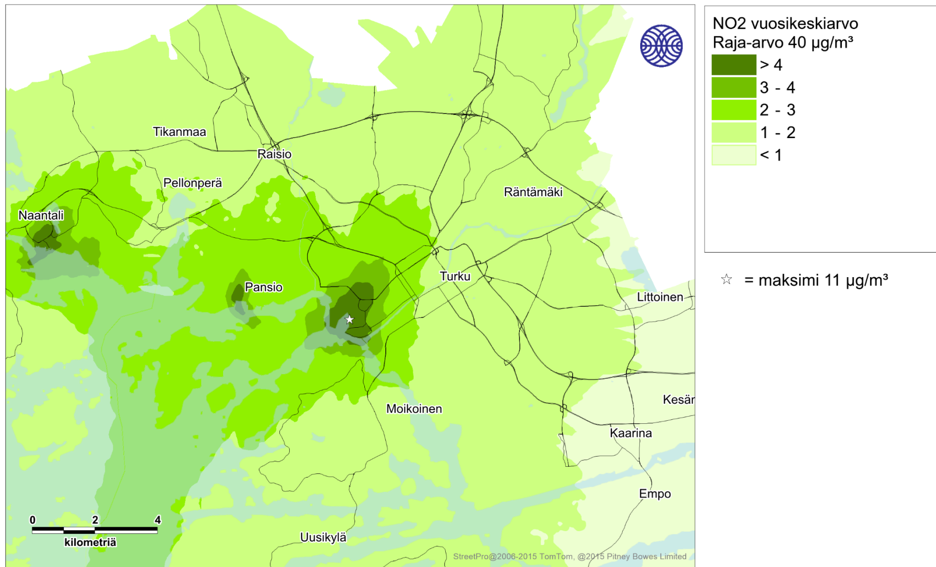
Kuva 14. Laivaliikenteen päästöjen aiheuttama typpidioksidin korkein vuosikeskiarvopitoisuus (µg/m³) tarkastelujaksolla 2016-2018.
