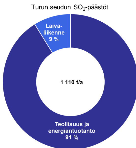
Kuva 41. Turun seudun rikkidioksidin kokonaispäästöt sekä eri päästölähteiden osuudet vuonna 2018.
