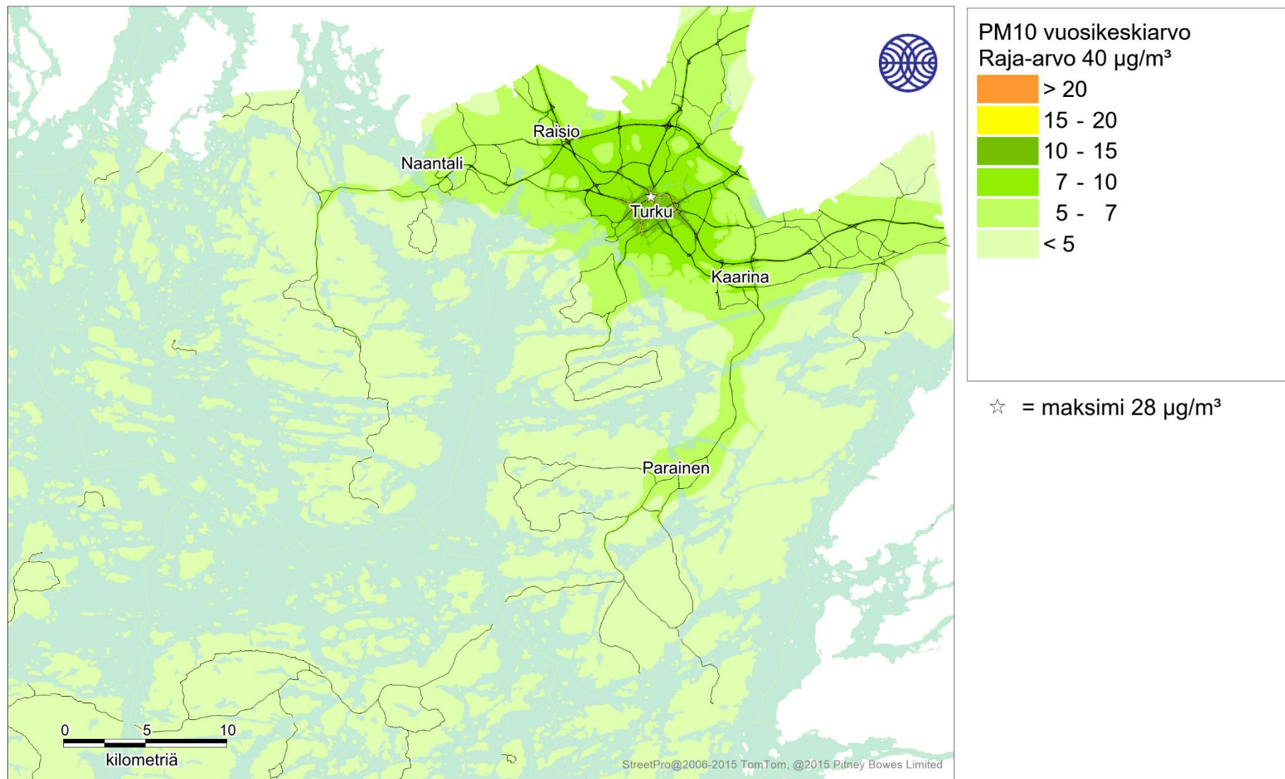
Kuva 39. Kaikkien päästölähteiden ja taustapitoisuuden yhdessä aiheuttama hengitettävien hiukkasten korkein vuosikeskiarvopitoisuus (µg/m³) tarkastelujaksolla 2016-2018.
