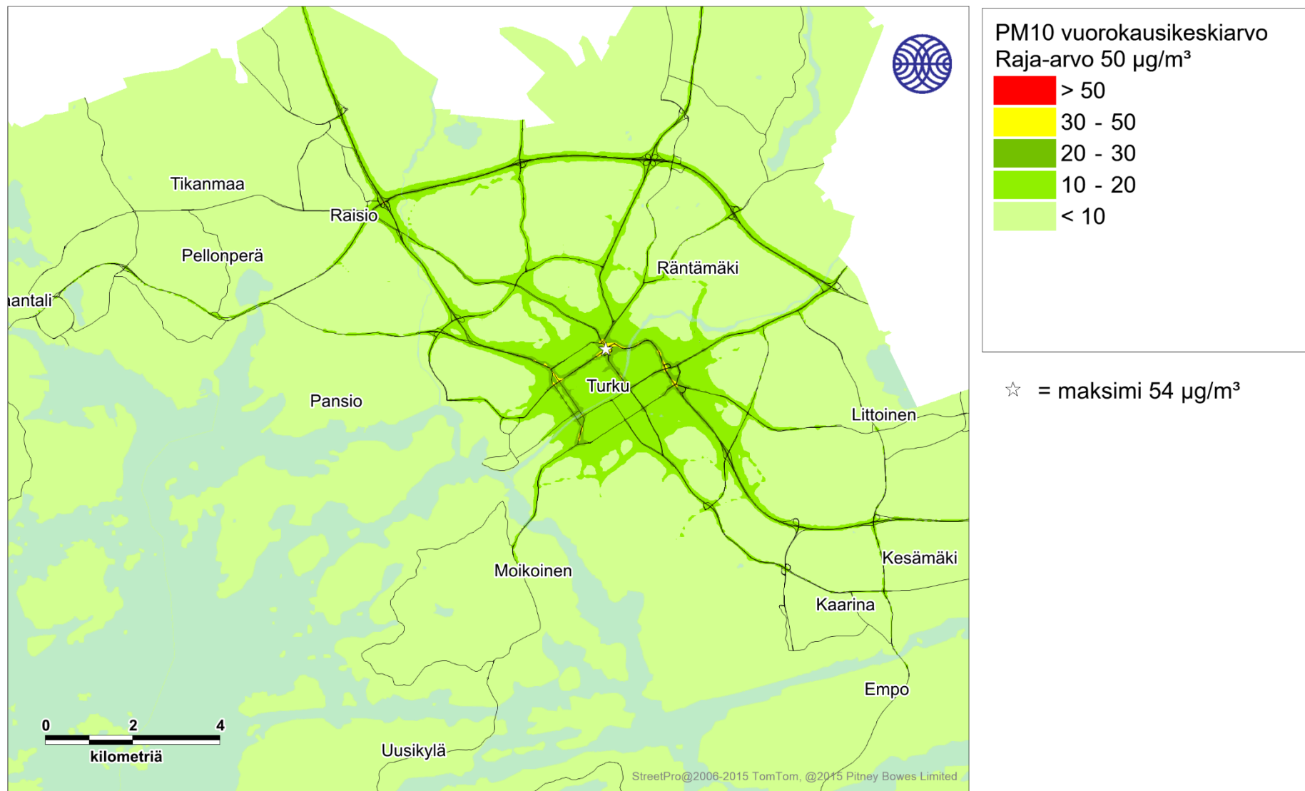
Kuva 46. Autoliikenteen päästöjen aiheuttama hengitettävien hiukkasten korkein vuorokausiraja-arvoon verrannollinen pitoisuus (µg/m³) tarkastelujaksolla 2016-2018.
