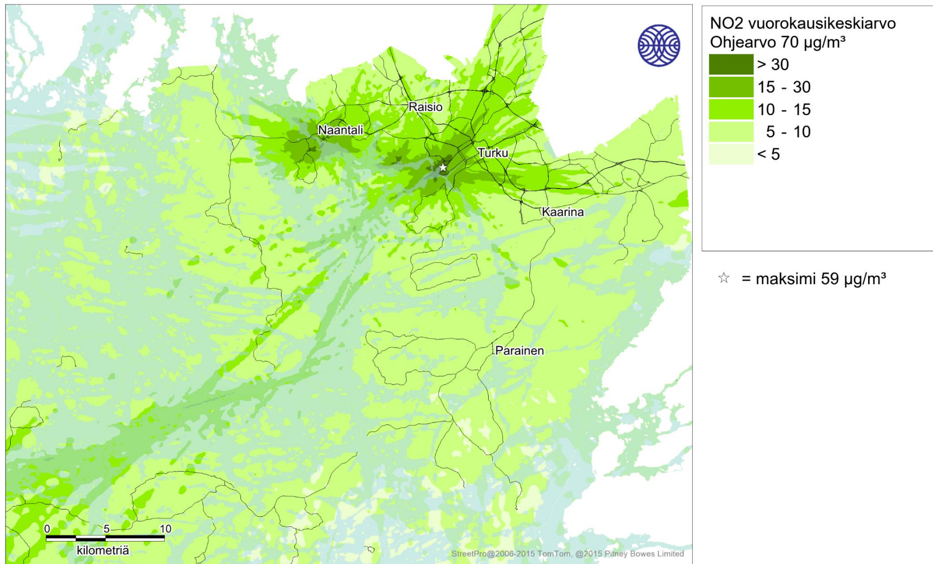
Kuva 15. Laivaliikenteen päästöjen aiheuttama typpidioksidin korkein vuorokausiohjearvoon verrannollinen pitoisuus (µg/m 3 ) tarkastelujaksolla 2016-2018.
