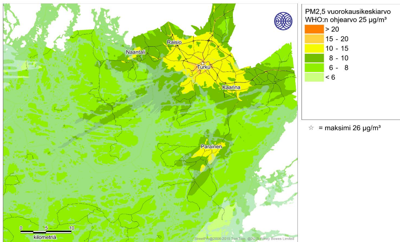
Kuva 8. Autoliikenteen, energiantuotannon, teollisuuden ja puunpoltton päästöjen sekä alueellisen taustapitoisuuden (vuosikeskiarvona 4,4 µg/m³) yhdessä aiheuttama pienhiukkasten (PM 2,5 ) korkein WHO:n vuorokausiohjearvoon verrannollinen pitoisuus (µg/m³) Turun seudulla vuonna 2018.
