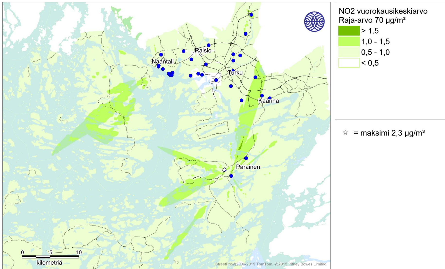
Kuva 11. Energiantuotannon ja teollisuuden päästöjen aiheuttama typpidioksidin korkein vuorokausiohjearvoon verrannollinen pitoisuus (µg/m³) tarkastelujaksolla 2016-2018.
