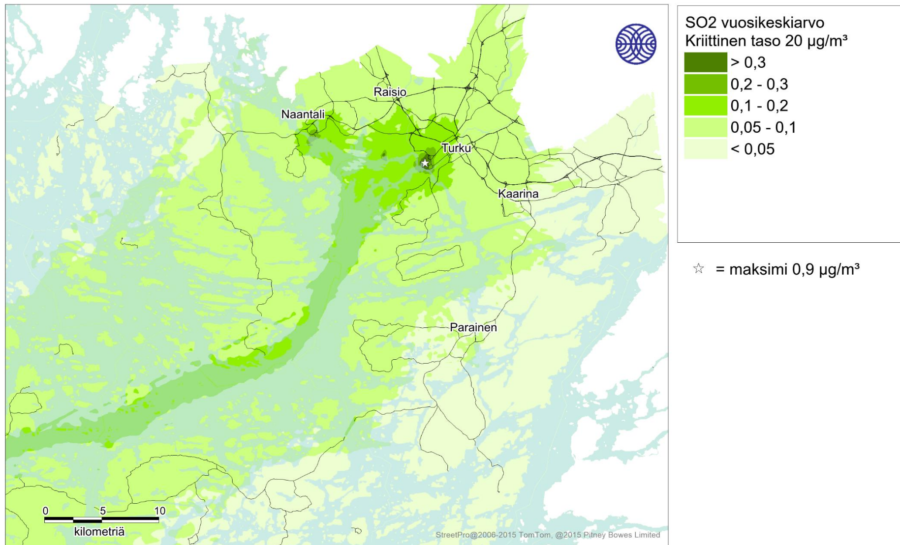
Kuva 55. Laivaliikenteen päästöjen aiheuttama rikkidioksidin korkein vuosikeskiarvopitoisuus (µg/m 3 ) tarkastelujaksolla 2016-2018.
