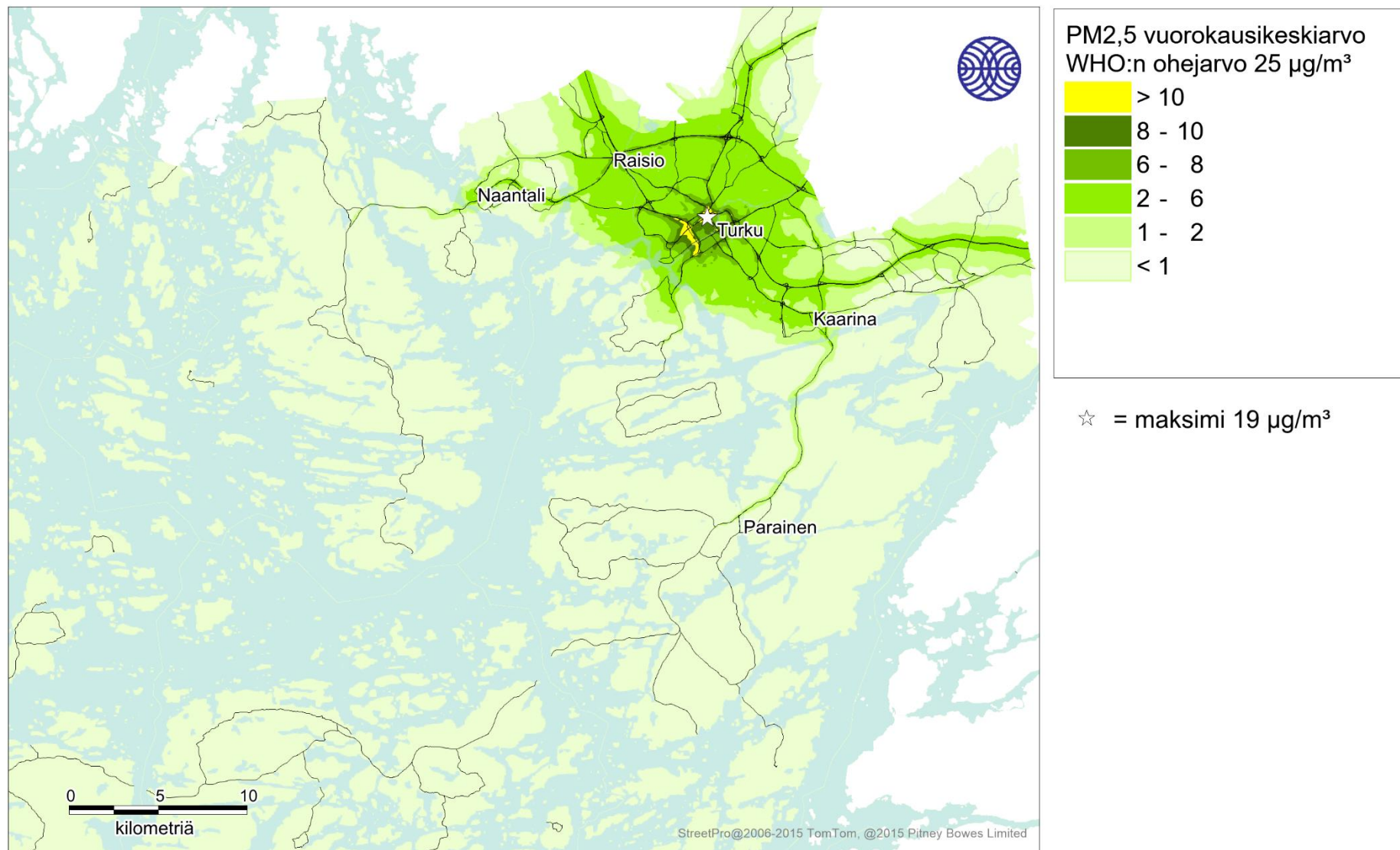
Kuva 25. Autoliikenteen päästöjen aiheuttama pienhiukkasten korkein WHO:n vuorokausiohjeeseen verrannollinen pitoisuus (µg/m³) tarkastelujaksolla 2016-2018.
