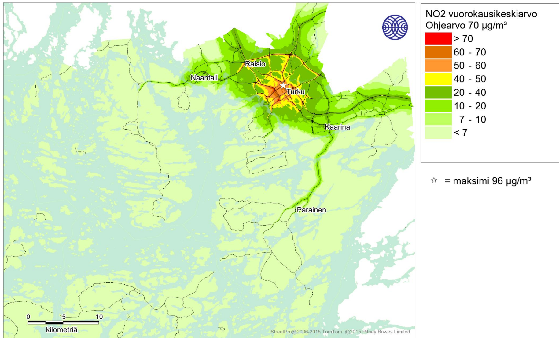
Kuva 7. Autoliikenteen päästöjen aiheuttama typpidioksidin korkein vuorokausiohjearvoon verrannollinen pitoisuus (µg/m³) tarkastelujaksolla 2016-2018.
