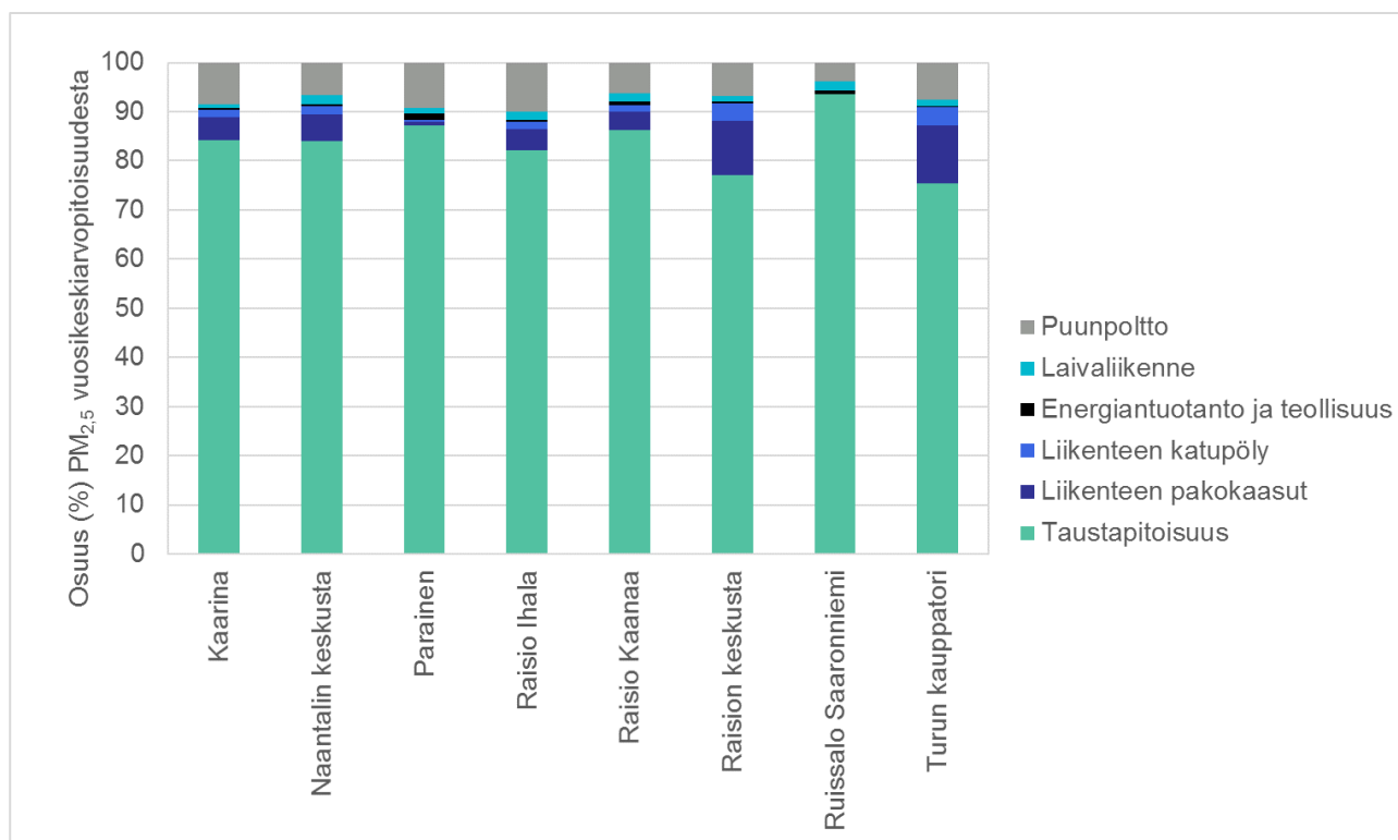
Kuva 32. Eri päästölähdesektoreiden osuus mallinnetuista pienhiukkasten vuosikeskiarvopitoisuuksista ilmanlaadun mittauspisteissä vuonna 2018.
