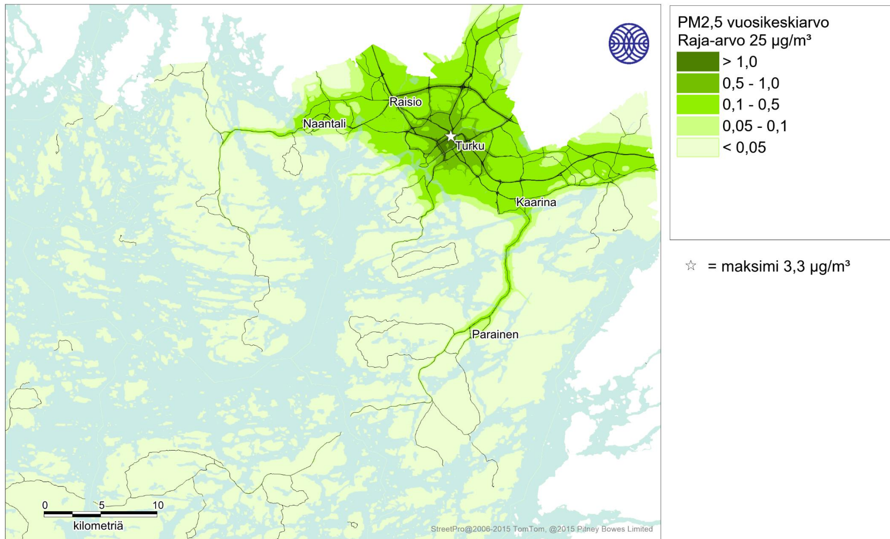
Kuva 23. Autoliikenteen päästöjen aiheuttama pienhiukkasten korkein vuosikeskiarvopitoisuus (µg/m³) tarkastelujaksolla 2016-2018.
