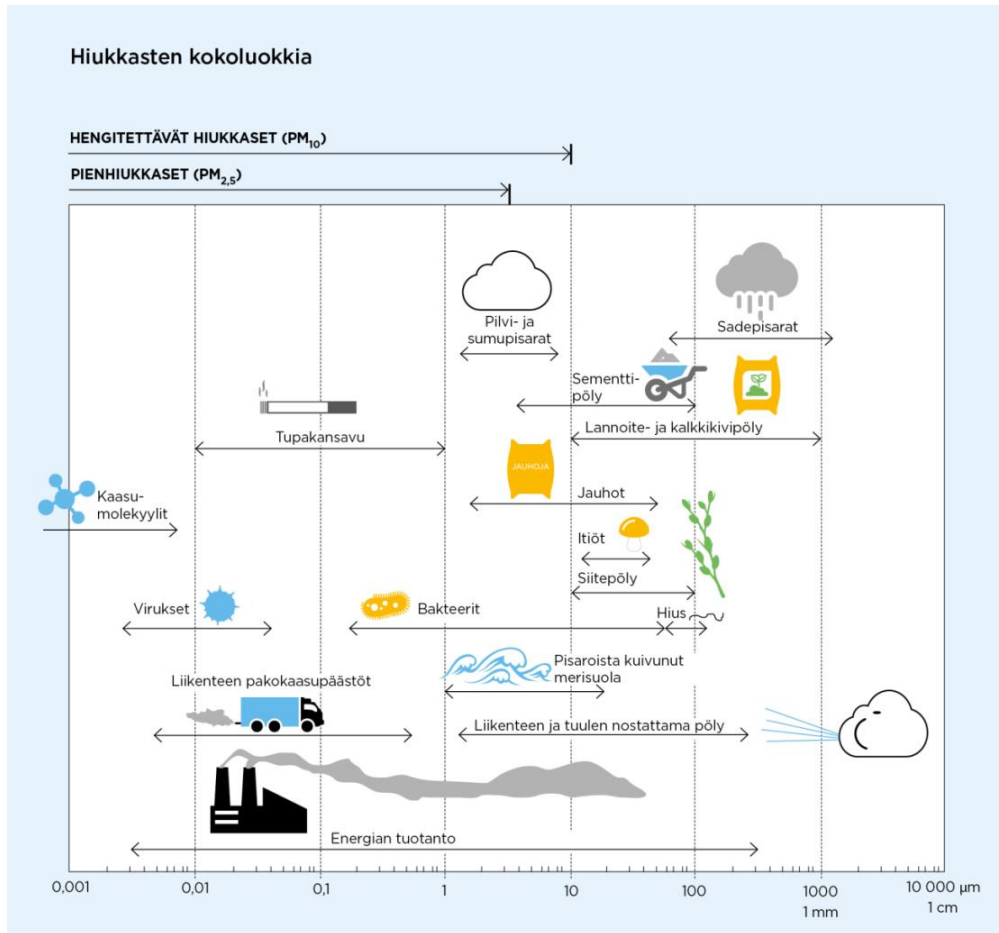
Kuva 38. Hiukkasten kokoluokkia. Hiukkasten koko ilmaistaan halkaisijana mikrometreissä (µm). Mikro (µ) etuliite tarkoittaa miljoonasosaa. 1 µm on siten metrin miljoonasosa eli millimetrin tuhannesosa.
