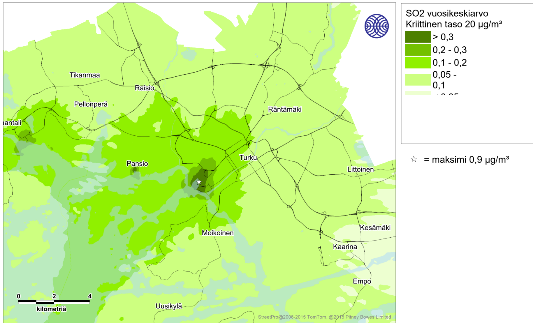
Kuva 56. Laivaliikenteen päästöjen aiheuttama rikkidioksidin korkein vuosikeskiarvopitoisuus (µg/m³) tarkastelujaksolla 2016-2018.
