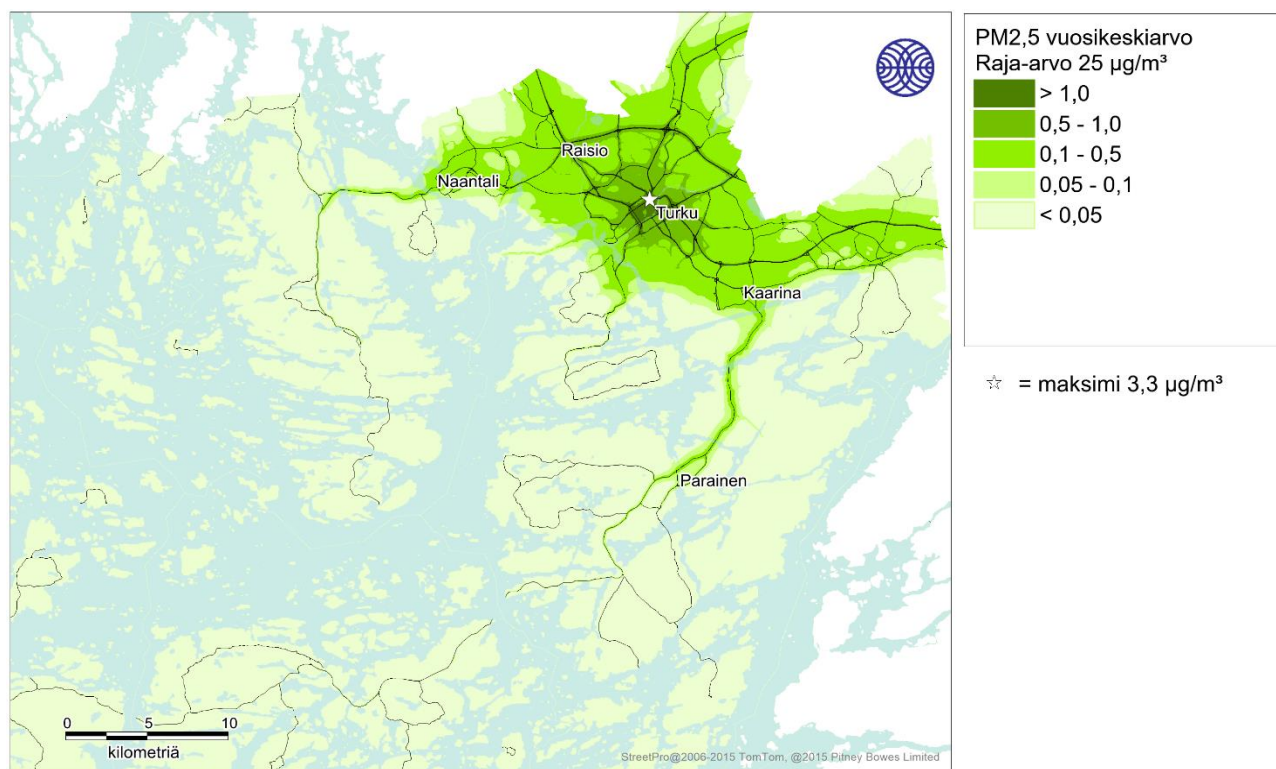
Kuva 9. Autoliikenteen päästöjen yksinään aiheuttama pienhiukkasten korkein vuosikeskiarvopitoisuus (µg/m³) Turun seudulla vuonna 2018 ilman alueellista taustapitoisuutta.
