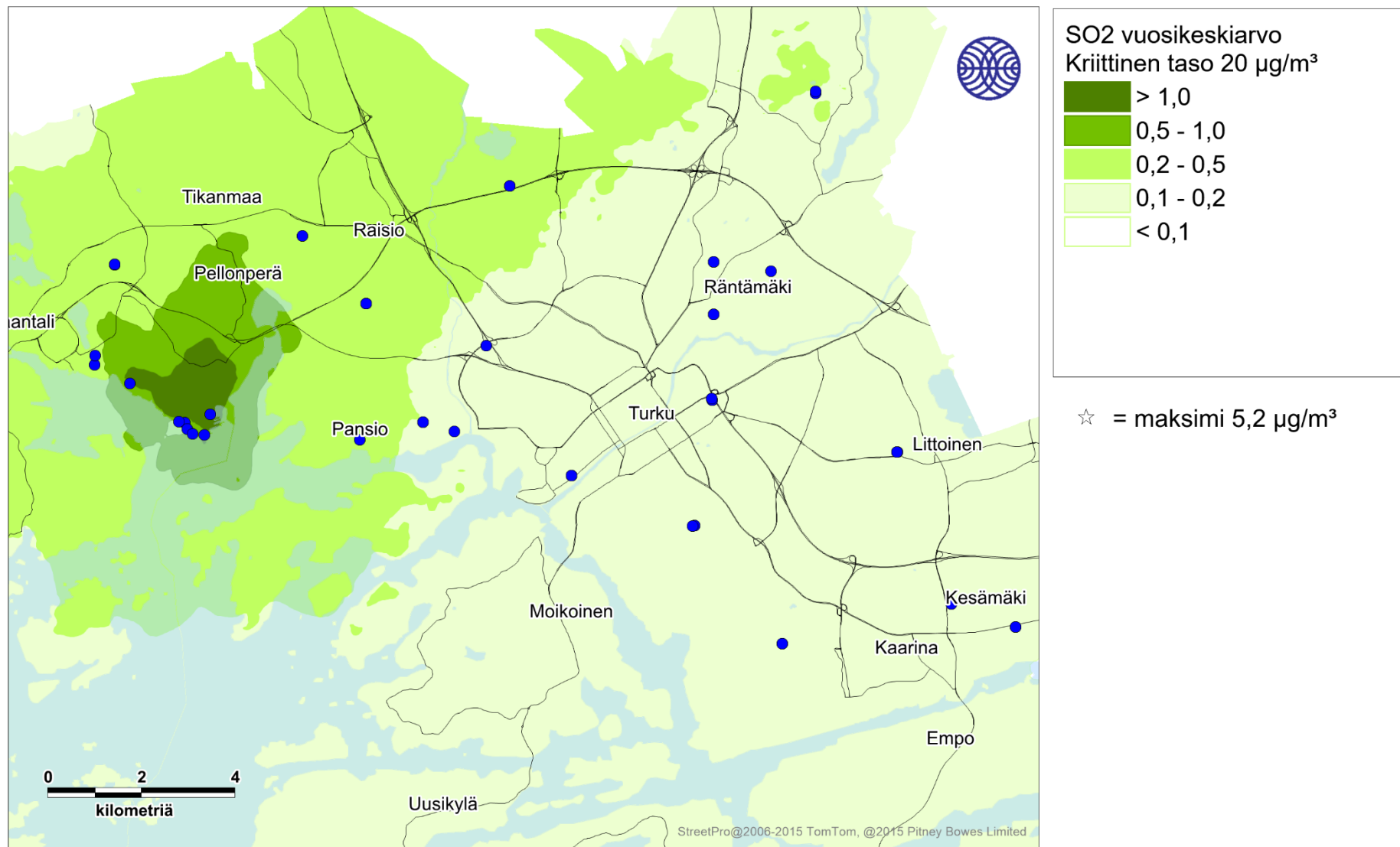
Kuva 52. Energiantuotannon ja teollisuuden päästöjen aiheuttama rikkidioksidin korkein vuosikeskiarvopitoisuus (µg/m³) tarkastelujaksolla 2016-2018.
