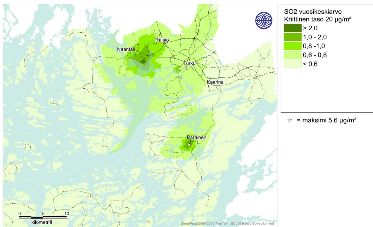
Kuva 16. Laivaliikenteen, energiantuotannon ja teollisuuden sekä alueellisen taustapitoisuuden (vuosikeskiarvona 0,4 \mu\text{g}/\text{m}^3 ) aiheuttama rikkidioksidin (SO 2 ) korkein vuosikeskiarvopitoisuus ( \mu\text{g}/\text{m}^3 ) Turun seudulla vuonna 2018.
