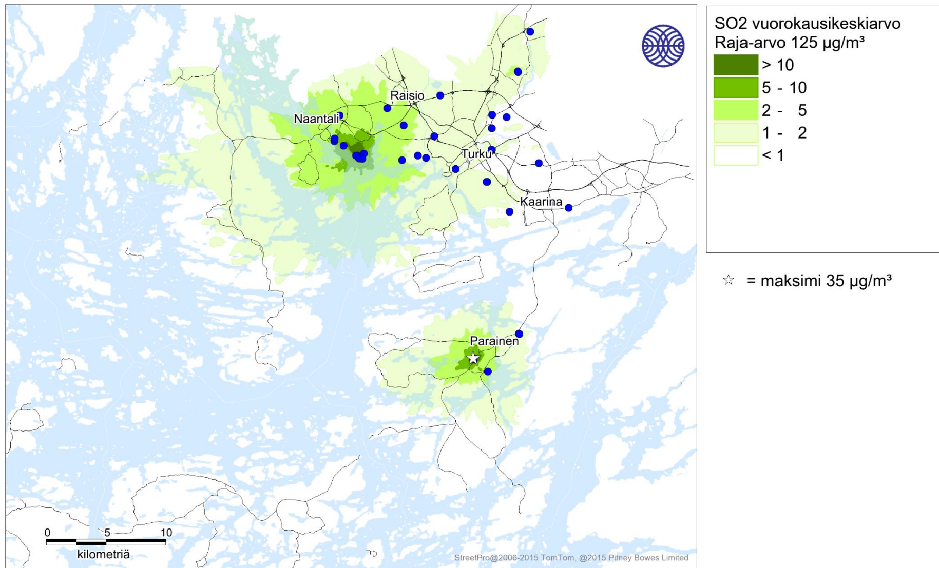
Kuva 53. Energiantuotannon ja teollisuuden päästöjen aiheuttama rikkidioksidin korkein vuorokausiraja-arvoon verrannollinen pitoisuus (µg/m 3 ) tarkastelujaksolla 2016-2018.
