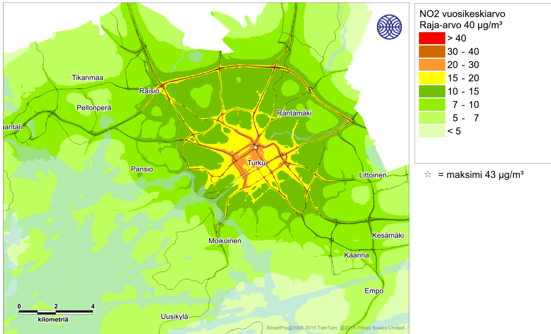
Kuva 2. Kaikkien päästölähteiden ja taustapitoisuuden yhdessä aiheuttama typidioksidin korkein vuosikeskiarvopitoisuus (µg/m³) tarkastelujaksolla 2016-2018.
