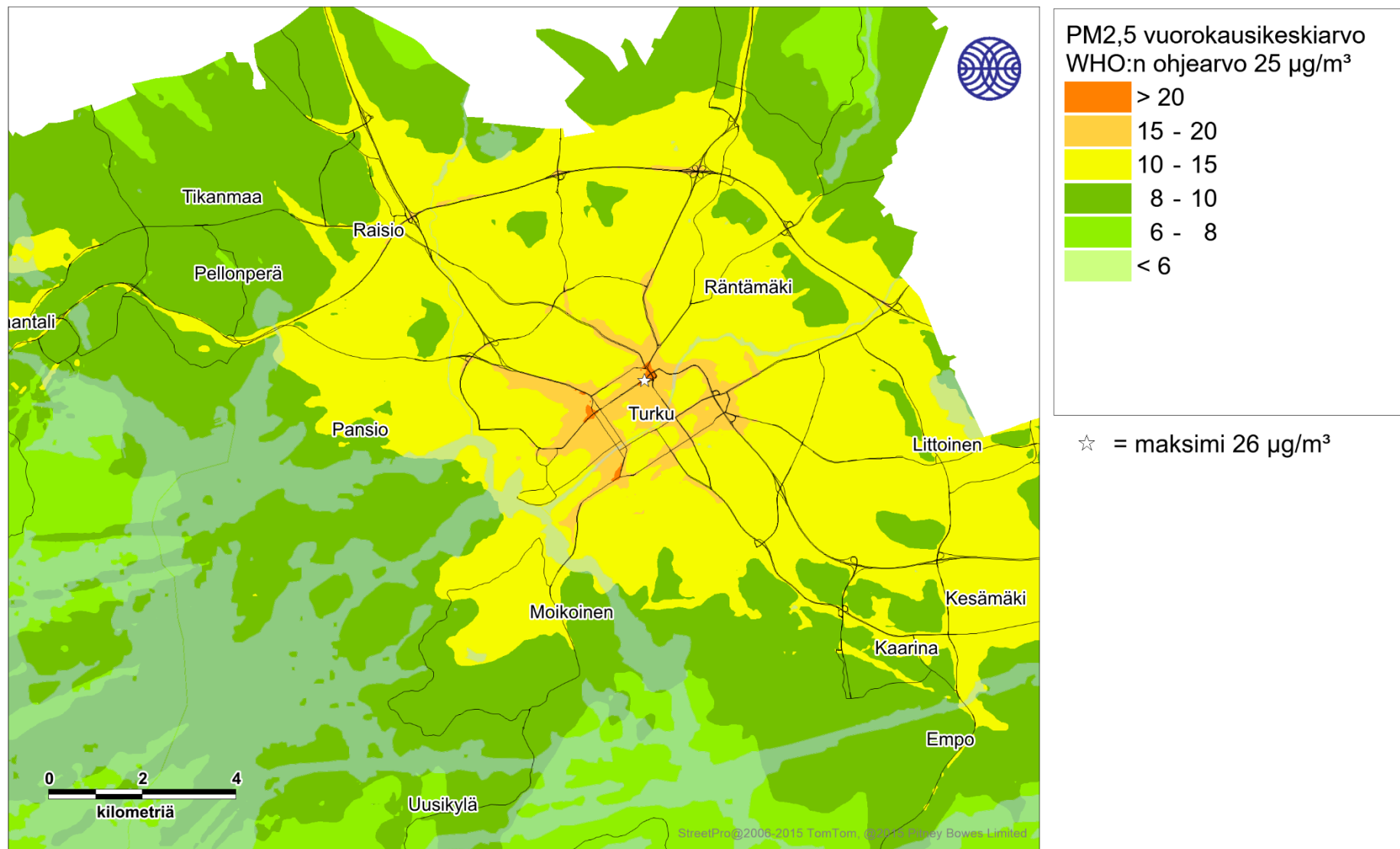
Kuva 22. Kaikkien päästölähteiden ja taustapitoisuuden aiheuttama pienhiukkasten korkein WHO:n vuorokausiohjearvoon verrannollinen pitoisuus (µg/m³) tarkastelujaksolla 2016-2018.
