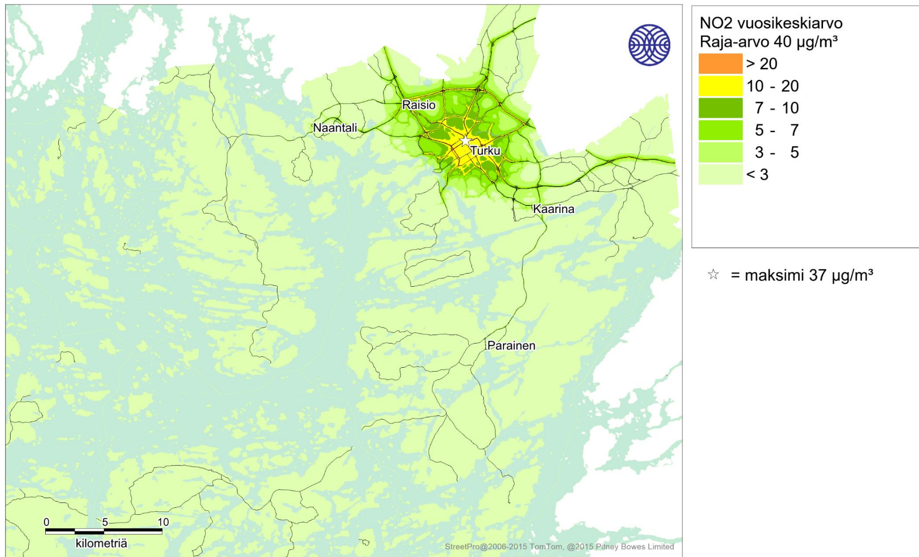
Kuva 5. Autoliikenteen päästöjen aiheuttama typidioksidin korkein vuosikeskiarvopitoisuus (µg/m³) tarkastelujaksolla 2016-2018.
