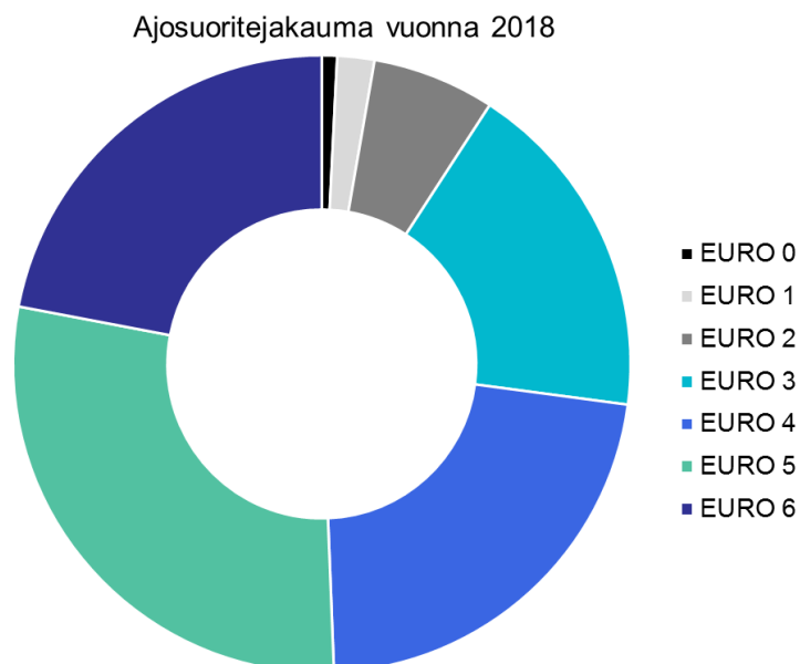
Kuva 43. ALISA-autokantamallin kaikkien ajoneuvojen EURO-päästöluokittaiset suoritejakaumat Suomessa vuonna 2018 (VTT, 2019).
