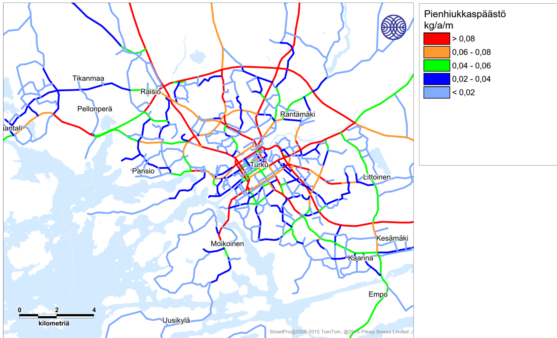
Kuva 64. Liikenteen pienhiukkaspäästöt (kg/a/m) vuonna 2018.
