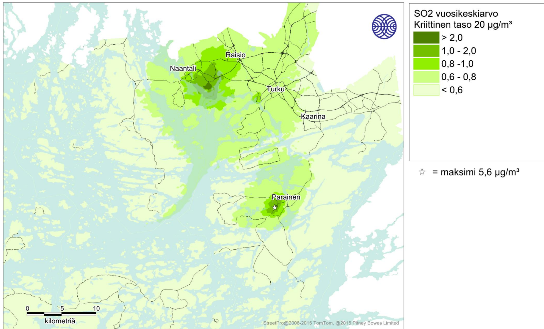
Kuva 47. Kaikkien päästölähteiden yhdessä aiheuttama rikkidioksidin korkein vuosikeskiarvopitoisuus (µg/m 3 ) tarkastelujaksolla 2016-2018.
