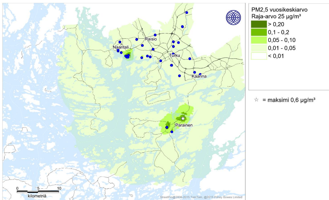
Kuva 10. Energiantuotannon ja teollisuuden päästöjen yksinään aiheuttama pienhiukkasten korkein vuosikeskiarvopitoisuus (µg/m 3 ) Turun seudulla vuonna 2018 ilman alueellista taustapitoisuutta. Siniset pisteet kuvaavat tarkastelussa mukana olleita energiantuotanto- tai teollisuuslaitoksia.
