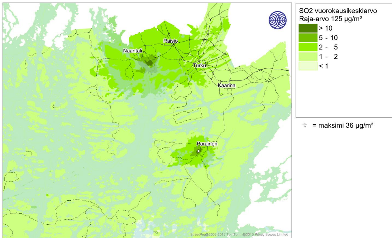
Kuva 17. Laivaliikenteen, energiantuotannon ja teollisuuden sekä alueellisen taustapitoisuuden (vuosikeskiarvona 0,4 µg/m 3 ) aiheuttama rikkidioksidin vuorokausiraja-arvoon verrannollinen pitoisuus (µg/m 3 ) Turun seudulla vuonna 2018.
