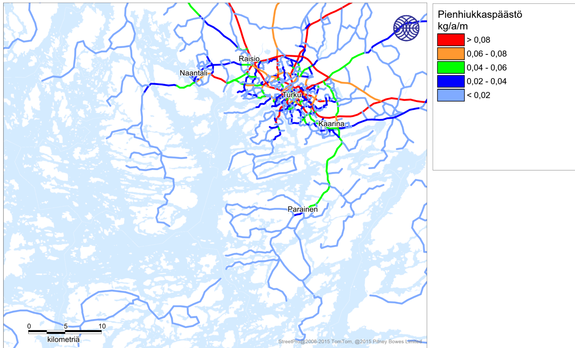
Kuva 63. Liikenteen pienhiukkaspäästöt (kg/a/m) vuonna 2018.
