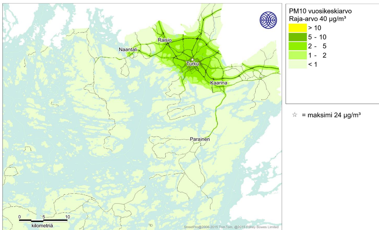
Kuva 15. Autoliikenteen päästöjen aiheuttama hengitettävien hiukkasten korkein vuosikeskiarvopitoisuus (µg/m³) Turun seudulla vuonna 2018 ilman alueellista taustapitoisuutta.
