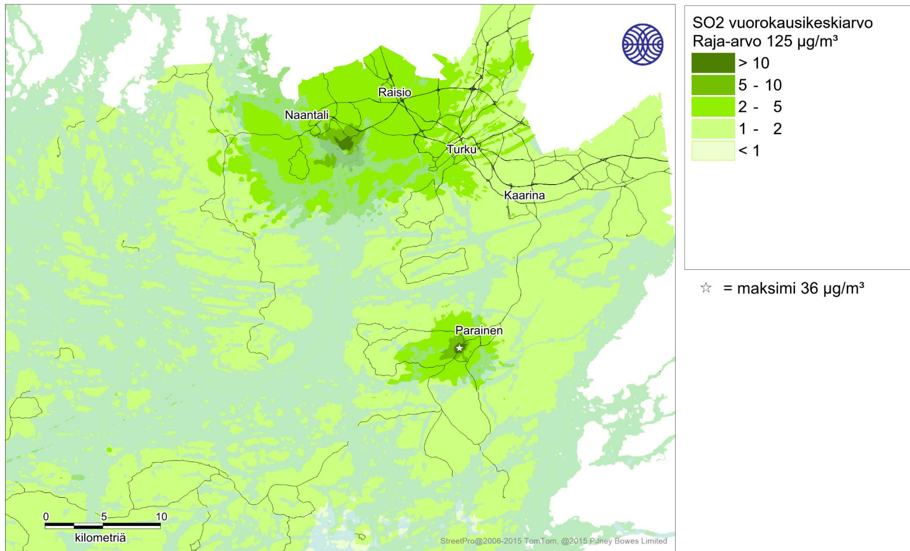
Kuva 49. Kaikkien päästölähteiden yhdessä aiheuttama rikkidioksidin korkein vuorokausiraja-arvoon verrannollinen pitoisuus (µg/m 3 ) tarkastelujaksolla 2016-2018.
