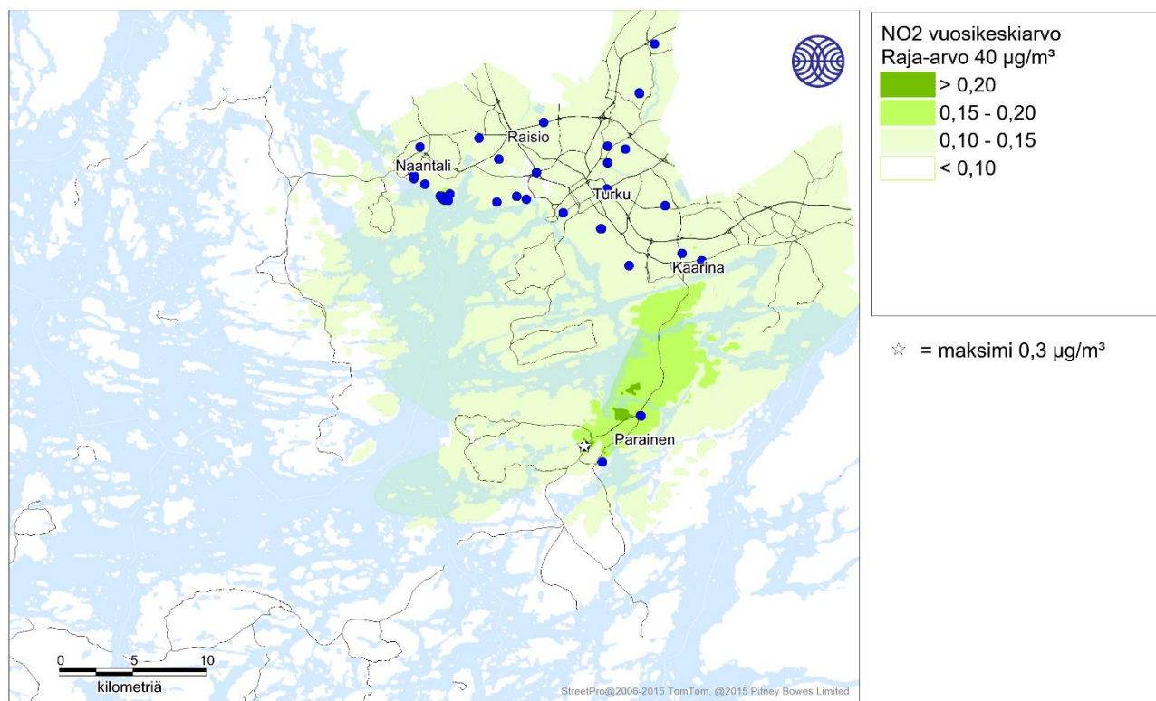
Kuva 5. Energiantuotannon ja teollisuuden päästöjen yksinään aiheuttama typpidioksidin korkein vuosikeskiarvopitoisuus (µg/m³) Turun seudulla vuonna 2018 ilman alueellista taustapitoisuutta. Siniset pisteet kuvaavat mallinnuksessa mukana olleita energiantuotanto- tai teollisuuslaitoksia.
