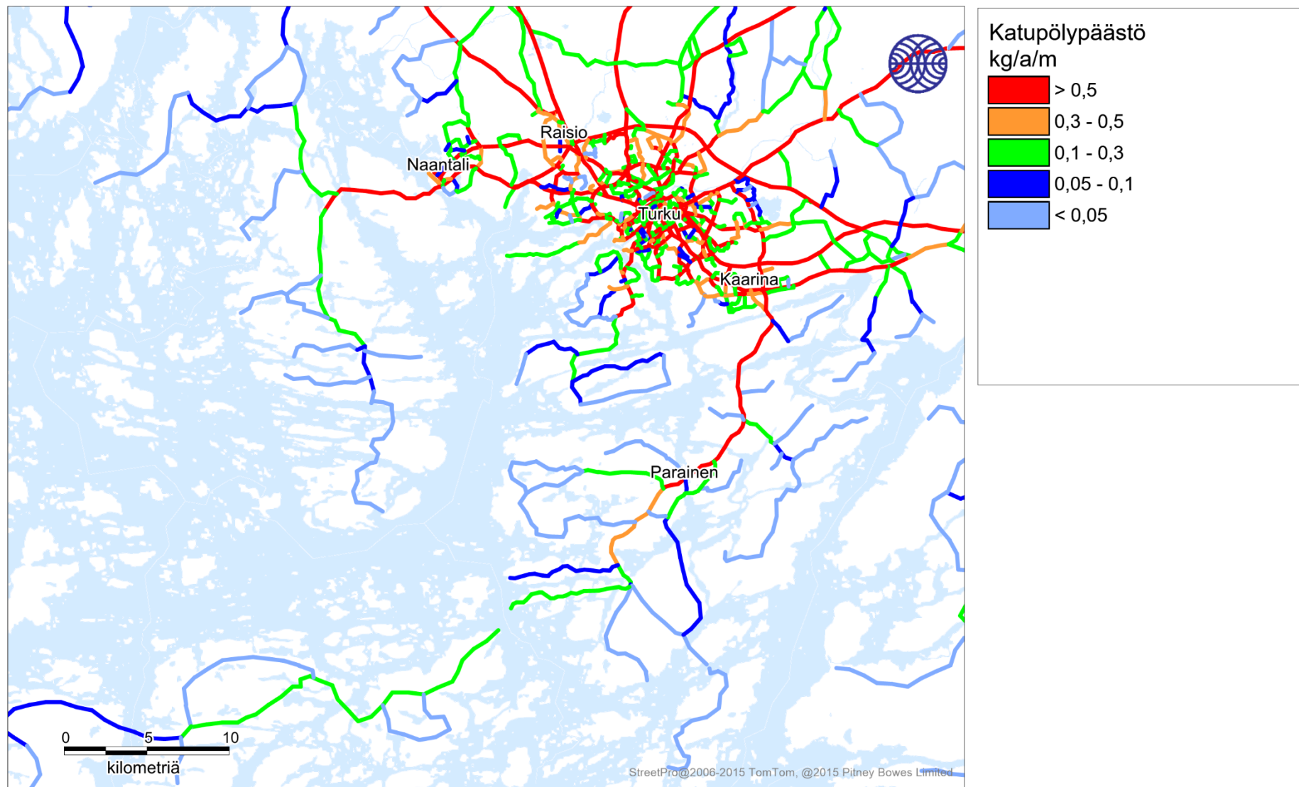
Kuva 65. Liikenteen katupölypäästöt eli PM10-suspensiopäästöt (kg/a/m) vuonna 2018.
