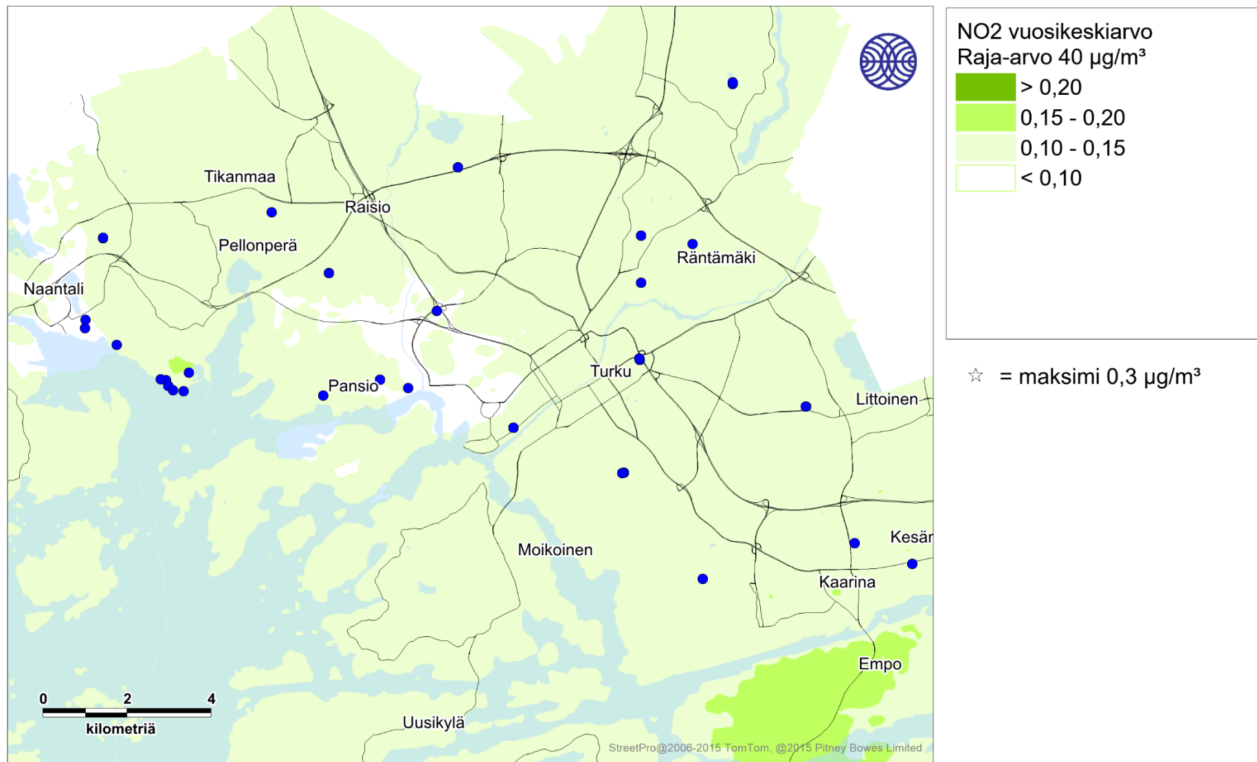
Kuva 10. Energiantuotannon ja teollisuuden päästöjen aiheuttama typpidioksidin korkein vuosikeskiarvopitoisuus (µg/m³) tarkastelujaksolla 2016-2018.
