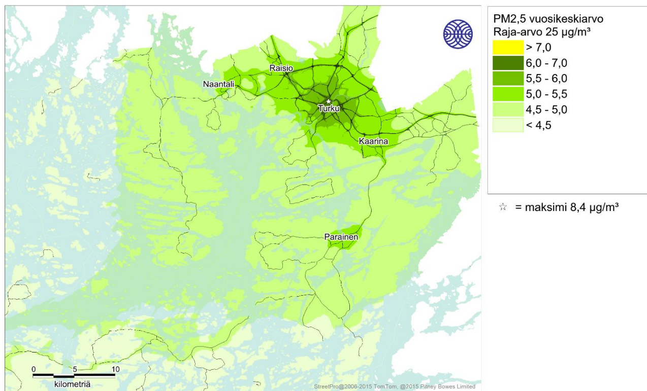
Kuva 7. Autoliikenteen, energiantuotannon, teollisuuden, laivaliikenteen ja puunpolton päästöjen sekä alueellisen taustapitoisuuden (vuosikeskiarvona 4,4 µg/m³) yhdessä aiheuttama pienhiukkasten (PM 2,5 ) korkein vuosikeskiarvopitoisuus (µg/m³) Turun seudulla vuonna 2018.
