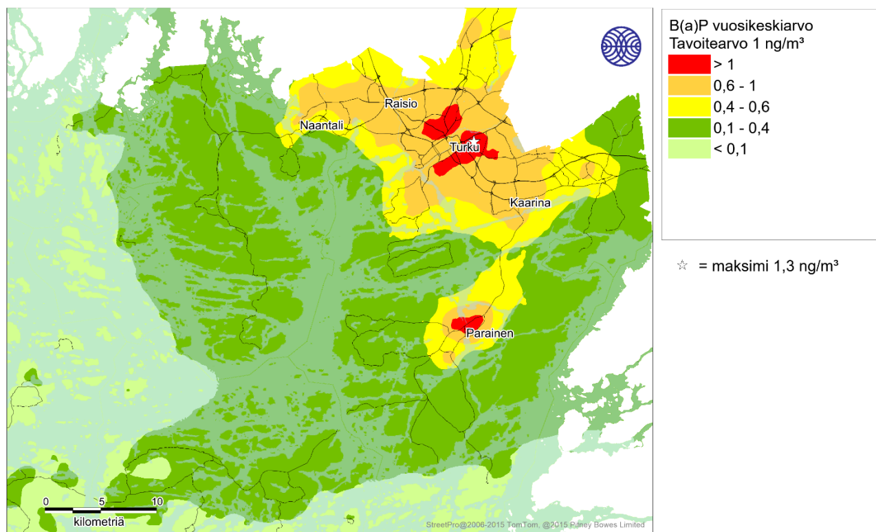
Kuva 20. Puun polton päästöjen aiheuttama bentso(a)pyreenin korkein vuosikeskiarvopitoisuus (ng/m 3 ) Turun seudulla vuonna 2018 ilman alueellista taustapitoisuutta.
