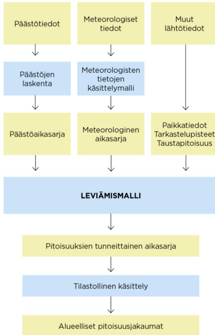
Kuva 50. Kaaviokuva Ilmatieteen laitoksella kehitettyjen leviämismallien, piste- ja pintapäästölähteiden leviämismallin UDM-FMI ja viivalähdemallin CAR-FMI toiminnasta.
