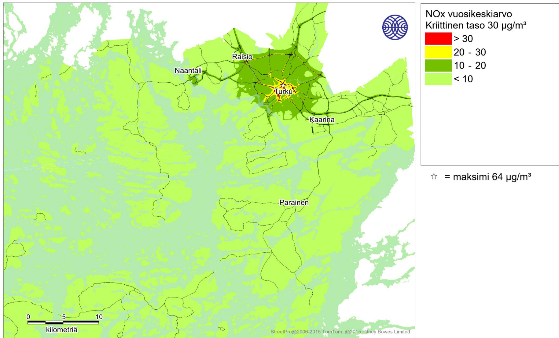
Kuva 17. Kaikkien päästölähteiden ja taustapitoisuuden yhdessä aiheuttama typenoksidien korkein vuosikeskiarvopitoisuus (µg/m³) tarkastelujaksolla 2016-2018.
