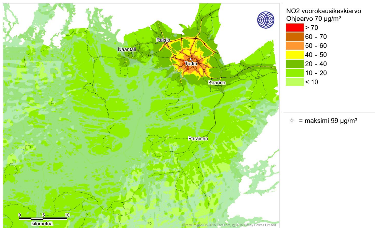
Kuva 2. Autoliikenteen, energiantuotannon, teollisuuden ja laivaliikenteen päästöjen sekä alueellisen taustapitoisuuden (vuosikeskiarvona 3,7 µg/m 3 ) yhdessä aiheuttama typpidioksidin vuorokausiohjearvoon verrannollinen pitoisuus (µg/m 3 ) Turun seudulla vuonna 2018.
