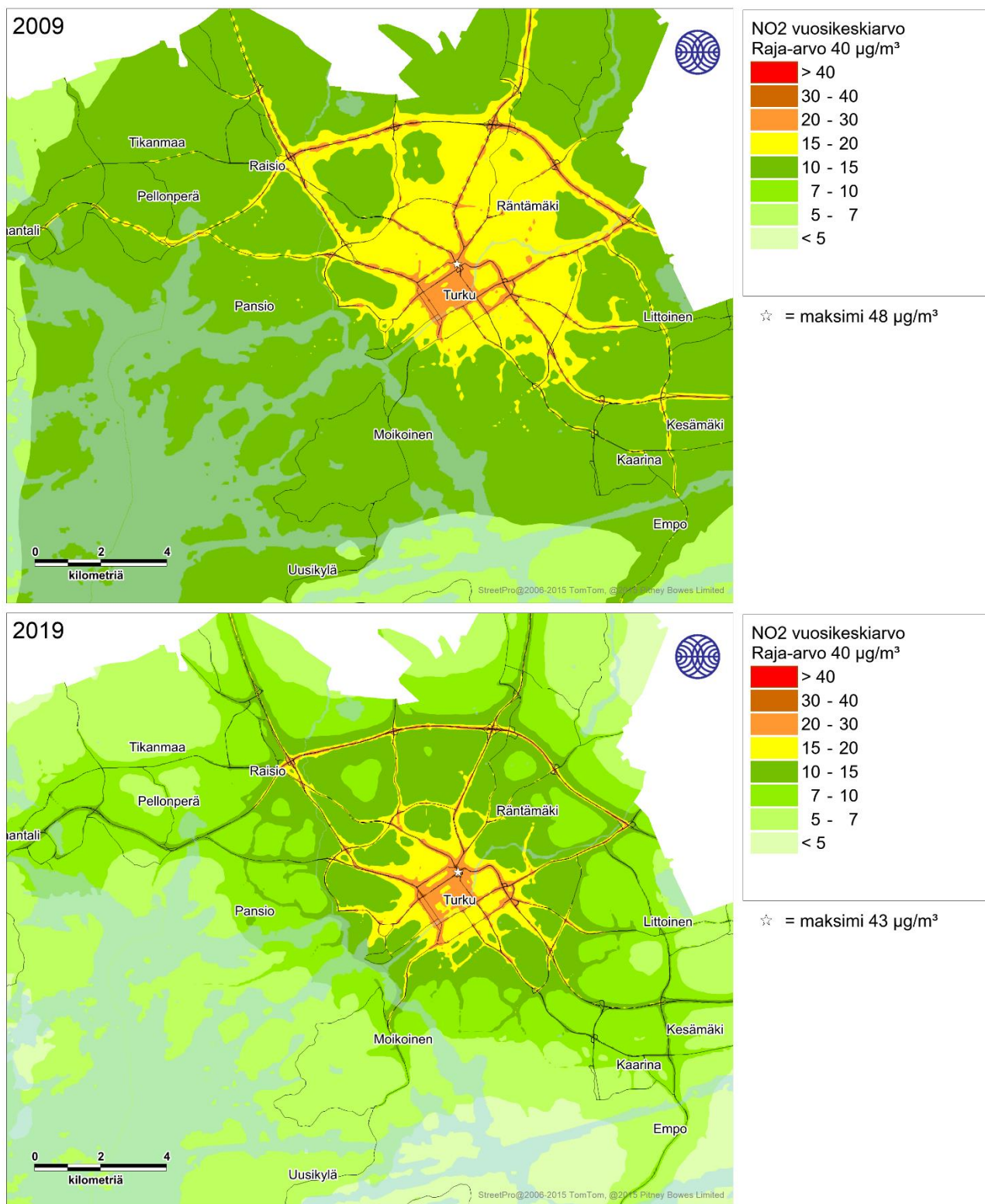
Kuva 35. Vuonna 2009 ja 2019 mallinnettu typpidioksidin (NO 2 ) korkein vuosikeskiarvopitoisuus (µg/m³) Turun seudulla.
