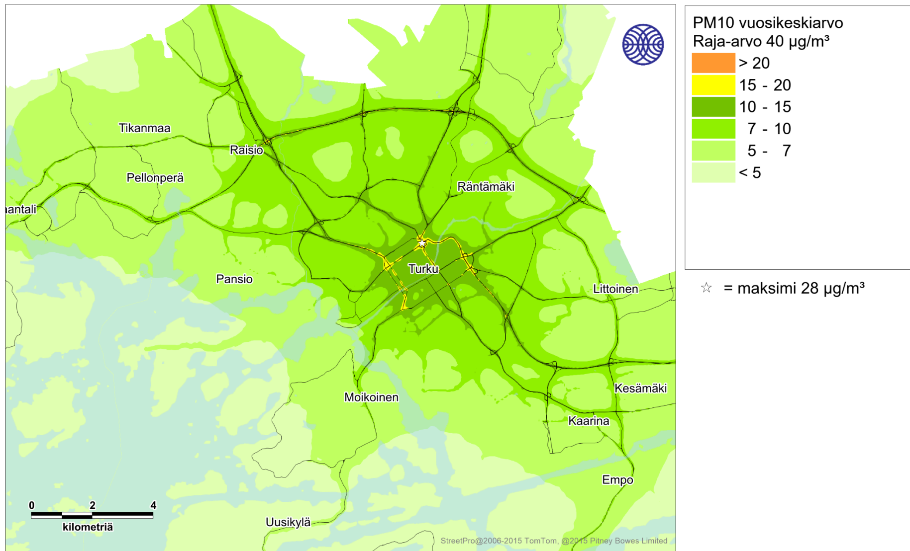
Kuva 40. Kaikkien päästölähteiden ja taustapitoisuuden yhdessä aiheuttama hengitettävien hiukkasten korkein vuosikeskiarvopitoisuus (µg/m³) tarkastelujaksolla 2016-2018.
