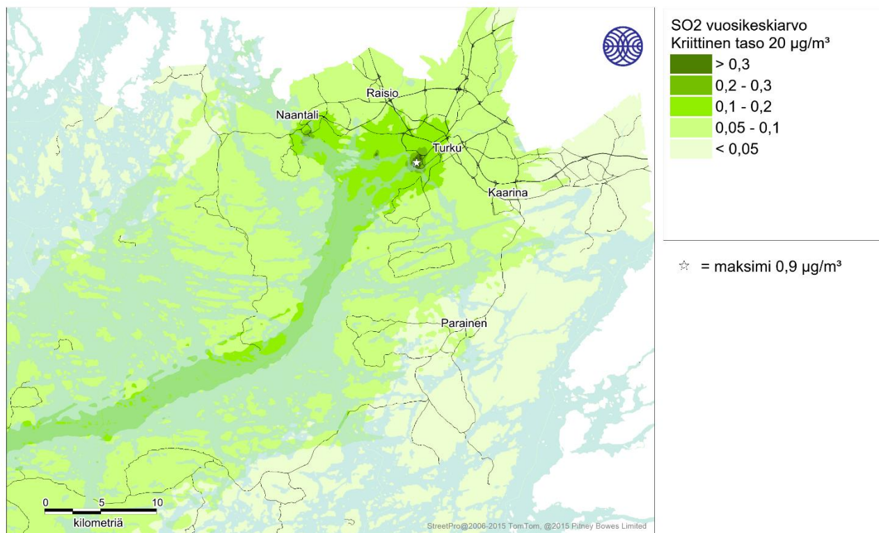
Kuva 19. Laivaliikenteen päästöjen aiheuttama rikkidioksidin korkein vuosikeskiarvopitoisuus (µg/m 3 ) Turun seudulla vuonna 2018 ilman alueellista taustapitoisuutta.
