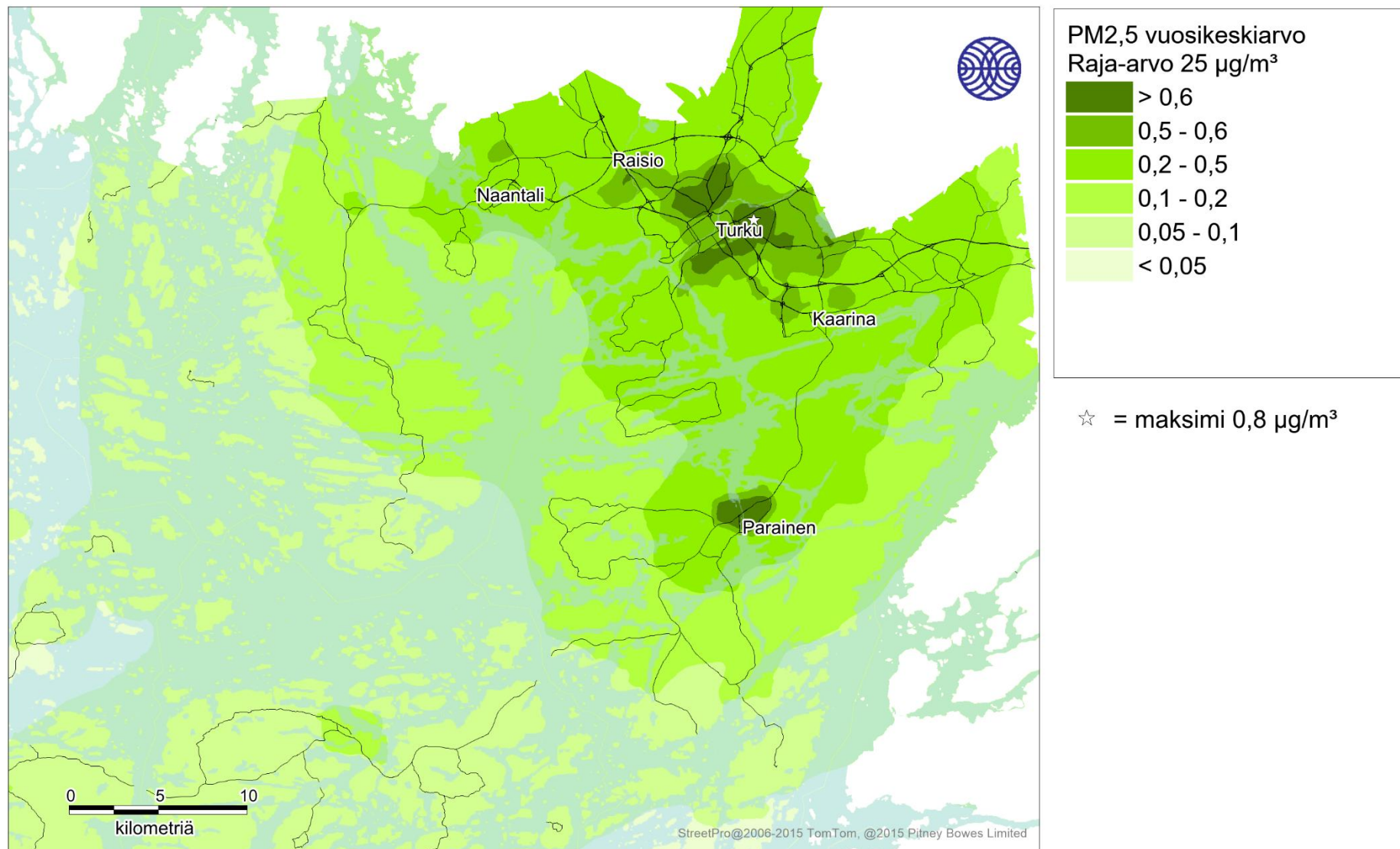
Kuva 35. Puunpolton päästöjen aiheuttama pienhiukkasten korkein vuosikeskiarvopitoisuus (µg/m³) tarkastelujaksolla 2016-2018.
