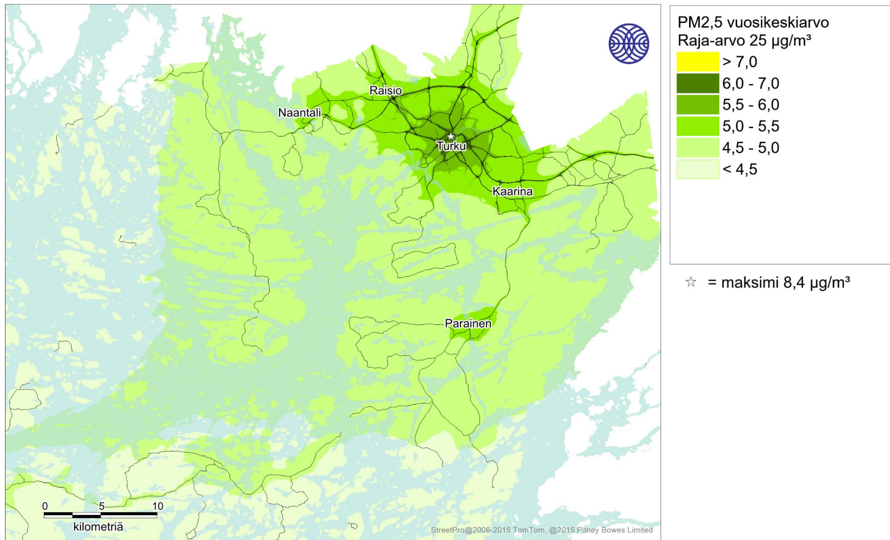
Kuva 19. Kaikkien päästölähteiden ja taustapitoisuuden yhdessä aiheuttama pienhiukkasten korkein vuosikeskiarvopitoisuus (µg/m 3 ) tarkastelujaksolla 2016-2018.
