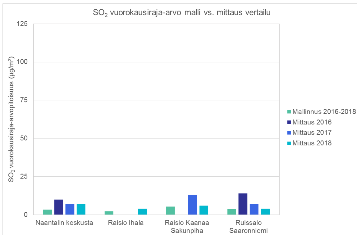
Kuva 29. Mallinnettujen ja mitattujen rikkidioksidin vuorokausiraja-arvoon ( 125 \mu\text{g}/\text{m}^3 ) verrannollisten pitoisuuksien vertailu Turun seudun ilmanlaadun mittausasemilla.
