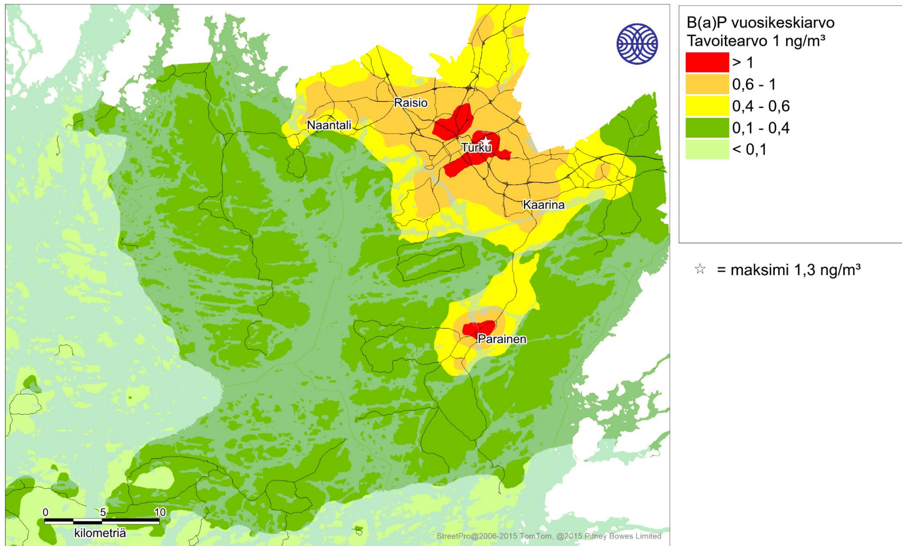
Kuva 59. Puunpolton päästöjen aiheuttama bentso(a)pyreenin korkein vuosikeskiarvopitoisuus (ng/m 3 ) tarkastelujaksolla 2016-2018.
