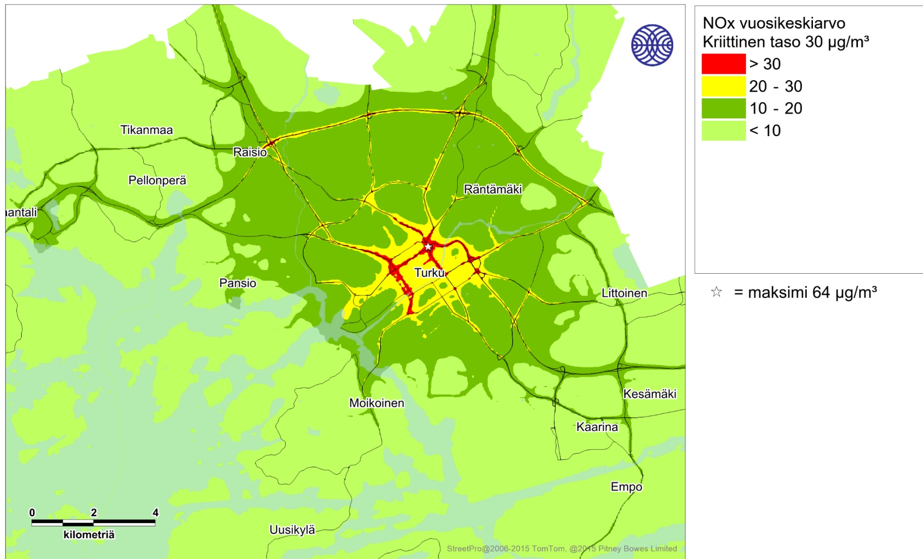
Kuva 18. Kaikkien päästölähteiden ja taustapitoisuuden yhdessä aiheuttama typenoksidien korkein vuosikeskiarvopitoisuus (µg/m³) tarkastelujaksolla 2016-2018.
