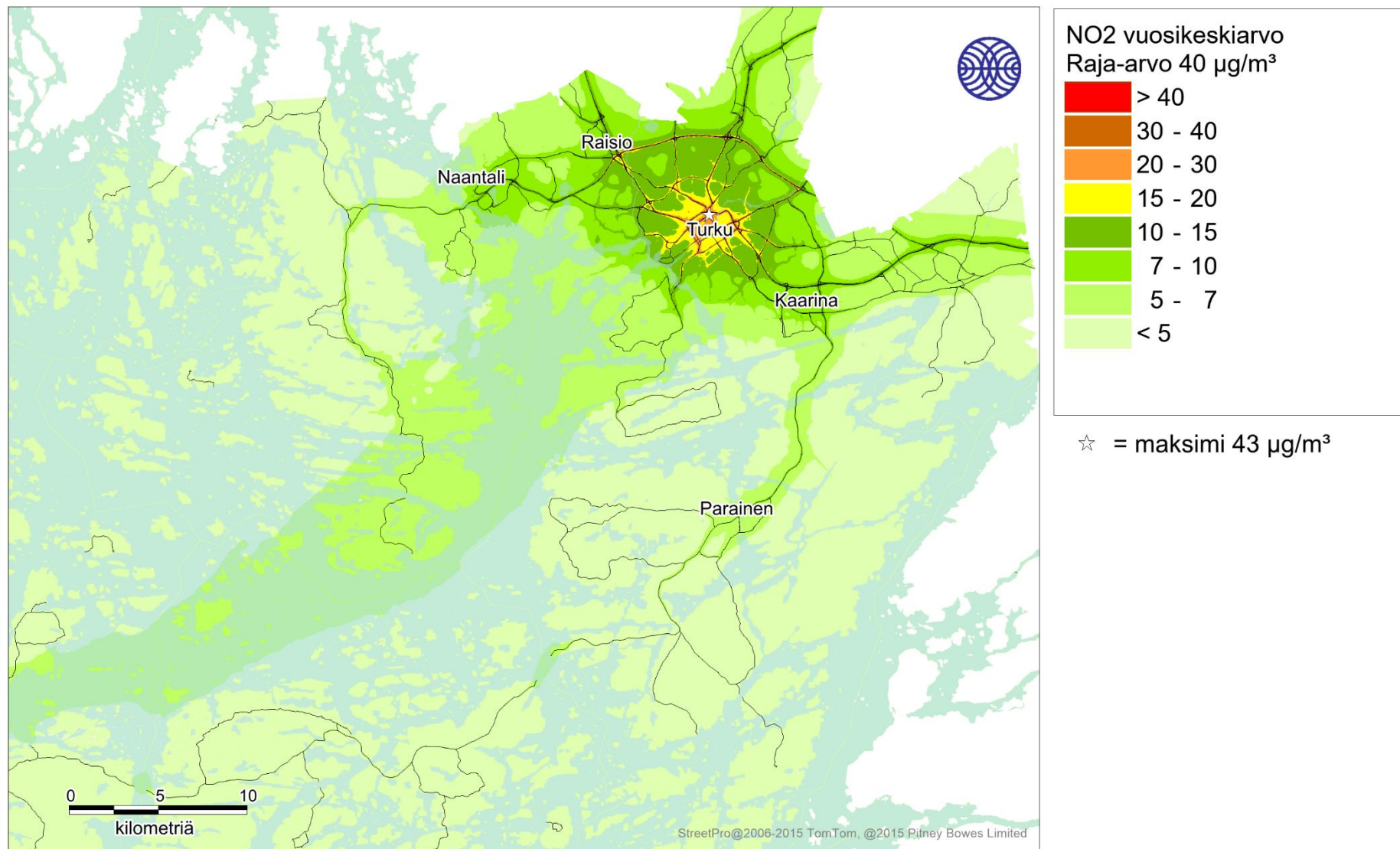
Kuva 1. Kaikkien päästölähteiden ja taustapitoisuuden yhdessä aiheuttama typpidioksidin korkein vuosikeskiarvopitoisuus (µg/m³) tarkastelujaksolla 2016-2018.
