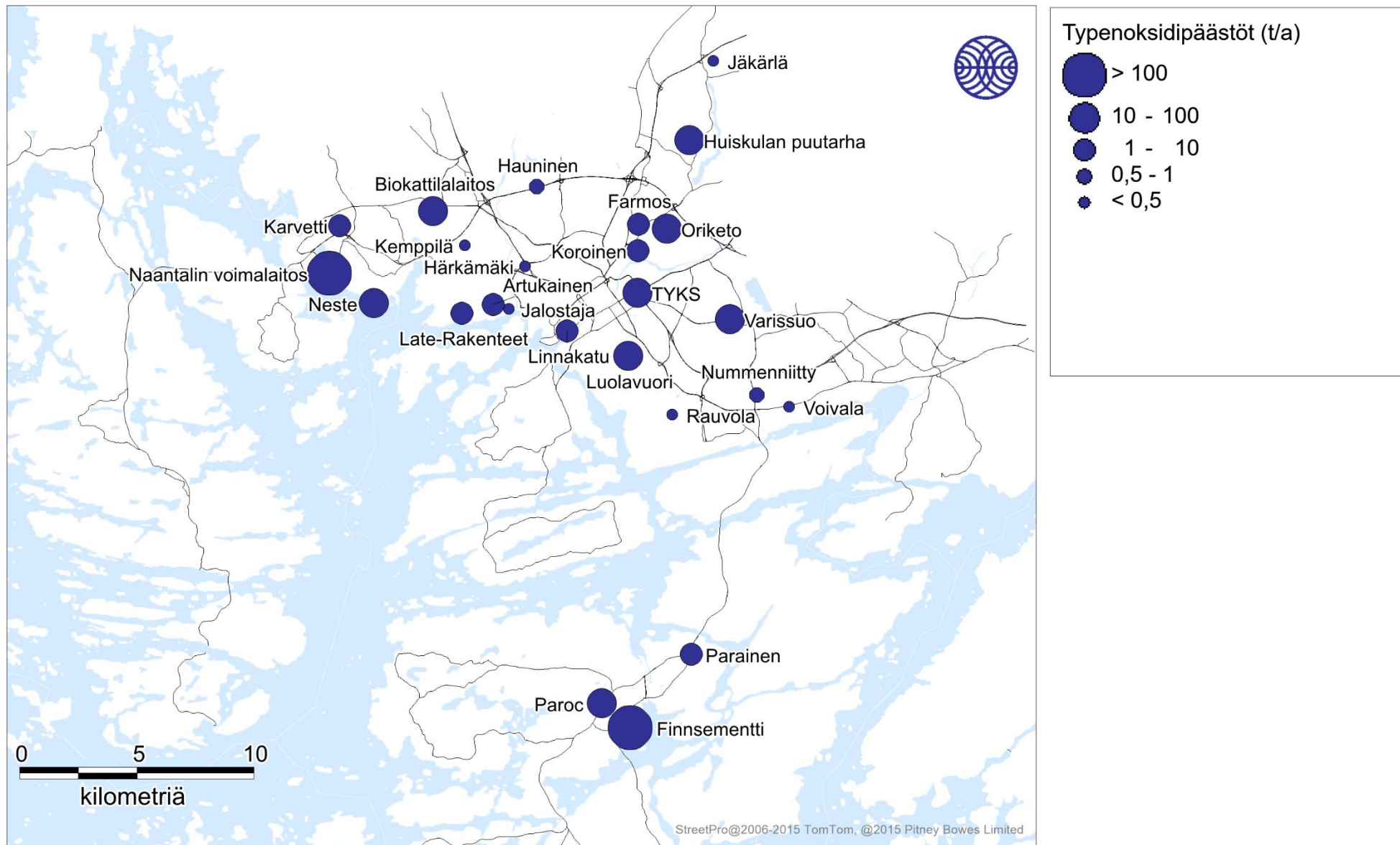
Kuva 67. Energiantuotannon ja teollisuuden NOx-päästöt (t/a) vuonna 2018.
