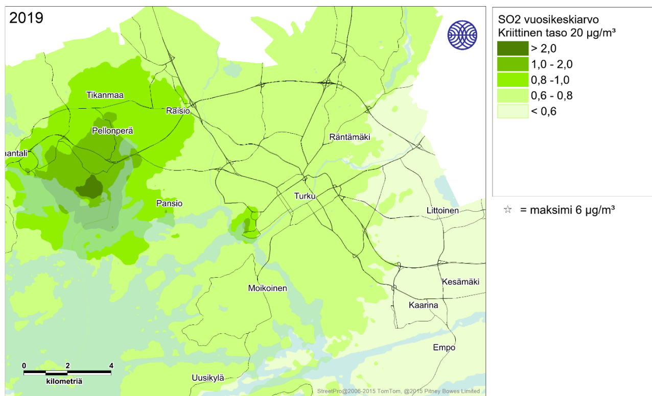
Kuva 37. Vuonna 2009 ja 2019 mallinnettu rikkidioksidin (SO 2 ) korkein vuosikeskiarvopitoisuus (µg/m³) Turun seudulla.
