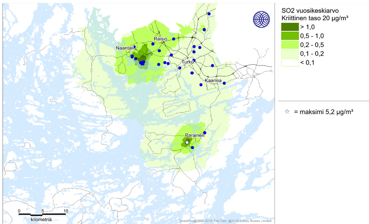
Kuva 18. Energiantuotannon ja teollisuuden päästöjen aiheuttama rikkidioksidin korkein vuosikeskiarvopitoisuus (µg/m³) Turun seudulla vuonna 2018 ilman alueellista taustapitoisuutta. Siniset pisteet kuvaavat mallinnuksessa mukana olleita energiantuotanto- tai teollisuuslaitoksia.
