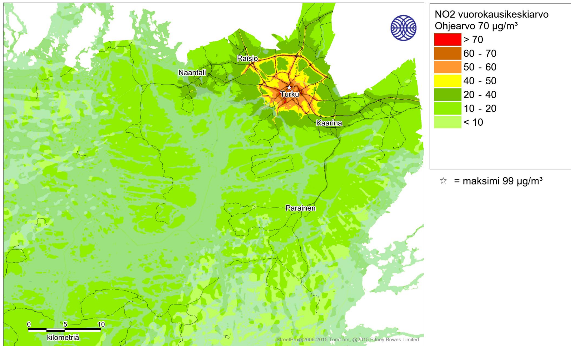
Kuva 3. Kaikkien päästölähteiden ja taustapitoisuuden yhdessä aiheuttama typpidioksidin korkein vuorokausiohjeeseen verrannollinen pitoisuus ( \mu\text{g}/\text{m}^3 ) tarkastelujaksolla 2016-2018.
