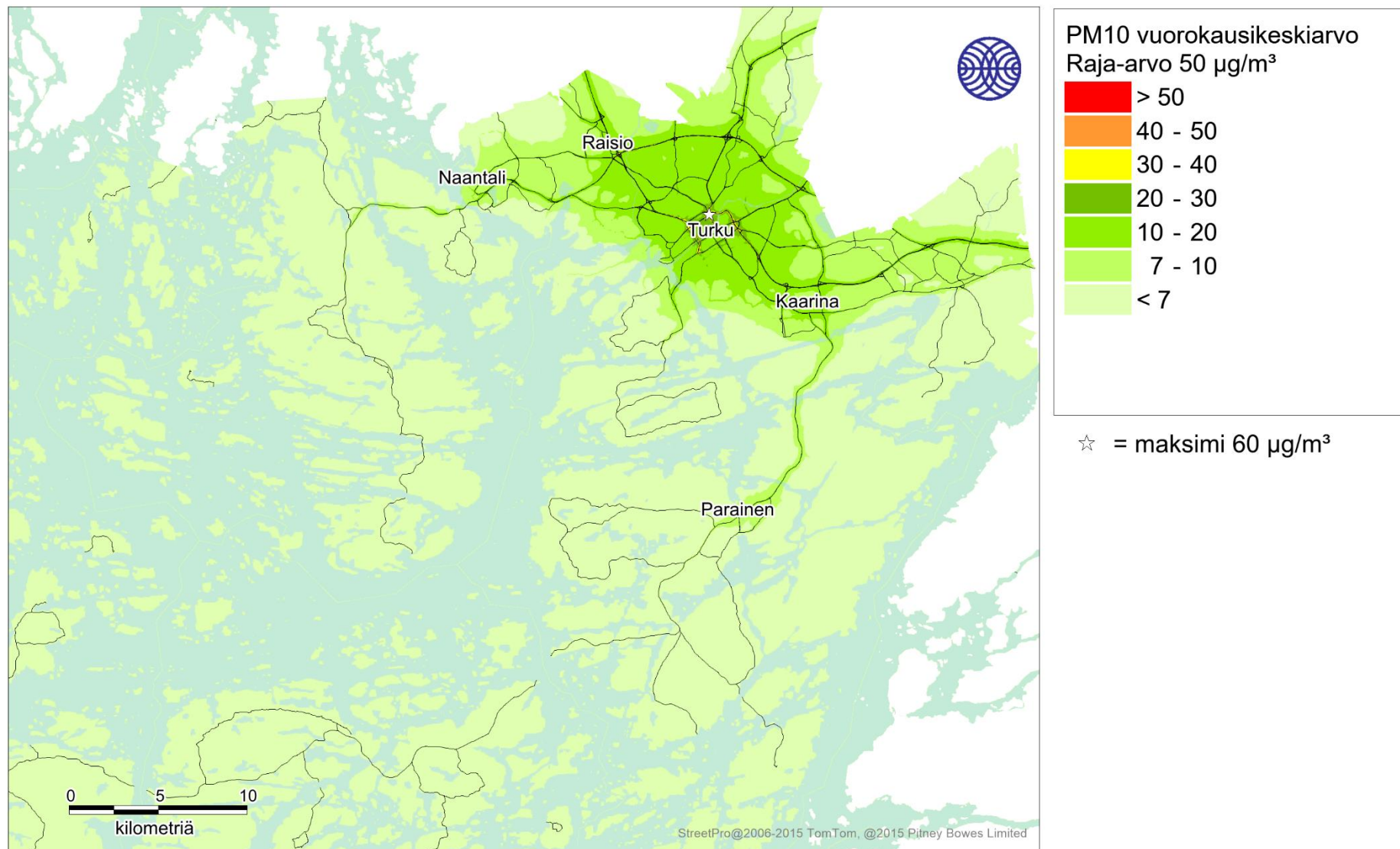
Kuva 41. Kaikkien päästölähteiden ja taustapitoisuuden aiheuttama hengitettävien hiukkasten korkein vuorokausiraja-arvoon verrannollinen pitoisuus (µg/m³) tarkastelujaksolla 2016-2018.
