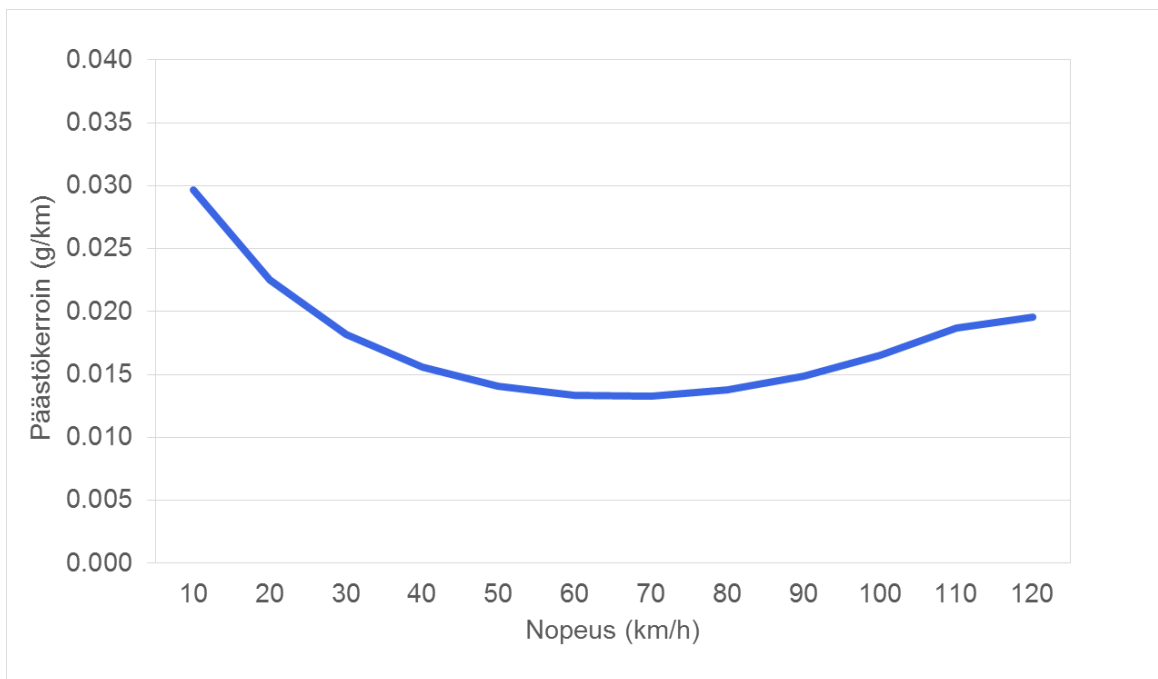
Kuva 45. Mallilaskelmissa käytettävät ajoneuvojen keskimääräiset nopeusriippuvat pienhiukkasten ( \text{PM}_{2.5} ) päästökertoimet. Kertoimien pohjana ovat EEA:n päästökertoimet (EEA, 2018) painotettuna suoritteiden EURO-päästöluokkajakaumilla ja koko Suomen keskimääräisillä ajonsuoriteosuuksilla vuonna 2018 (VTT, 2019).
