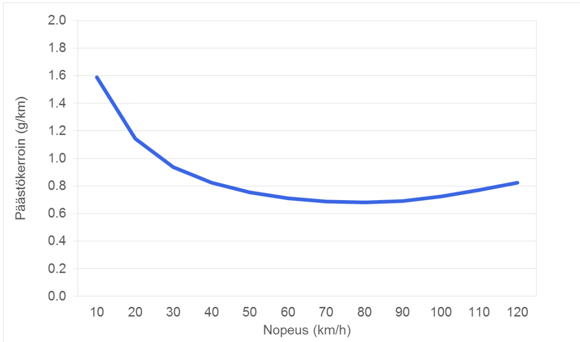
Kuva 44. Mallilaskelmissa käytettävät ajoneuvojen keskimääräiset nopeusriippuvat typenoksidien ( \text{NO}_x ) päästökertoimet. Kertoimien pohjana ovat EEA:n päästökertoimet (EEA, 2018) painotettuna suoritteiden EURO-päästöluokkajakaumilla ja koko Suomen keskimääräisillä ajosuoriteosuuksilla vuonna 2018 (VTT, 2019).
