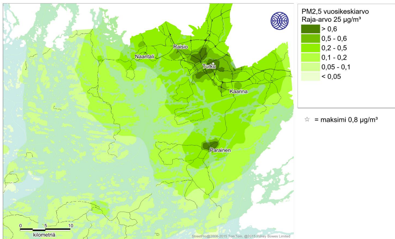
Kuva 12. Asuinrakennusten puunpolton päästöjen yksinään aiheuttama pienhiukkasten korkein vuosikeskiarvopitoisuus (µg/m³) Turun seudulla vuonna 2018 ilman alueellista taustapitoisuutta.
