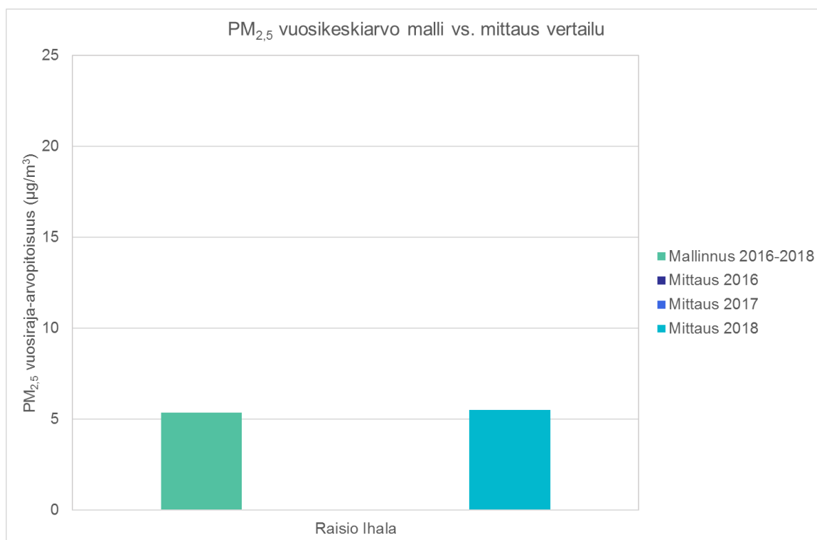
Kuva 24. Mallinnettujen ja mitattujen pienhiukkasten vuosiraja-arvoon ( 25 \mu\text{g}/\text{m}^3 ) verrannollisten pitoisuuksien vertailu Raision Ihalan ilmanlaadun mittausasemalla.
