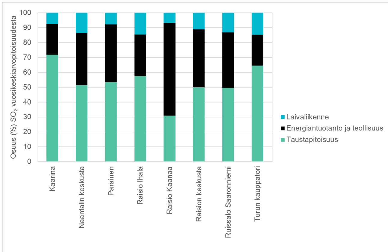
Kuva 34. Eri päästölähdesektoreiden osuus mallinnetuista rikkidioksidin vuosikeskiarvopitoisuuksista ilmanlaadun mittauspisteissä vuonna 2018.
