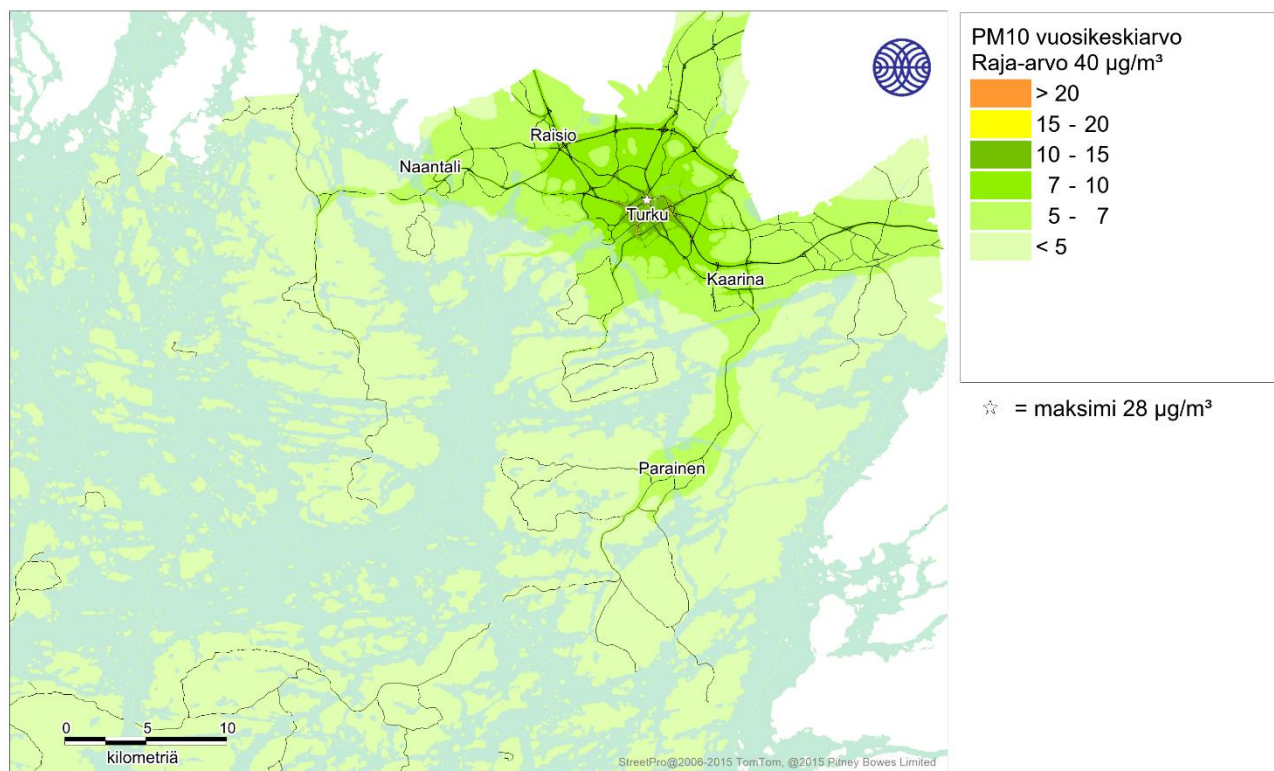
Kuva 13. Autoliikenteen, energiantuotannon, teollisuuden ja puun polton päästöjen sekä pienhiukkasten alueellisen taustapitoisuuden (vuosikeskiarvona 4,4 µg/m³) aiheuttama hengitettävien hiukkasten (PM 10 ) korkein vuosikeskiarvopitoisuus (µg/m³) Turun seudulla vuonna 2018.
