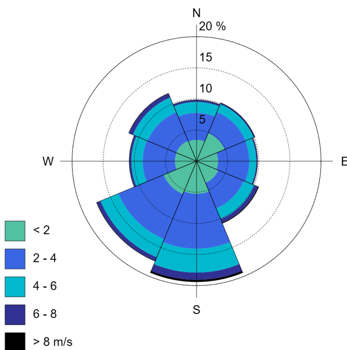
Kuva 49. Keskimääräinen tuulen suunta- ja nopeusjakauma Turun seudulla vuosina 2016–2018. Tuulitiedot kuvaavat olosuhteita 10 metrin korkeudella maan pinnasta.
