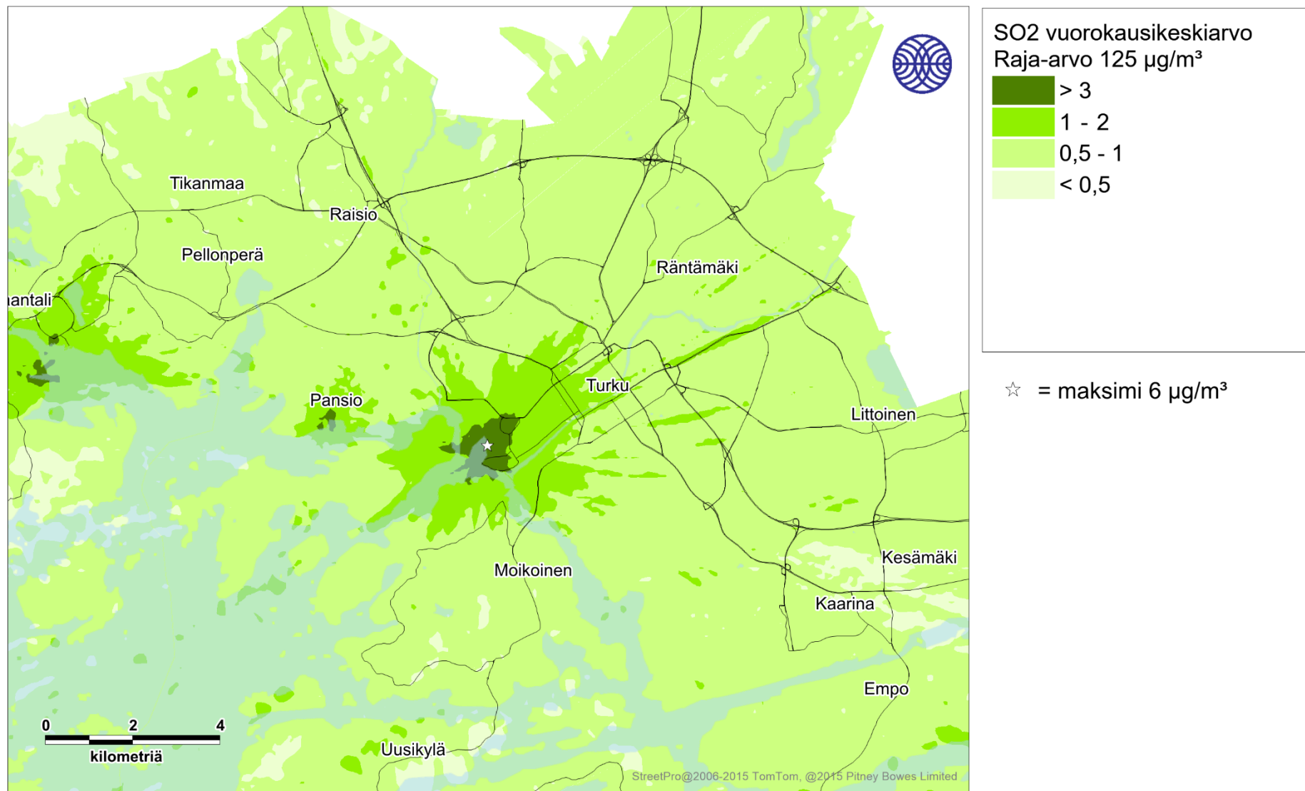
Kuva 58. Laivaliikenteen päästöjen aiheuttama rikkidioksidin korkein vuorokausiraja-arvoon verrannollinen pitoisuus (µg/m 3 ) tarkastelujaksolla 2016-2018.
