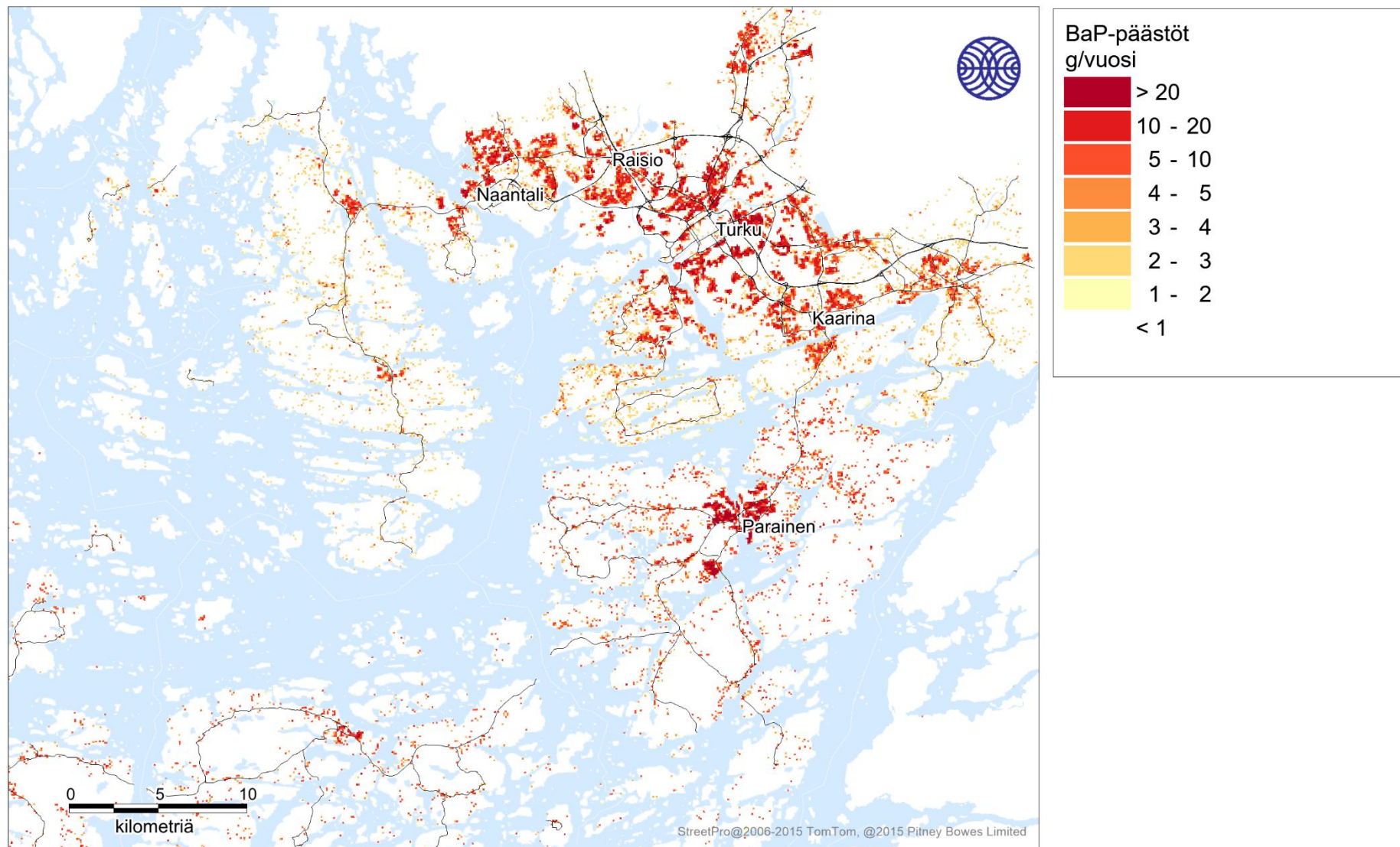
Kuva 75. Puunpolton bentso(a)pyreenipäästöt (g/a).
