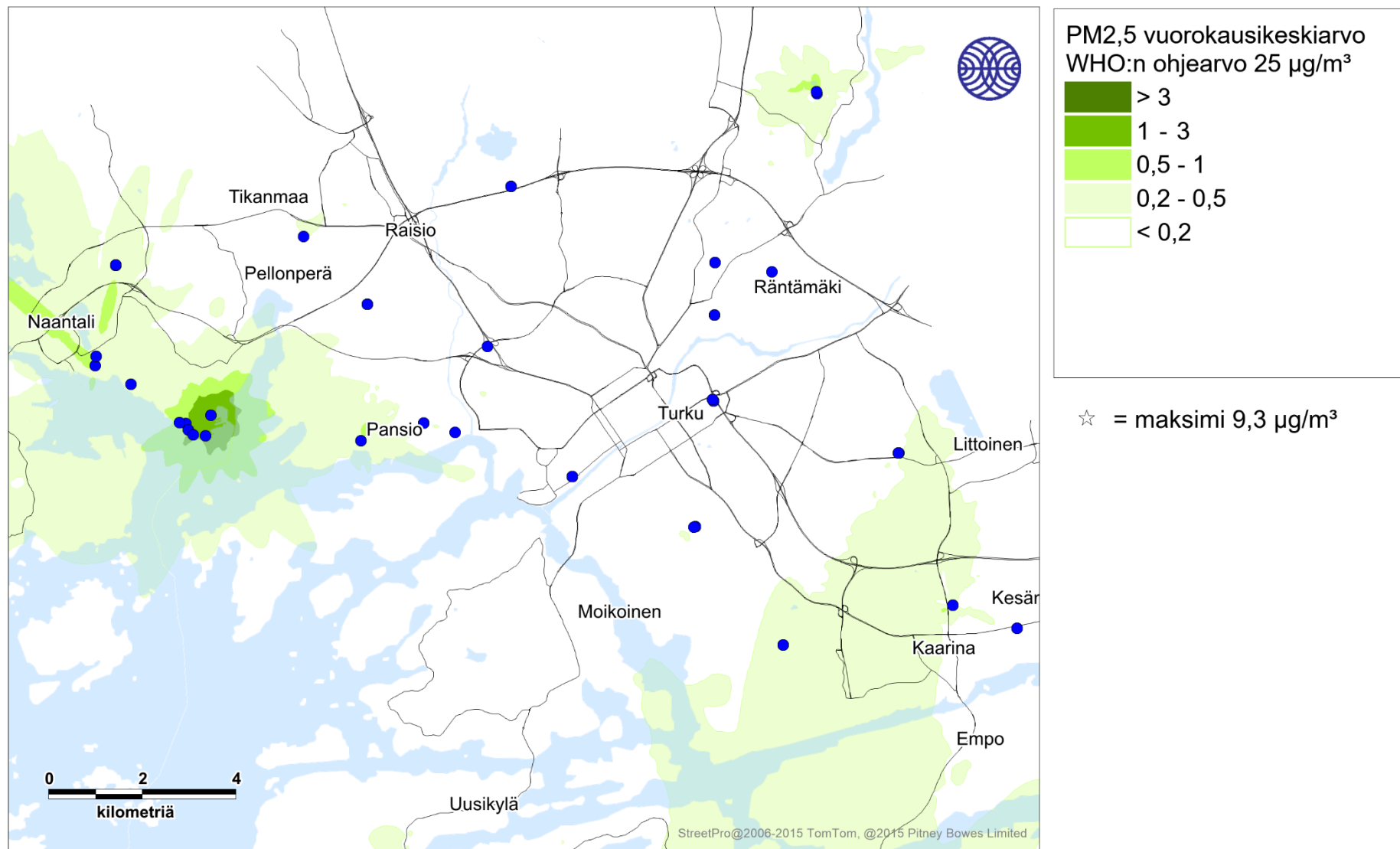
Kuva 30. Energiantuotannon ja teollisuuden päästöjen aiheuttama pienhiukkasten korkein WHO:n vuorokausiohjearvoon verrannollinen pitoisuus (µg/m³) tarkastelujaksolla 2016-2018.
