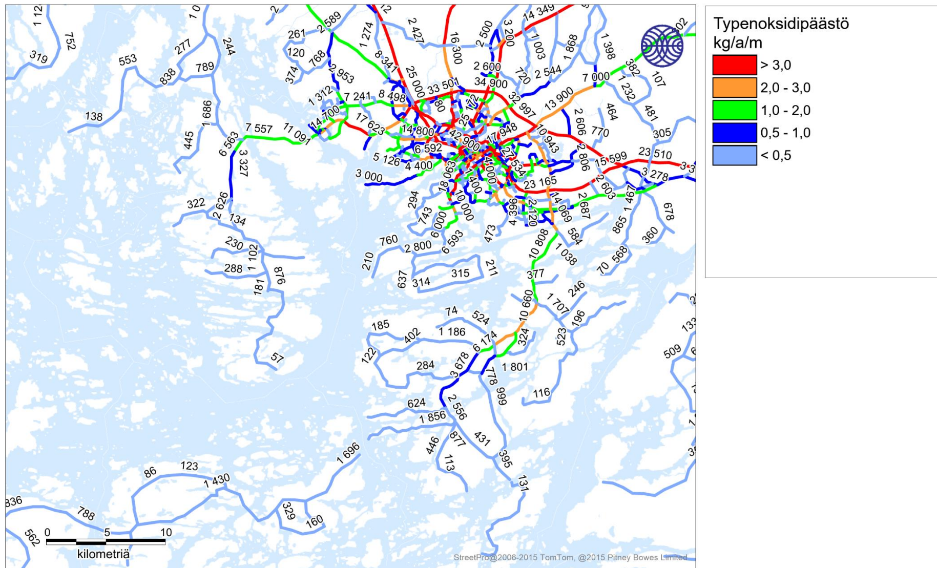
Kuva 61. Liikenteen NOx-päästöt (kg/a/m) ja keskimääräinen vuorokausiliikennemäärä (KVL/KAVL) vuonna 2018.
