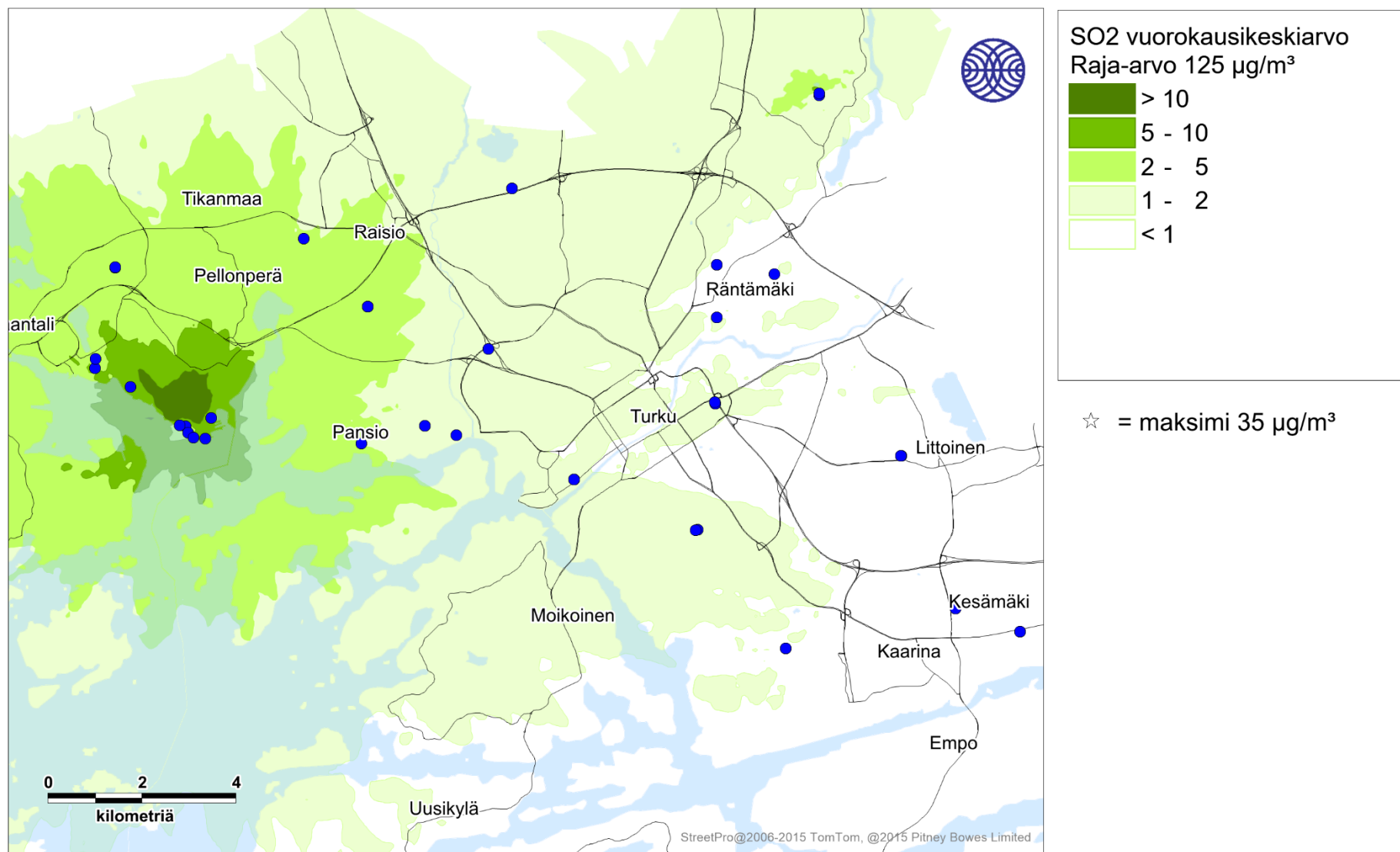
Kuva 54. Energiantuotannon ja teollisuuden päästöjen aiheuttama rikkidioksidin korkein vuorokausiraja-arvoon verrannollinen pitoisuus (µg/m 3 ) tarkastelujaksolla 2016-2018.
