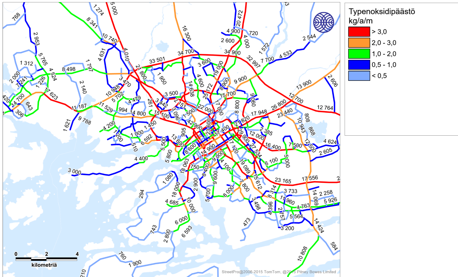
Kuva 62. Liikenteen NOx-päästöt (kg/a/m) ja keskimääräinen vuorokausiliikennemäärä (KVL/KAVL) vuonna 2018.
