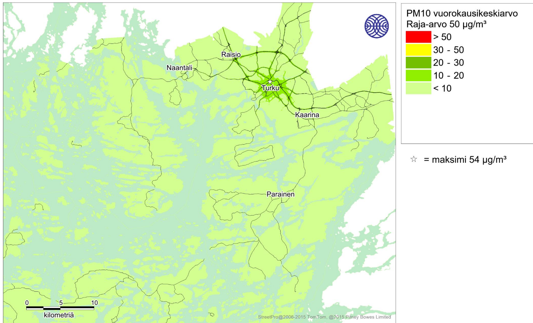
Kuva 45. Autoliikenteen päästöjen aiheuttama hengitettävien hiukkasten korkein vuorokausiraja-arvoon verrannollinen pitoisuus (µg/m³) tarkastelujaksolla 2016-2018.
