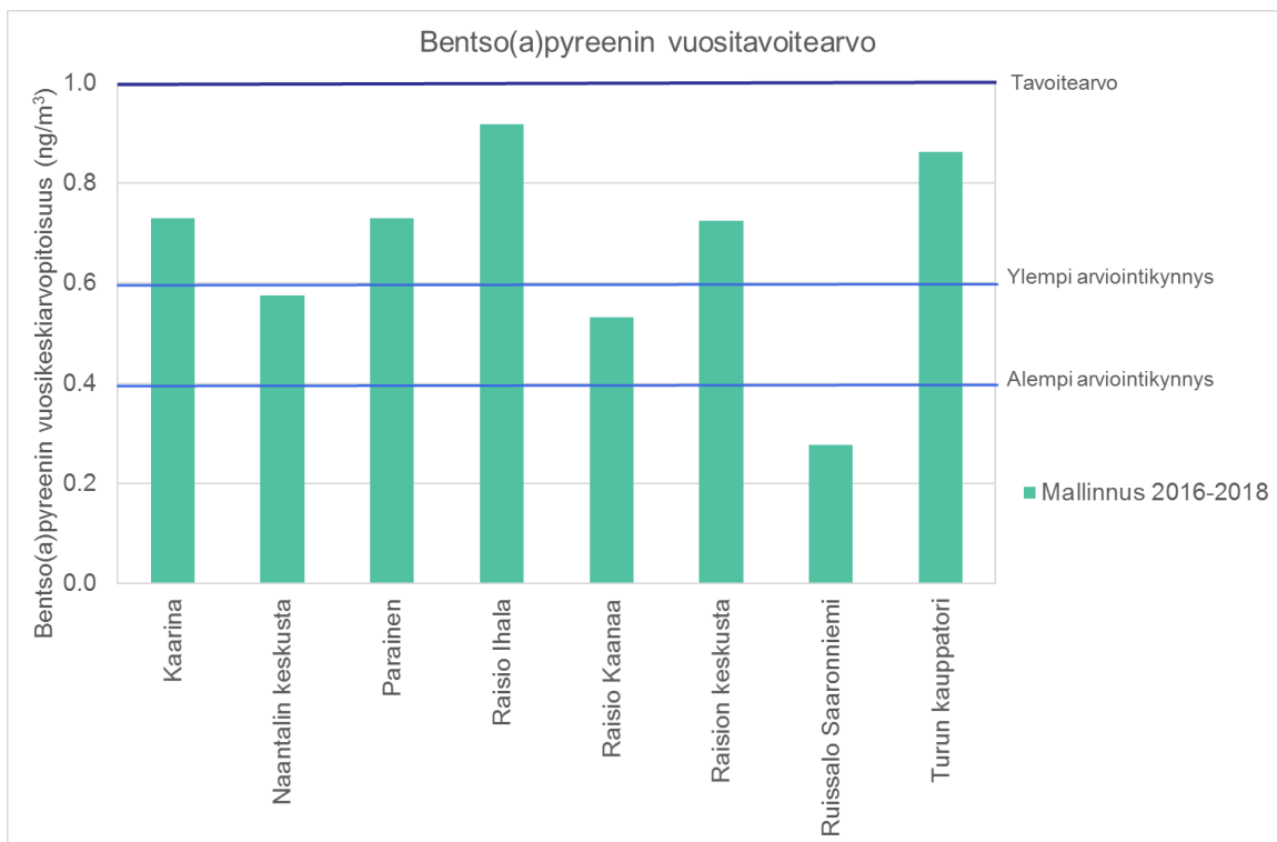
Kuva 30. Mallinnetut bentso(a)pyreenin tavoitearvoon (1 ng/m 3 ) verrannolliset pitoisuudet Turun seudun ilmanlaadun mittausasemien kohdalla niiden mittauskorkeudelle mallinnettuna. Turun seudulla ei ole mitattu bentso(a)pyreeniä vuosina 2016–2018.
