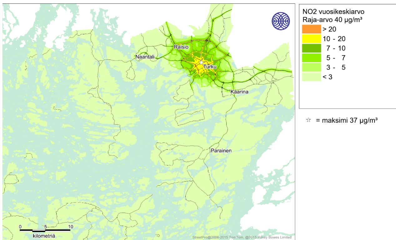
Kuva 4. Autoliikenteen päästöjen yksinään aiheuttama typpidioksidin korkein vuosikeskiarvopitoisuus (µg/m³) Turun seudulla vuonna 2018 ilman alueellista taustapitoisuutta.
