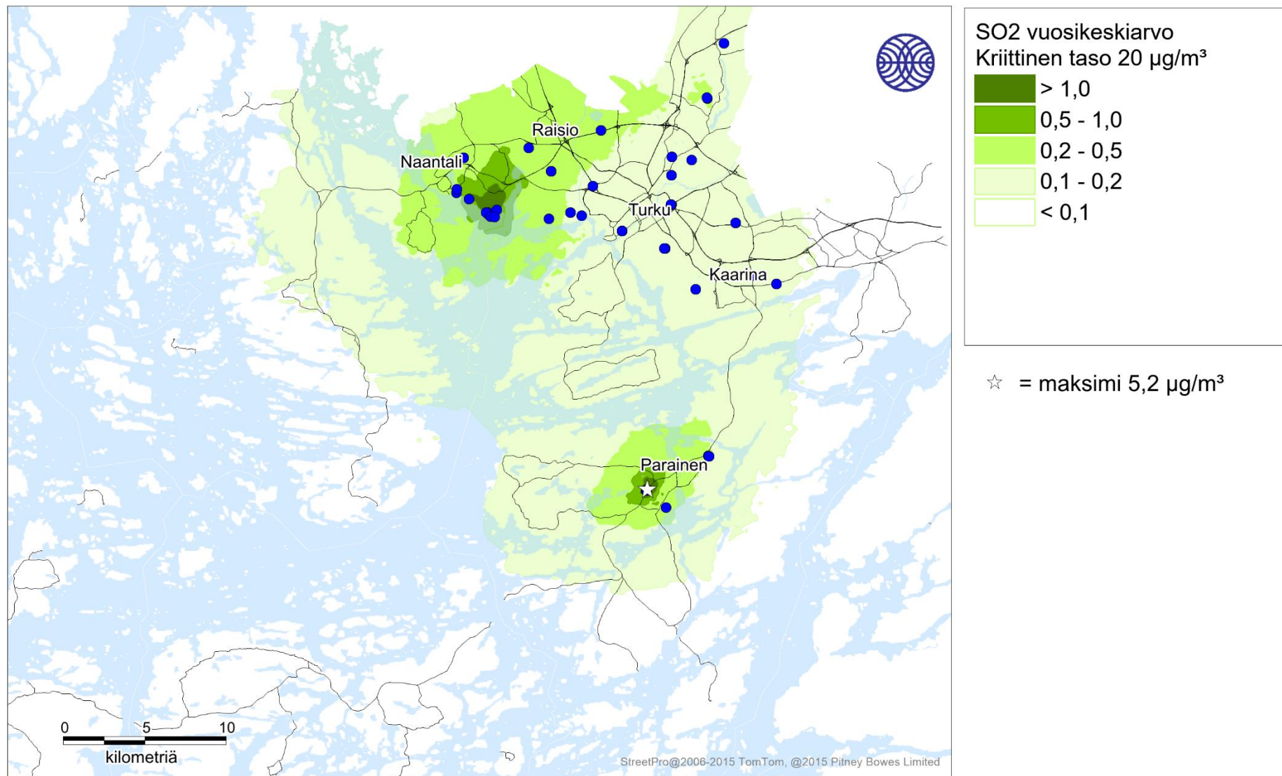
Kuva 51. Energiantuotannon ja teollisuuden päästöjen aiheuttama rikkidioksidin korkein vuosikeskiarvopitoisuus (µg/m³) tarkastelujaksolla 2016-2018.
