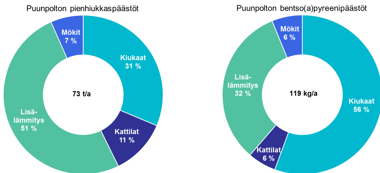
Kuva 48. Turun seudun asuinrakennusten puunpolton aiheuttamat pienhiukkasten päästöt (t/a) ja bentso(a)pyreenin päästöt (kg/a) lämmityslähteittäin vuonna 2018.
