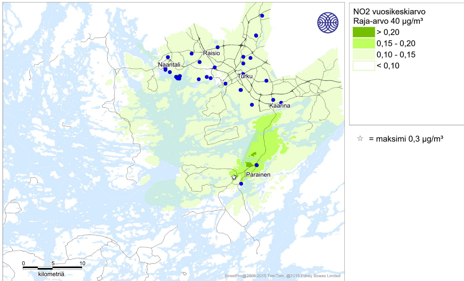
Kuva 9. Energiantuotannon ja teollisuuden päästöjen aiheuttama typpidioksidin korkein vuosikeskiarvopitoisuus (µg/m³) tarkastelujaksolla 2016-2018.
