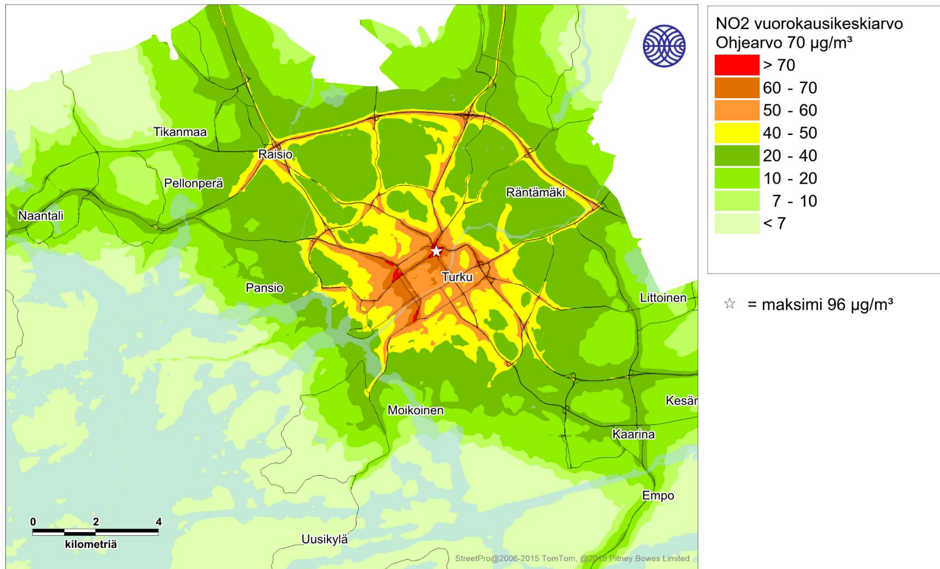
Kuva 8. Autoliikenteen päästöjen aiheuttama typpidioksidin korkein vuorokausiohjearvoon verrannollinen pitoisuus (µg/m 3 ) tarkastelujaksolla 2016-2018.
