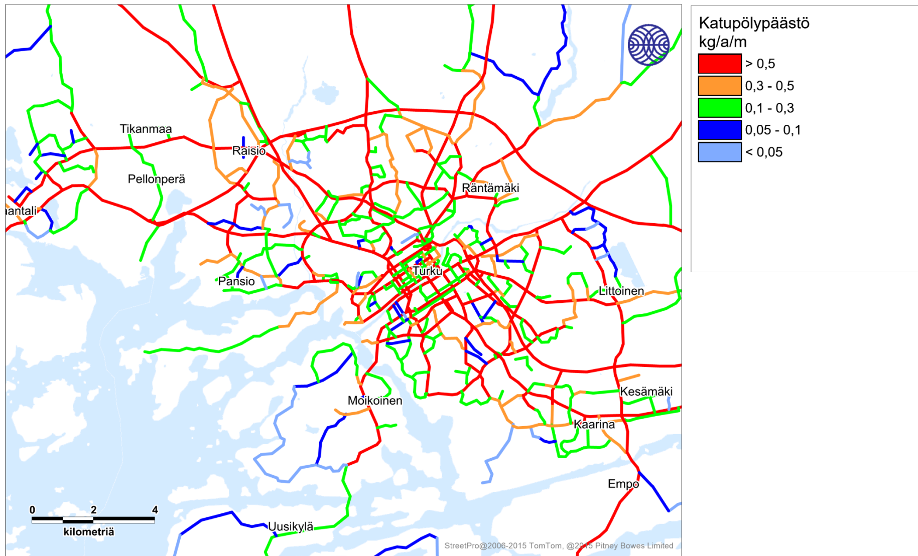
Kuva 66. Liikenteen katupölypäästöt eli PM10-suspensiopäästöt (kg/a/m) vuonna 2018.
