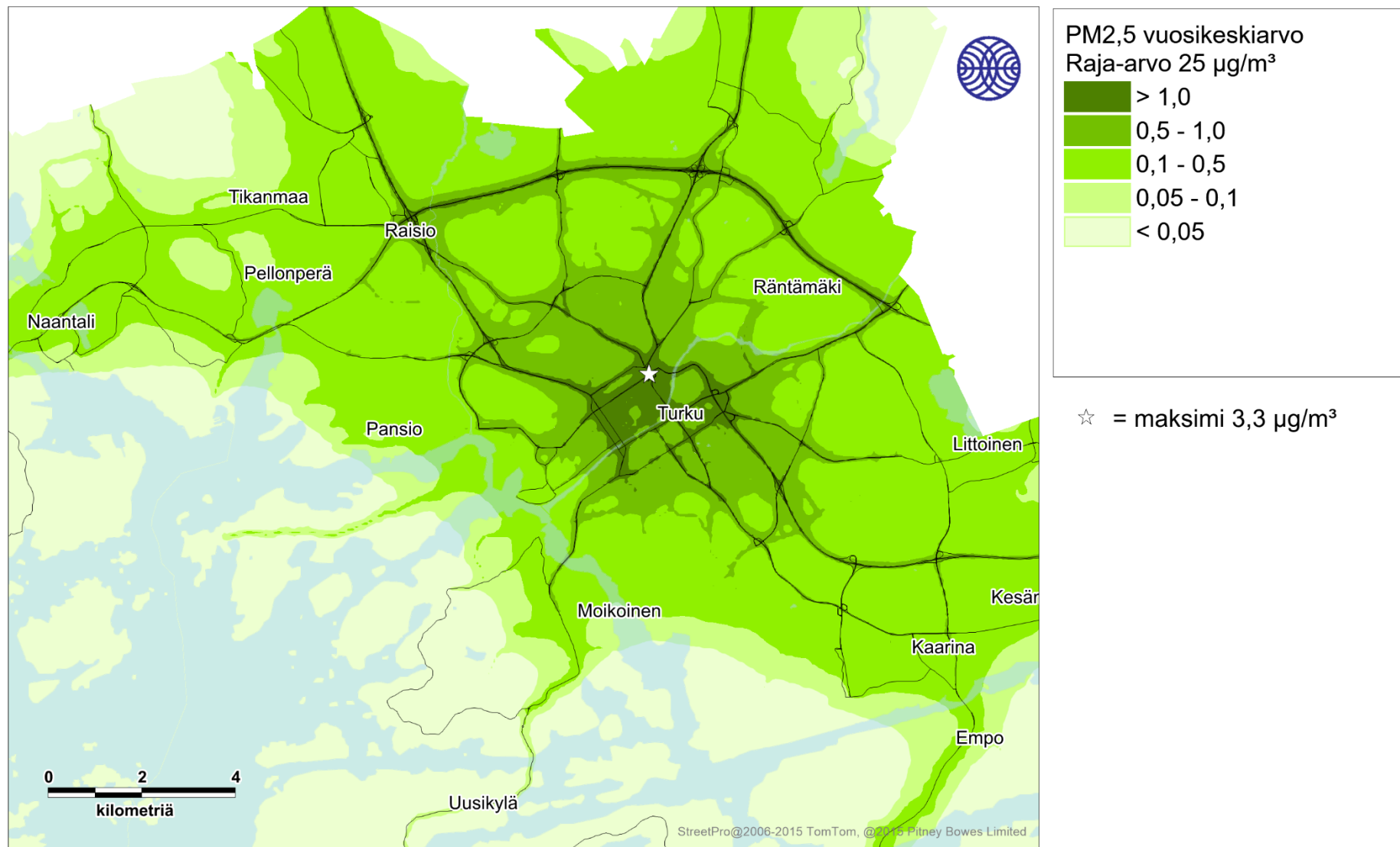
Kuva 24. Autoliikenteen päästöjen aiheuttama pienhiukkasten korkein vuosikeskiarvopitoisuus (µg/m³) tarkastelujaksolla 2016-2018.
