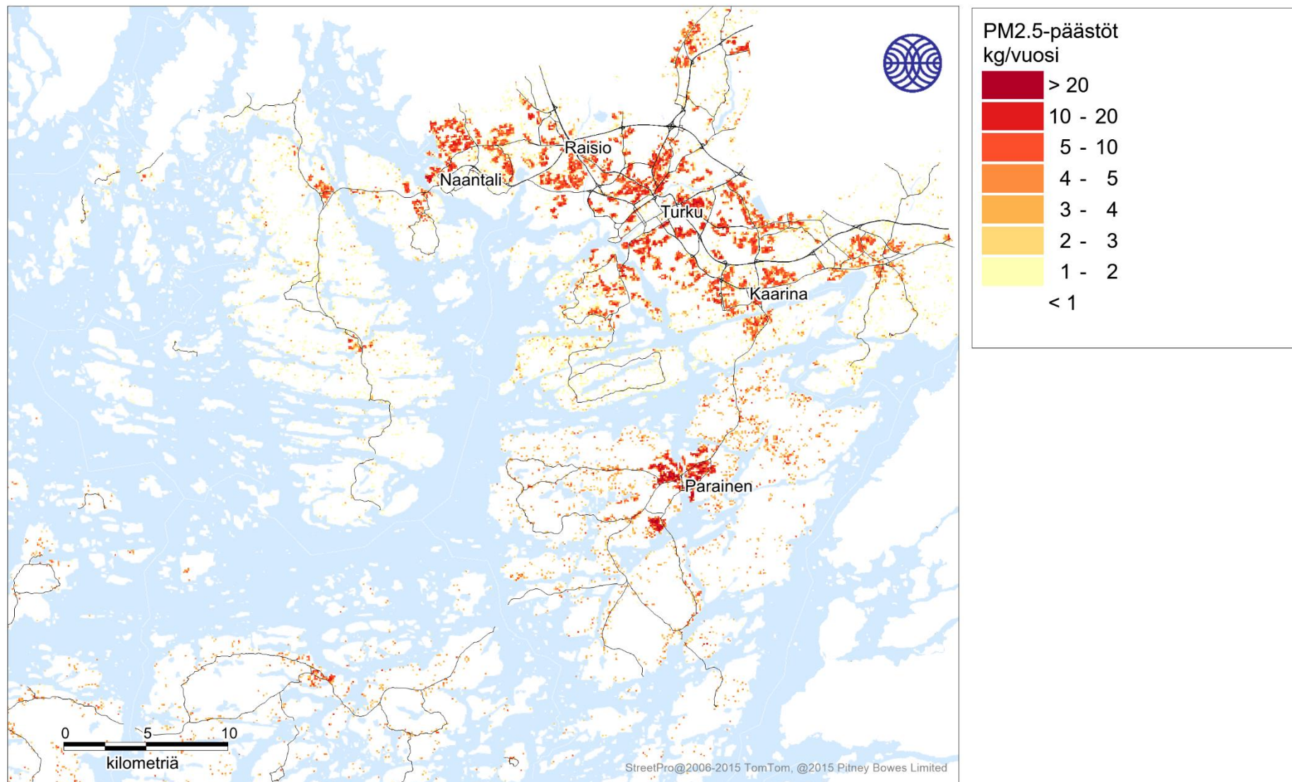
Kuva 74. Puunpolton pienhiukkaspäästöt (kg/a).
