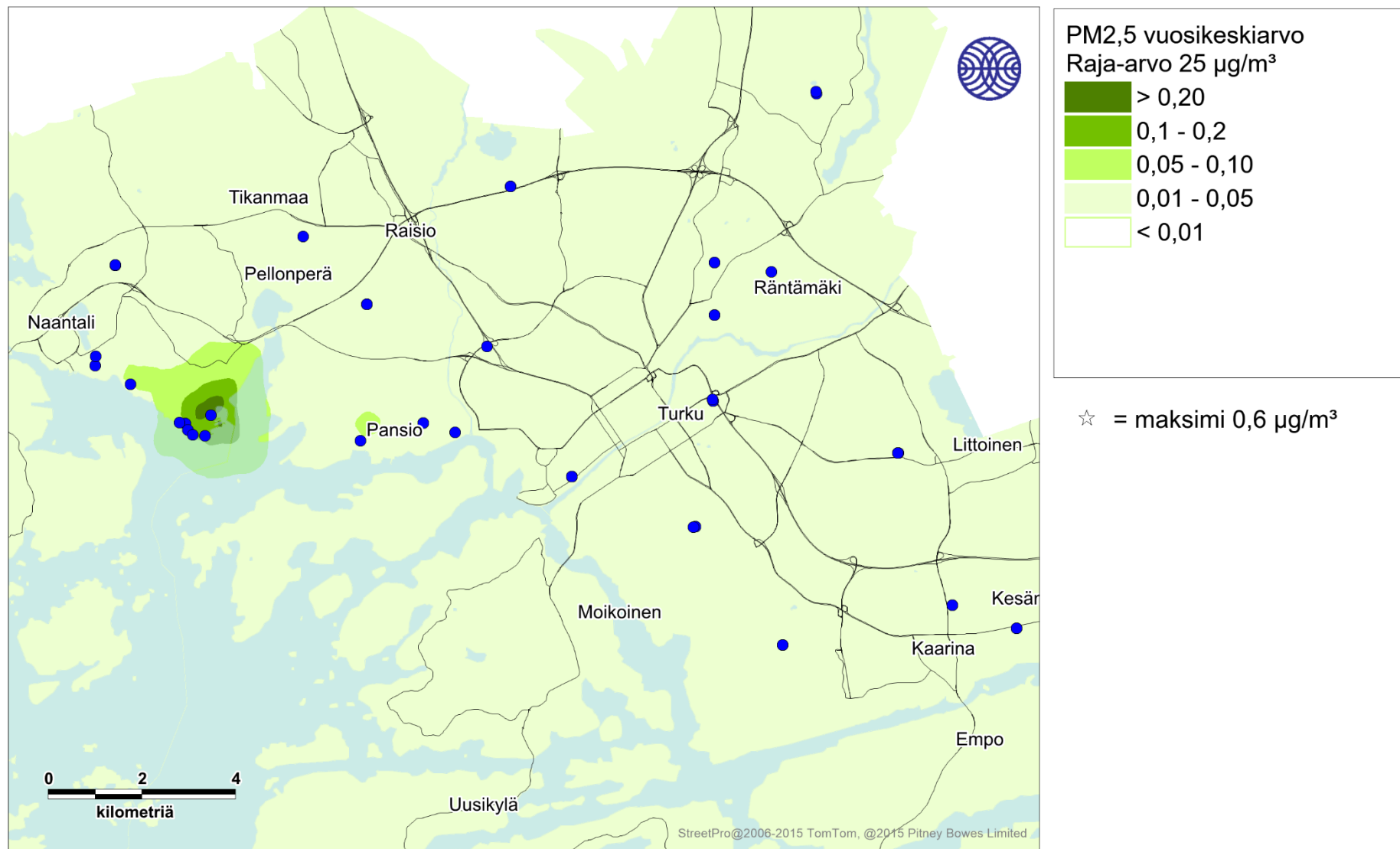
Kuva 28. Energiantuotannon ja teollisuuden päästöjen aiheuttama pienhiukkasten korkein vuosikeskiarvopitoisuus (µg/m³) tarkastelujaksolla 2016-2018.
