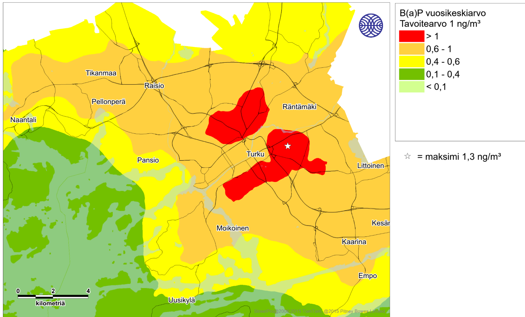
Kuva 60. Puunpolton päästöjen aiheuttama bentso(a)pyreenin korkein vuosikeskiarvopitoisuus (ng/m 3 ) tarkastelujaksolla 2016-2018.
