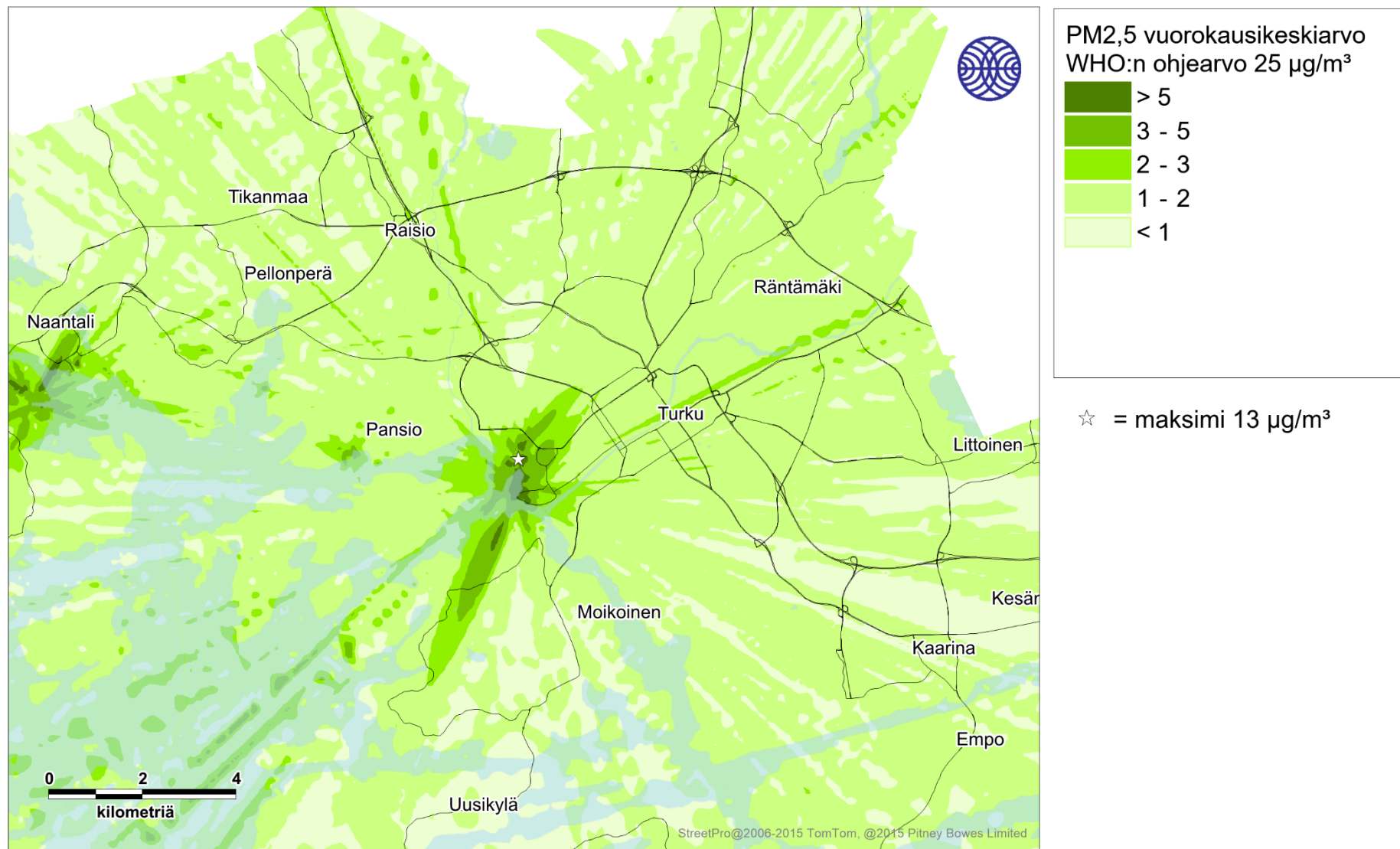
Kuva 34. Laivaliikenteen päästöjen aiheuttama pienhiukkasten korkein WHO:n vuorokausiohjearvoon verrannollinen pitoisuus (µg/m³) tarkastelujaksolla 2016-2018.
