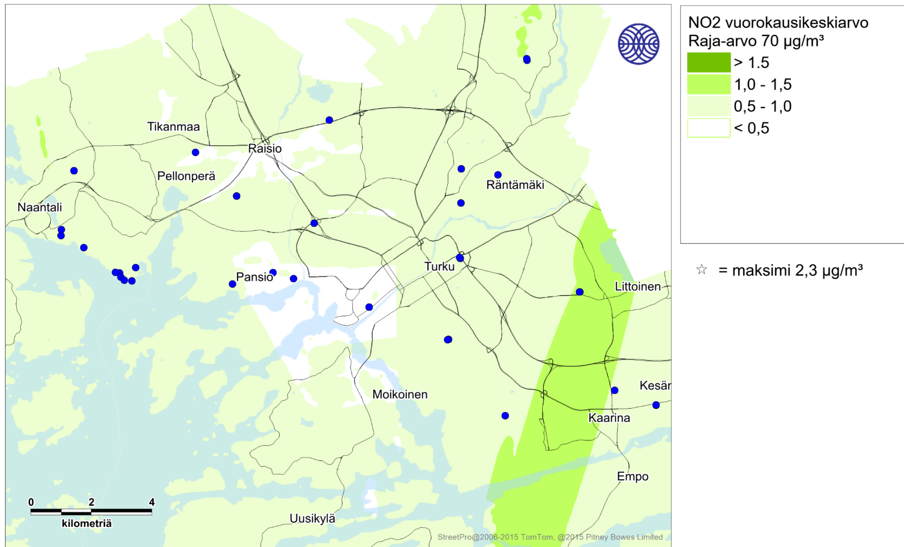
Kuva 12. Energiantuotannon ja teollisuuden päästöjen aiheuttama typpidioksidin korkein vuorokausiohjearvoon verrannollinen pitoisuus (µg/m³) tarkastelujaksolla 2016-2018.
