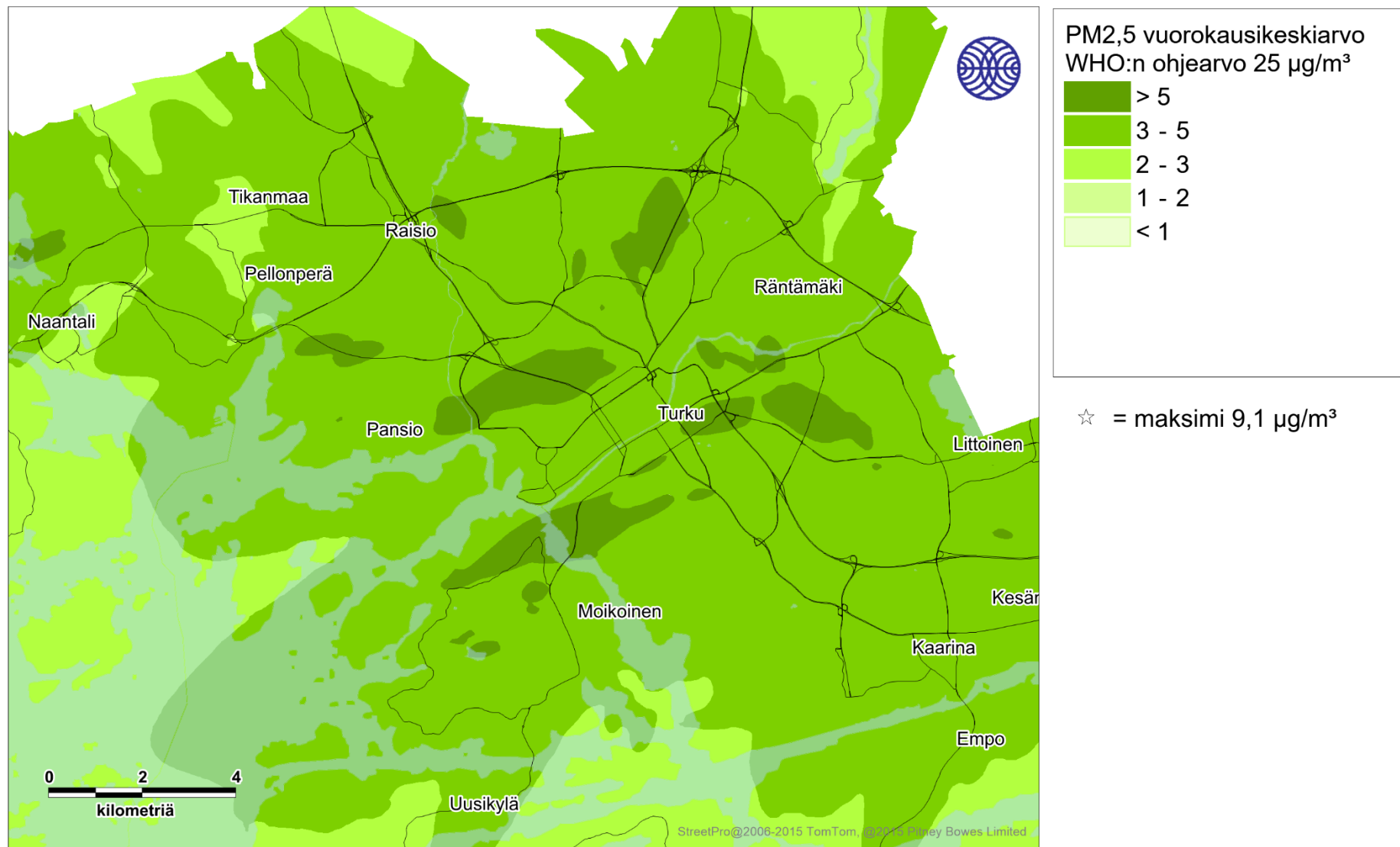
Kuva 38. Puunpolton päästöjen aiheuttama pienhiukkasten korkein WHO:n vuorokausiohjearvoon verrannollinen pitoisuus (µg/m³) tarkastelujaksolla 2016-2018.
