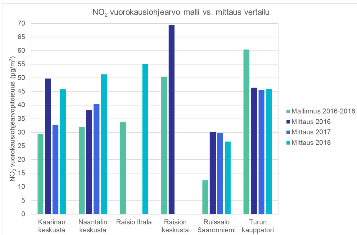
Kuva 23. Mallinnettujen ja mitattujen typidioksidin vuorokausiohjeearvoon (70 µg/m³) verrannollisten pitoisuuksien vertailu Turun seudun ilmanlaadun mittausasemilla.
