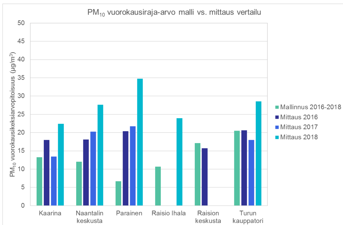
Kuva 27. Mallinnettujen ja mitattujen hengitettävien hiukkasten vuorokausiraja-arvoon (50 µg/m³) verrannollisten pitoisuuksien vertailu Turun seudun ilmanlaadun mittausasemilla.
