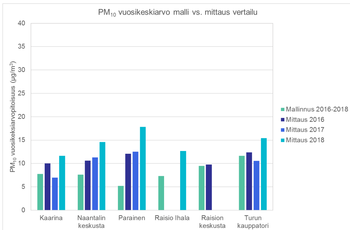
Kuva 26. Mallinnettujen ja mitattujen hengitettävien hiukkasten vuosiraja-arvoon (40 µg/m³) verrannollisten pitoisuuksien vertailu Turun seudun ilmanlaadun mittausasemilla.
