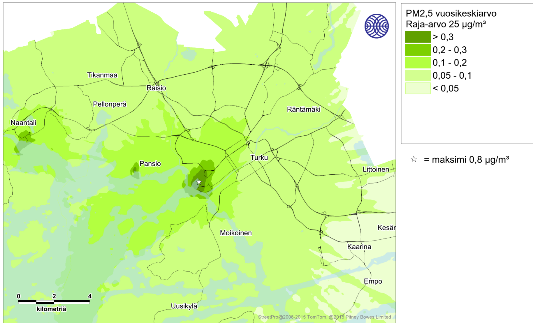
Kuva 32. Laivaliikenteen päästöjen aiheuttama pienhiukkasten korkein vuosikeskiarvopitoisuus (µg/m³) tarkastelujaksolla 2016-2018.
