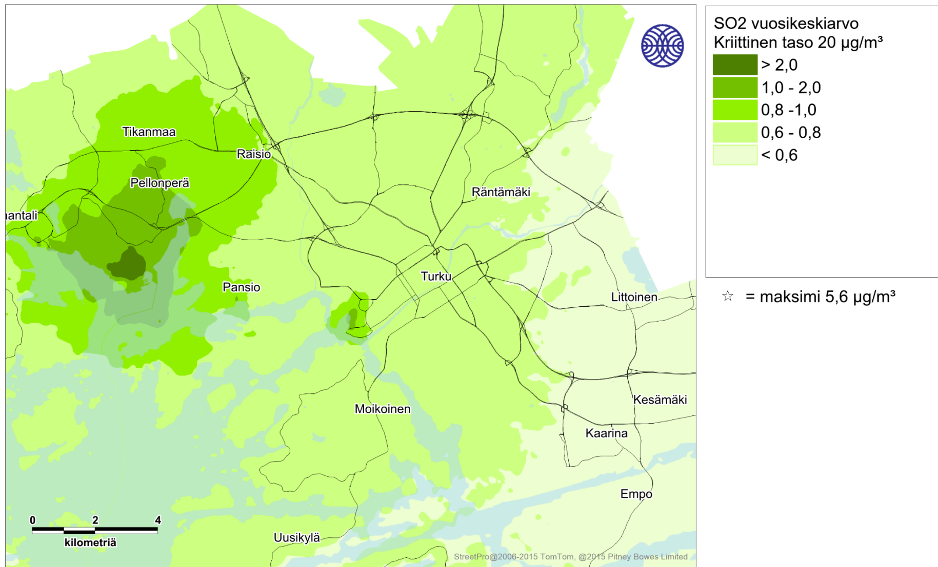
Kuva 48. Kaikkien päästölähteiden yhdessä aiheuttama rikkidioksidin korkein vuosikeskiarvopitoisuus (µg/m 3 ) tarkastelujaksolla 2016-2018.
