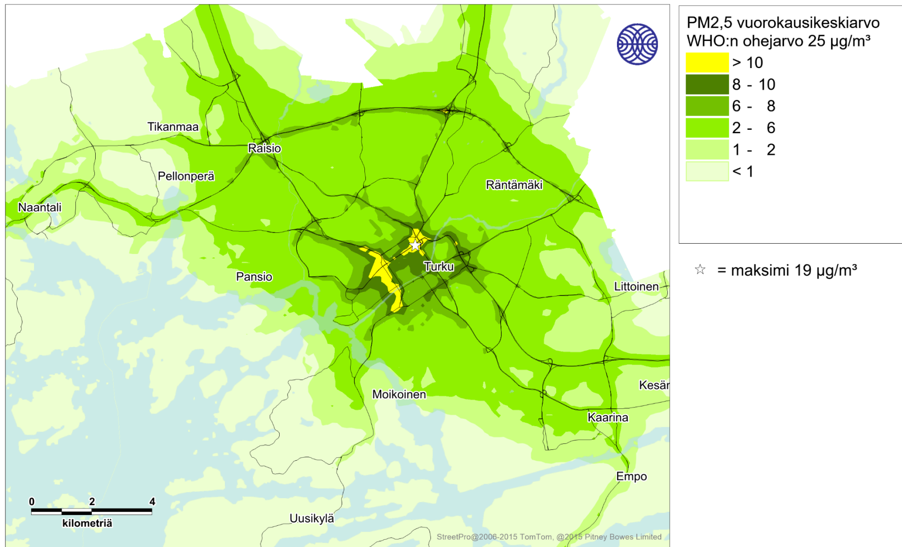
Kuva 26. Autoliikenteen päästöjen aiheuttama pienhiukkasten korkein WHO:n vuorokausiohjearvoon verrannollinen pitoisuus (µg/m³) tarkastelujaksolla 2016-2018.
