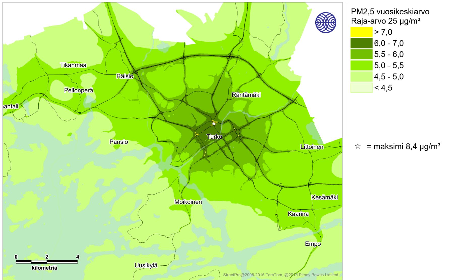
Kuva 20. Kaikkien päästölähteiden ja taustapitoisuuden yhdessä aiheuttama pienhiukkasten korkein vuosikeskiarvopitoisuus (µg/m³) tarkastelujaksolla 2016-2018.
