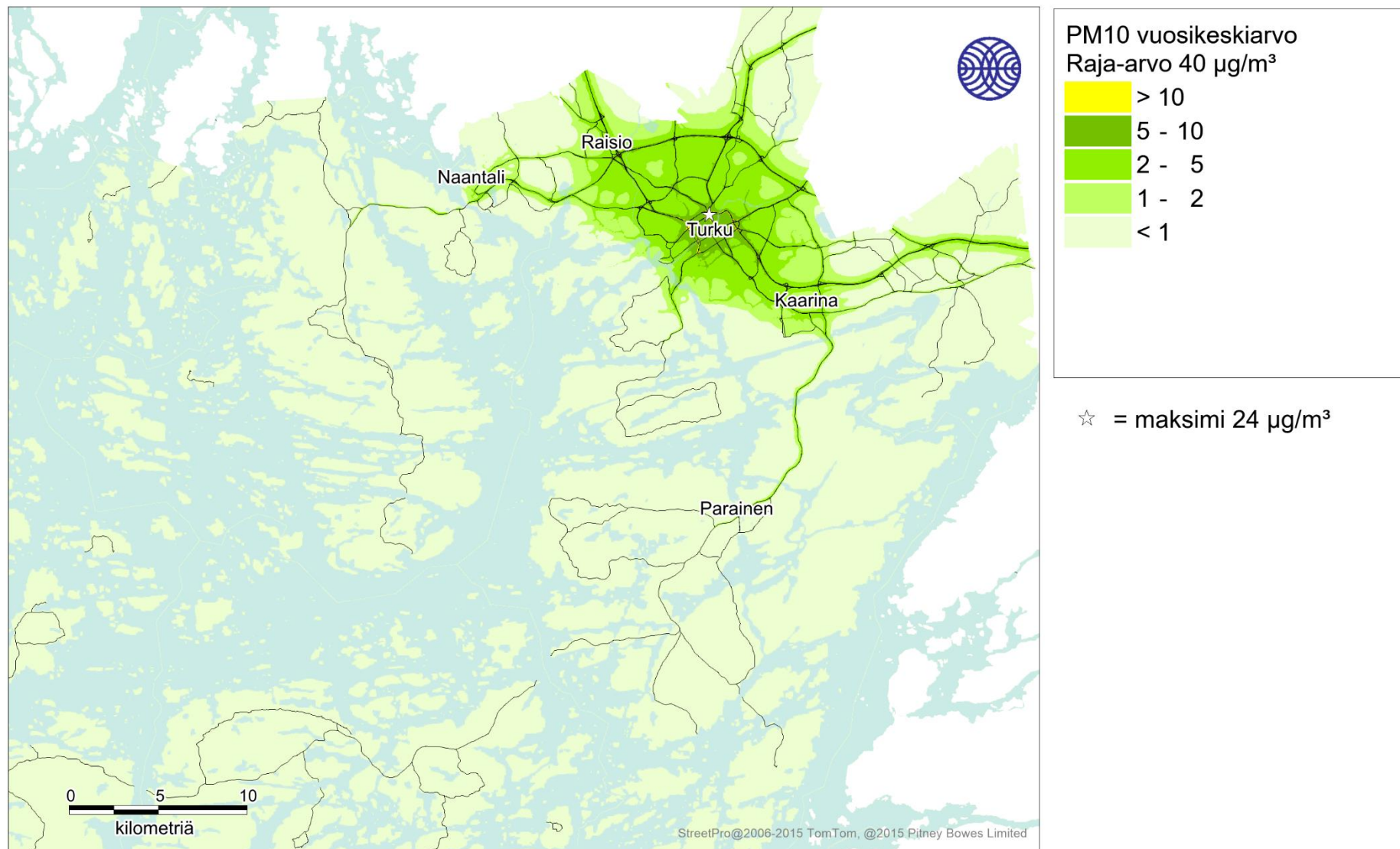
Kuva 43. Autoliikenteen päästöjen aiheuttama hengitettävien hiukkasten korkein vuosikeskiarvopitoisuus (µg/m³) tarkastelujaksolla 2016-2018.
