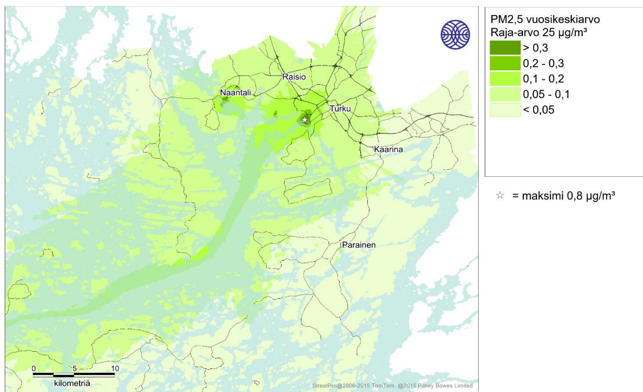
Kuva 11. Laivaliikenteen päästöjen yksinään aiheuttama pienhiukkasten korkein vuosikeskiarvopitoisuus (µg/m³) Turun seudulla vuonna 2018 ilman alueellista taustapitoisuutta.
