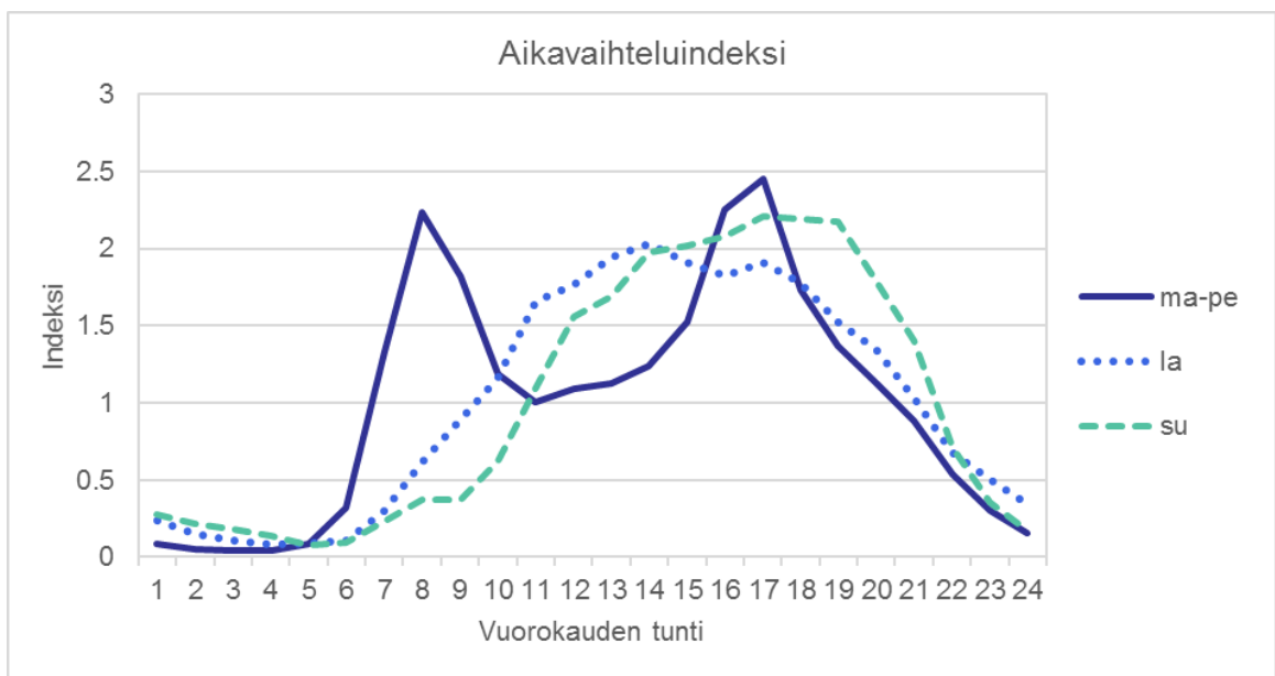
Kuva 42. Mallilaskelmissa käytetyt liikenteen tunneittaista vaihtelua kuvaavat aikavaihteluindeksit LAM-pisteessä 239 (vt1 Kaarina).
