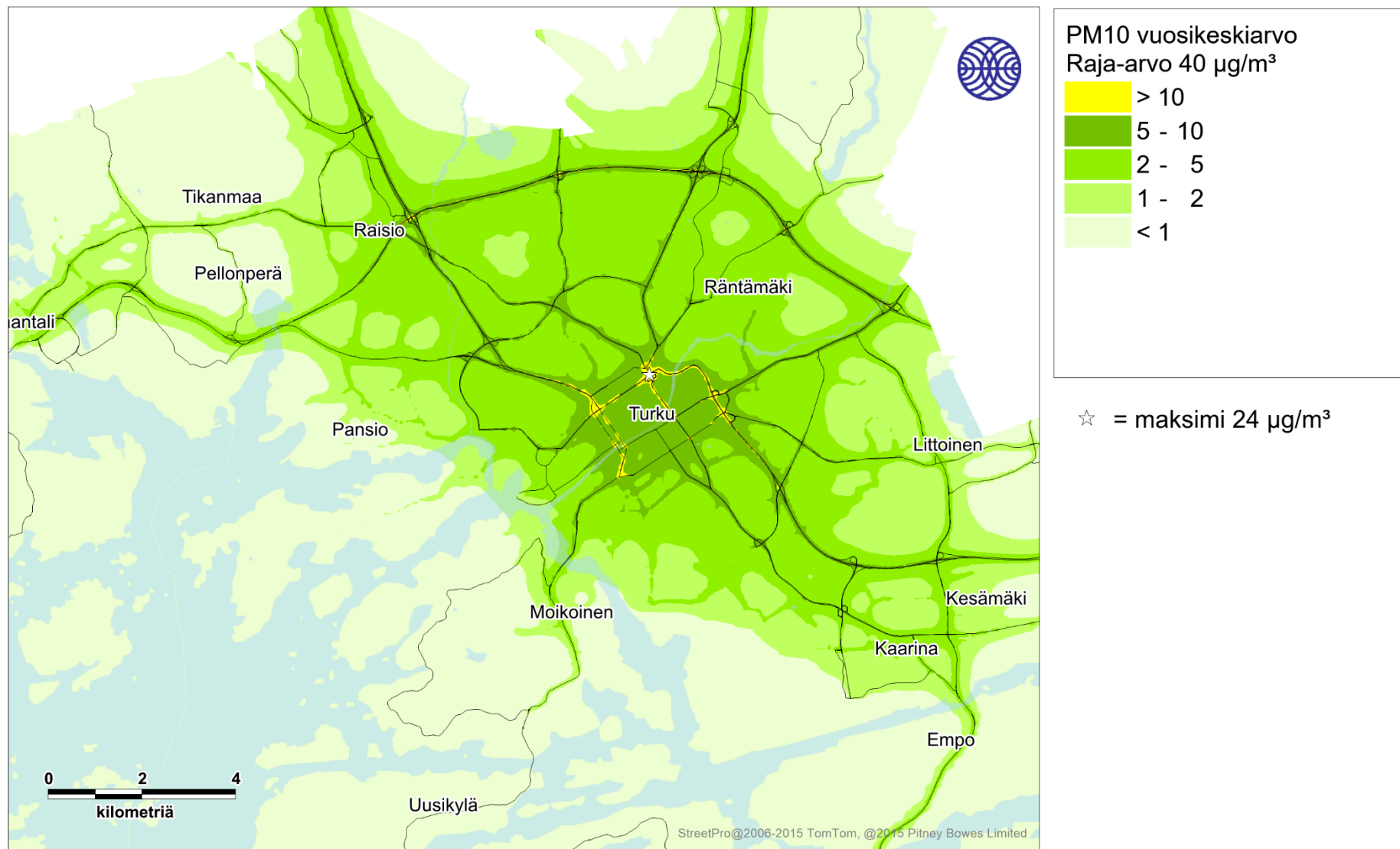
Kuva 44. Autoliikenteen päästöjen aiheuttama hengitettävien hiukkasten korkein vuosikeskiarvopitoisuus (µg/m³) tarkastelujaksolla 2016-2018.
