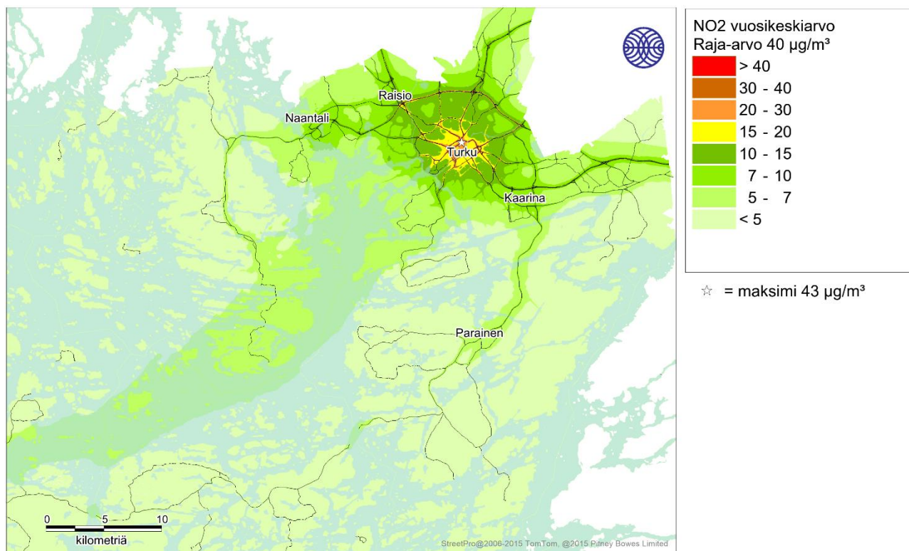
Kuva 1. Autoliikenteen, energiantuotannon, teollisuuden ja laivaliikenteen päästöjen sekä alueellisen taustapitoisuuden (vuosikeskiarvona 3,7 µg/m³) yhdessä aiheuttama typpidioksidin (NO 2 ) korkein vuosikeskiarvopitoisuus (µg/m³) Turun seudulla vuonna 2018.
