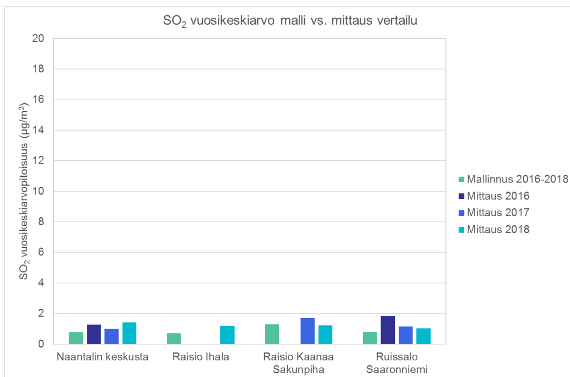
Kuva 28. Mallinnettujen ja mitattujen rikkidioksidin kriittiseen tasoon ( 20 \mu\text{g}/\text{m}^3 ) verrannollisten vuosikeskiarvopitoisuuksien vertailu Turun seudun ilmanlaadun mittausasemilla.
