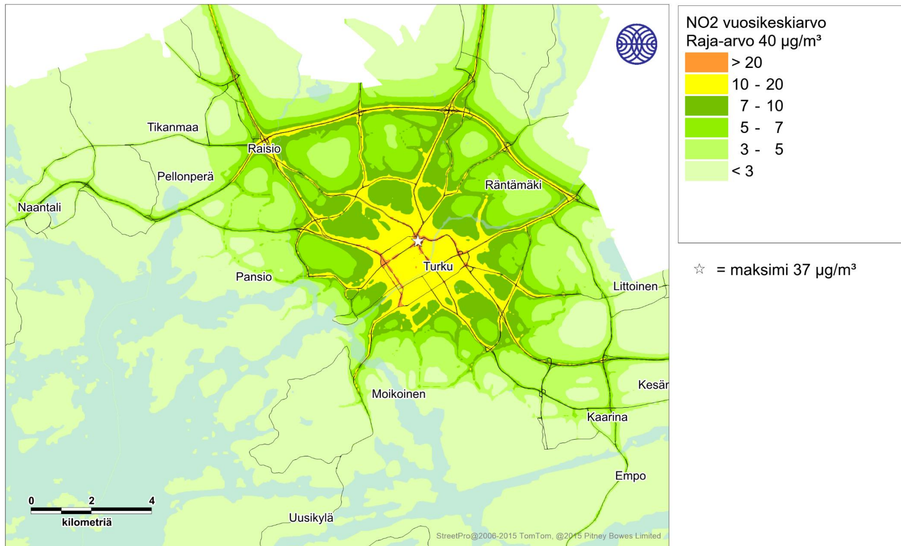
Kuva 6. Autoliikenteen päästöjen aiheuttama typidioksidin korkein vuosikeskiarvopitoisuus (µg/m³) tarkastelujaksolla 2016-2018.
