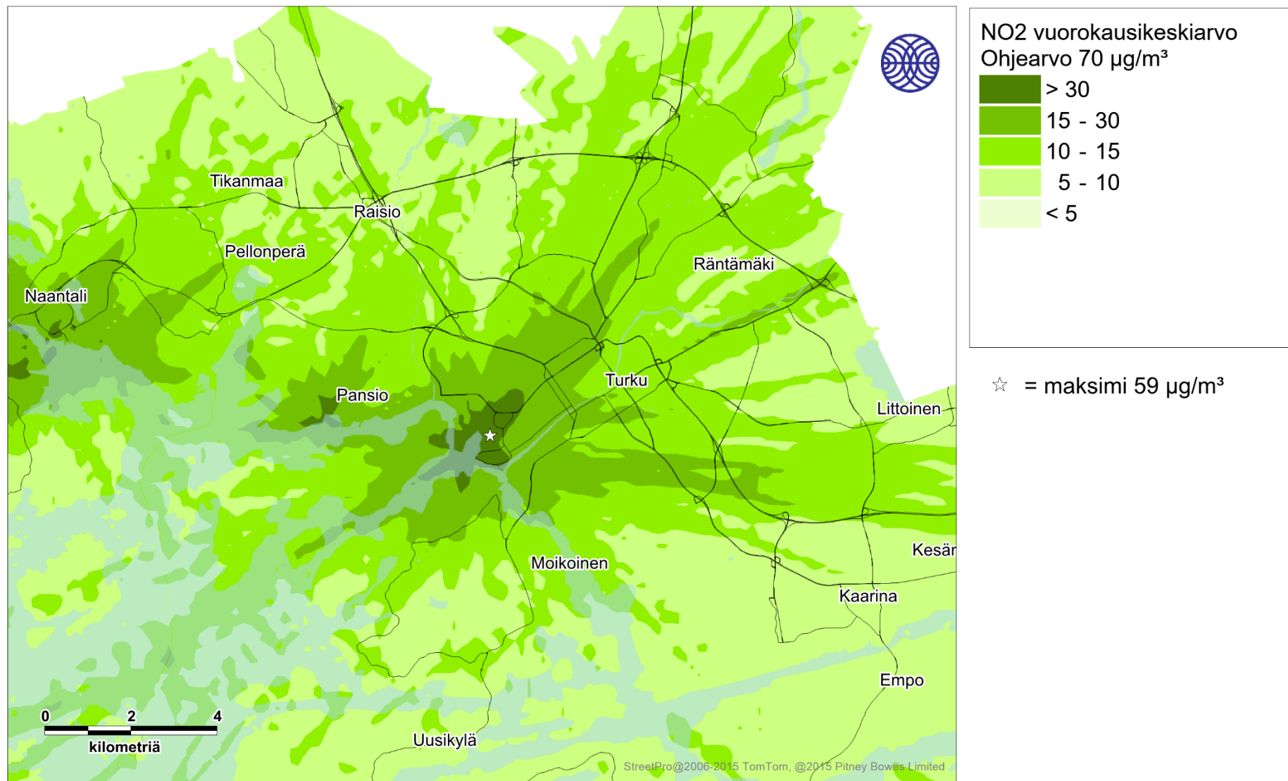
Kuva 16. Laivaliikenteen päästöjen aiheuttama typpidioksidin korkein vuorokausiohjearvoon verrannollinen pitoisuus (µg/m³) tarkastelujaksolla 2016-2018.
