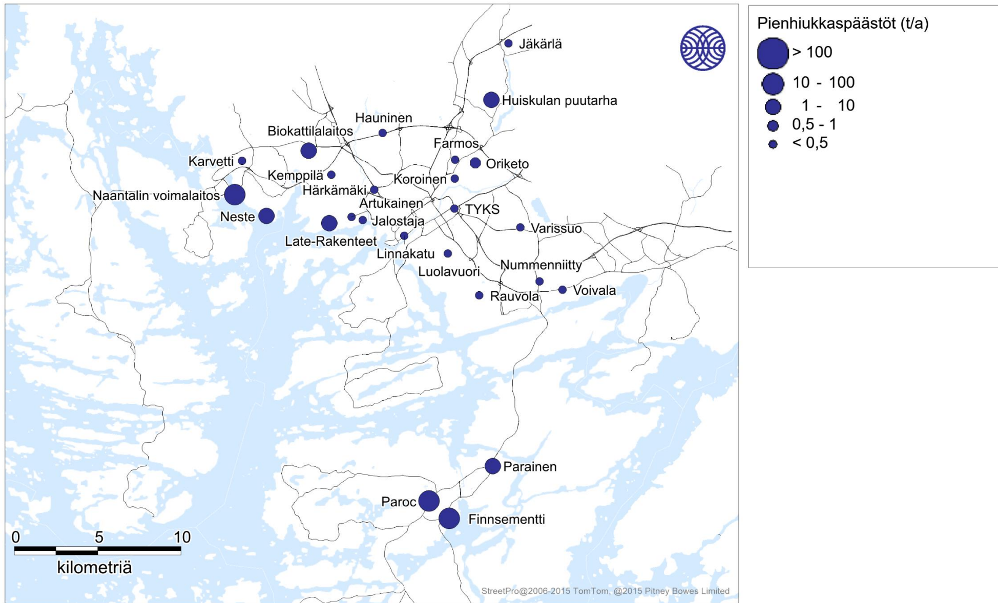
Kuva 68. Energiantuotannon ja teollisuuden pienhiukkaspäästöt (t/a) vuonna 2018.
