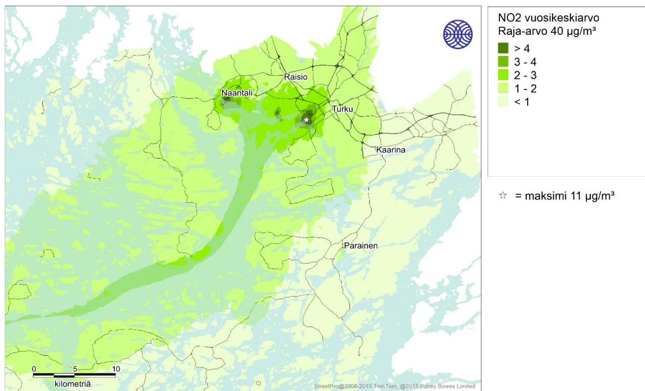
Kuva 6. Laivaliikenteen päästöjen yksinään aiheuttama typpidioksidin korkein vuosikeskiarvopitoisuus (µg/m³) Turun seudulla vuonna 2018 ilman alueellista taustapitoisuutta.
