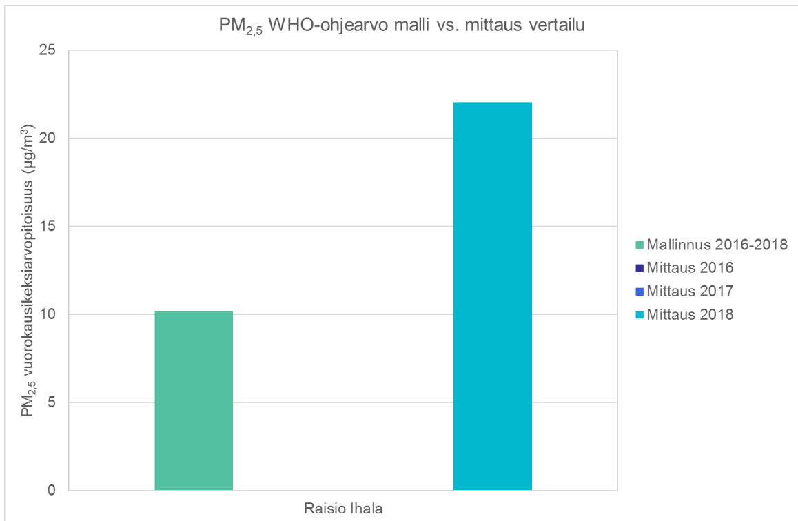
Kuva 25. Mallinnettujen ja mitattujen pienhiukkasten WHO:n ohjearvoon ( 25 \mu\text{g}/\text{m}^3 ) verrannollisten pitoisuuksien vertailu Raision Ihalan ilmanlaadun mittausasemalla.
