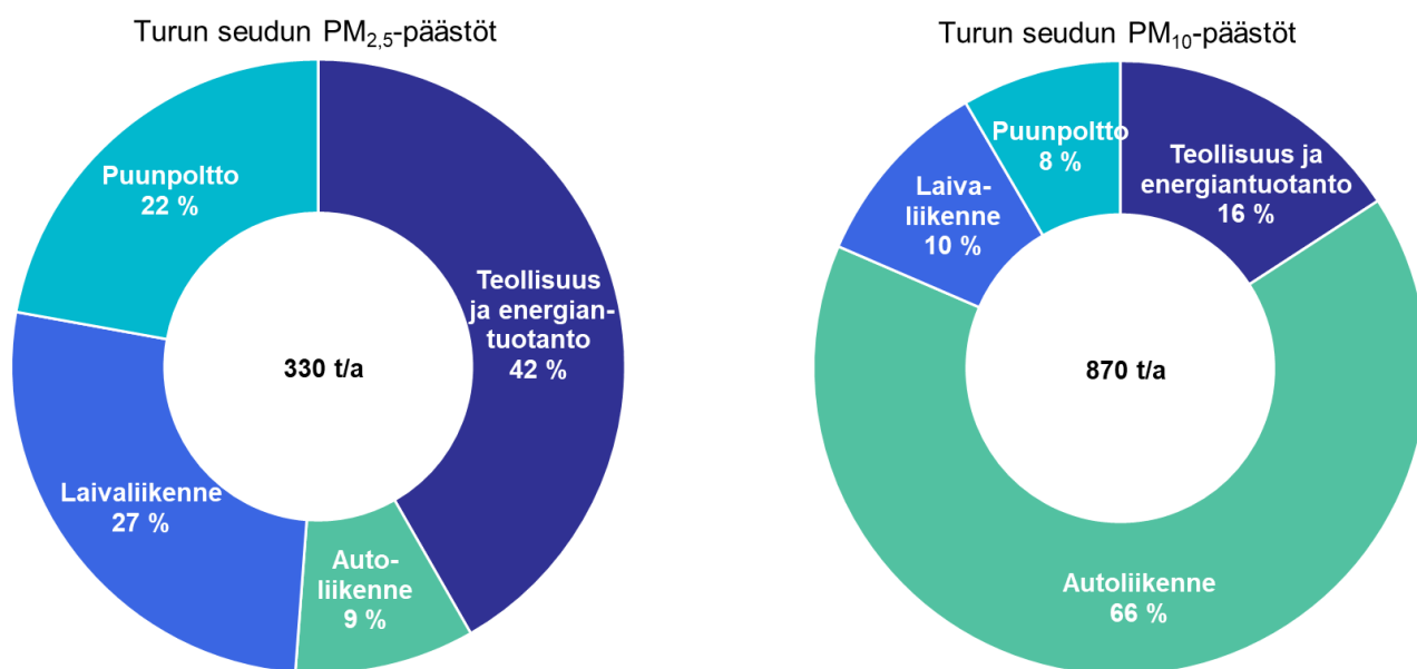
Kuva 40. Turun seudun pienhiukkasten ja hengitettävien hiukkasten kokonaispäästöt sekä eri päästölähteiden osuudet vuonna 2018.
