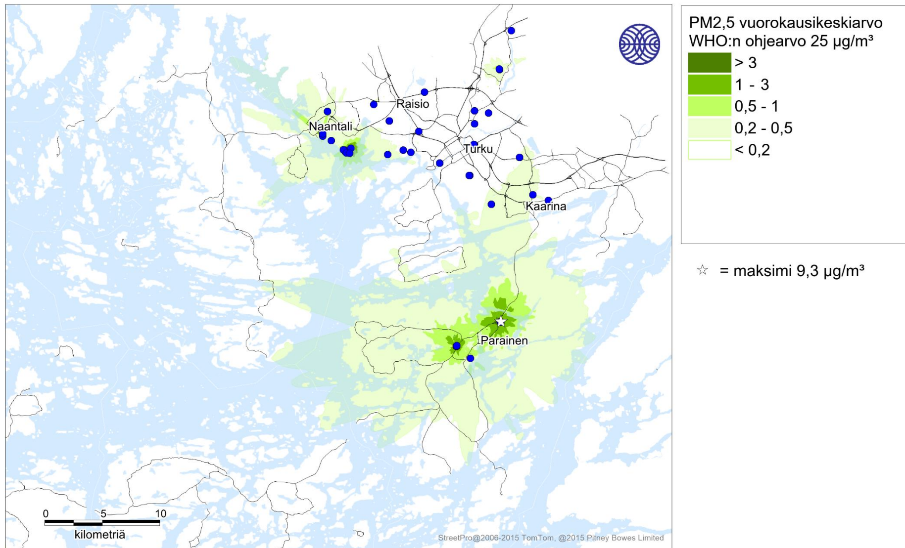
Kuva 29. Energiantuotannon ja teollisuuden päästöjen aiheuttama pienhiukkasten korkein WHO:n vuorokausiohjearvoon verrannollinen pitoisuus (µg/m³) tarkastelujaksolla 2016-2018.
