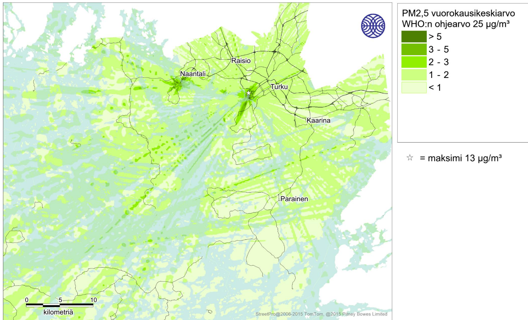
Kuva 33. Laivaliikenteen päästöjen aiheuttama pienhiukkasten korkein WHO:n vuorokausiohjearvoon verrannollinen pitoisuus (µg/m³) tarkastelujaksolla 2016-2018.
