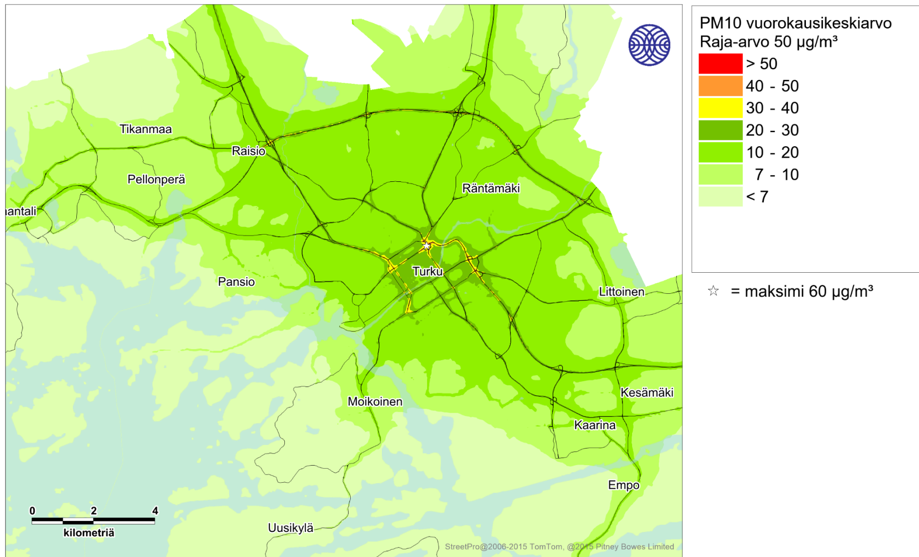
Kuva 42. Kaikkien päästölähteiden ja taustapitoisuuden aiheuttama hengitettävien hiukkasten korkein vuorokausiraja-arvoon verrannollinen pitoisuus (µg/m³) tarkastelujaksolla 2016-2018.
