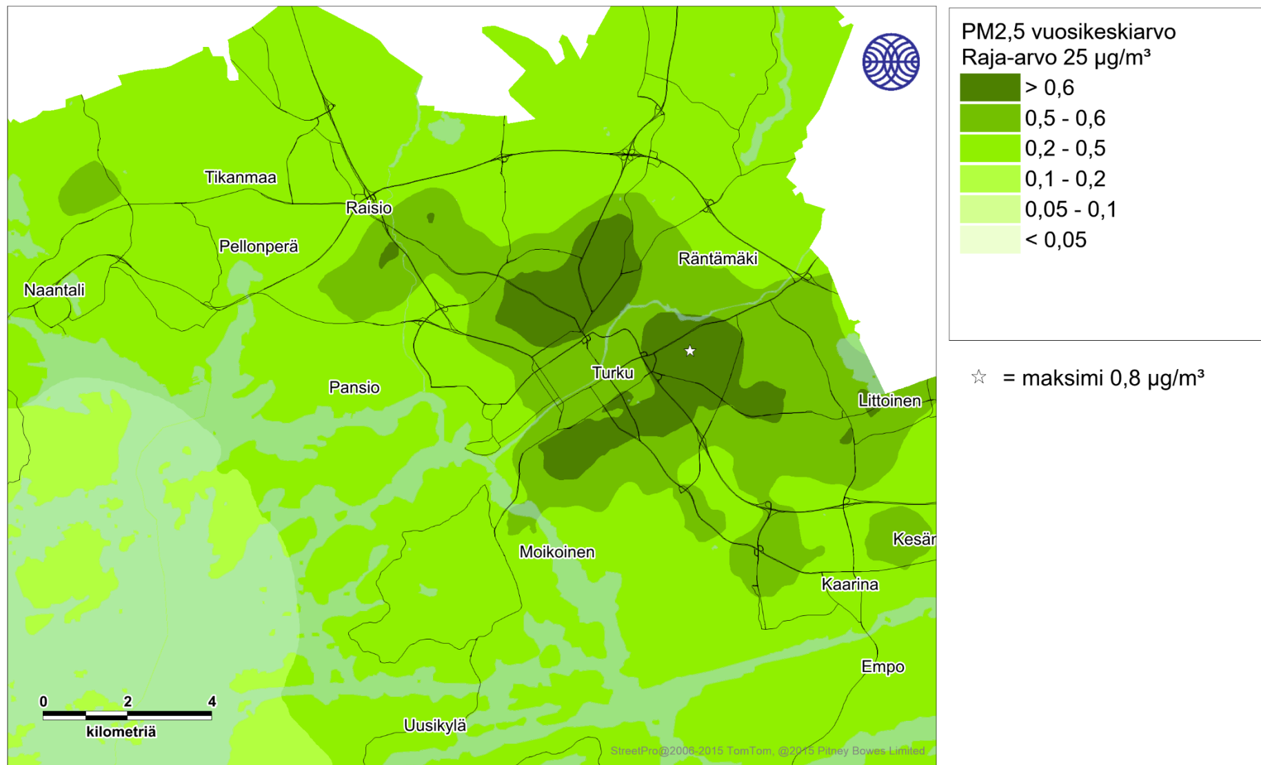
Kuva 36. Puunpolton päästöjen aiheuttama pienhiukkasten korkein vuosikeskiarvopitoisuus (µg/m³) tarkastelujaksolla 2016-2018.
