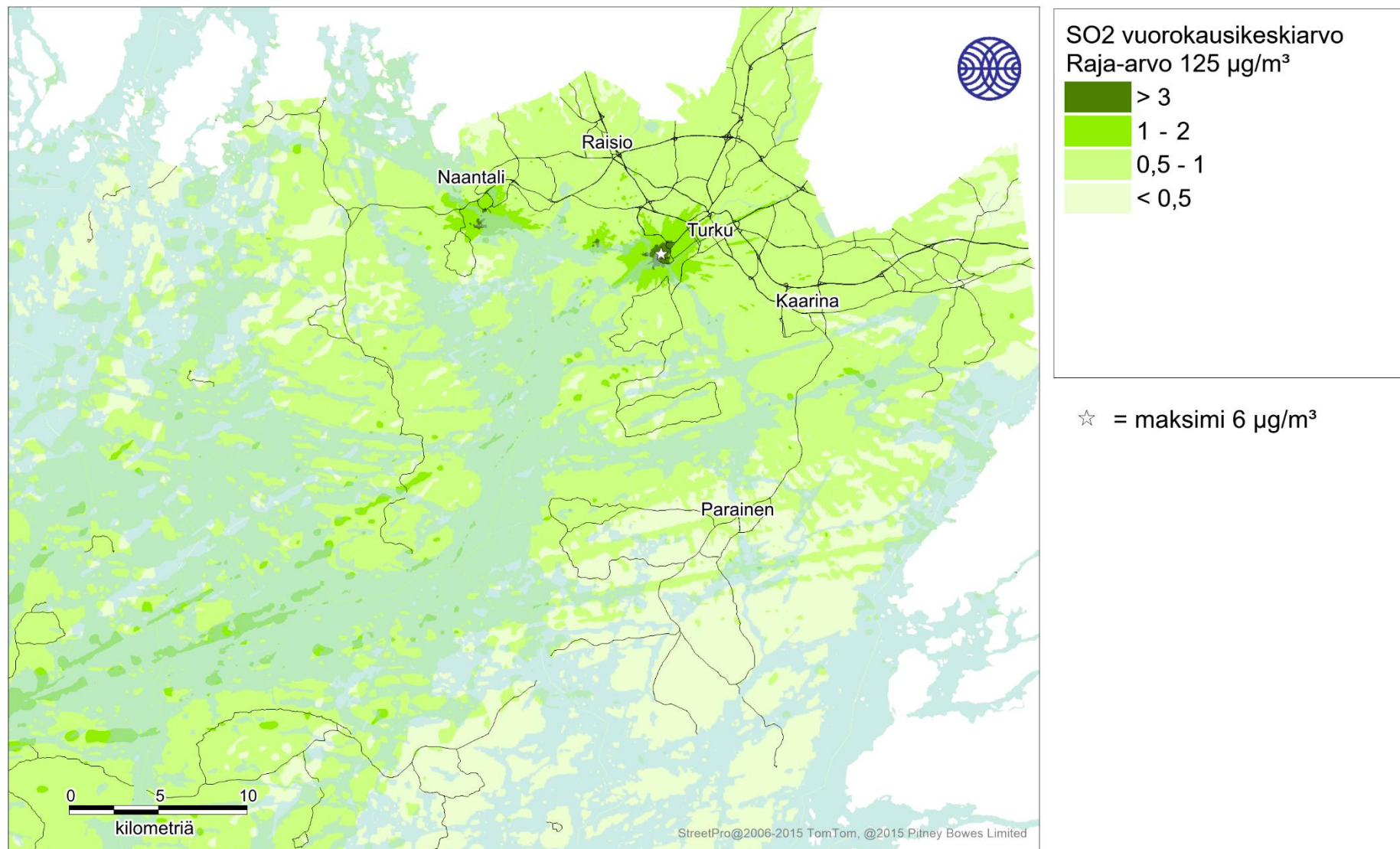
Kuva 57. Laivaliikenteen päästöjen aiheuttama rikkidioksidin korkein vuorokausiraja-arvoon verrannollinen pitoisuus (µg/m³) tarkastelujaksolla 2016-2018.
