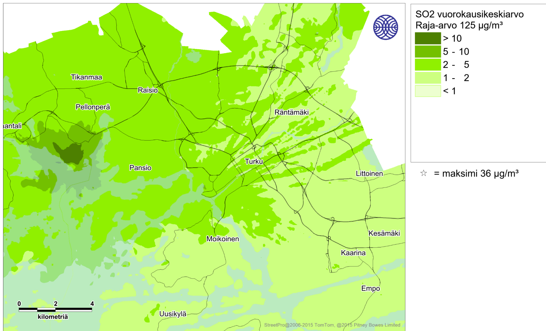
Kuva 50. Kaikkien päästölähteiden yhdessä aiheuttama rikkidioksidin korkein vuorokausiraja-arvoon verrannollinen pitoisuus (µg/m³) tarkastelujaksolla 2016-2018.
