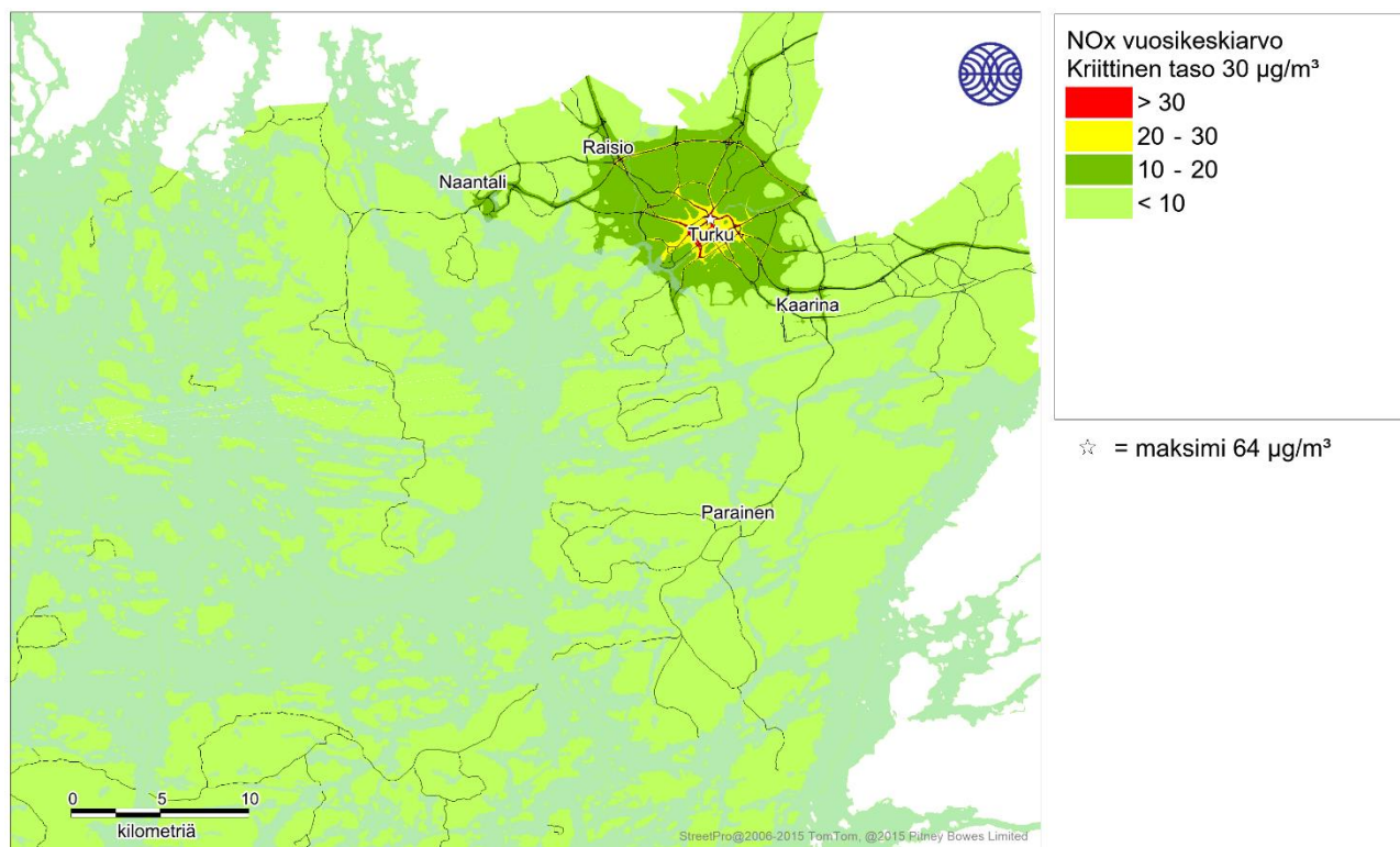
Kuva 3. Autoliikenteen, energiantuotannon, teollisuuden ja laivaliikenteen päästöjen sekä alueellisen taustapitoisuuden (vuosikeskiarvona 3,7 µg/m³) yhdessä aiheuttama typen oksidien (NO x ) korkein vuosikeskiarvopitoisuus (µg/m³) Turun seudulla vuonna 2018.
