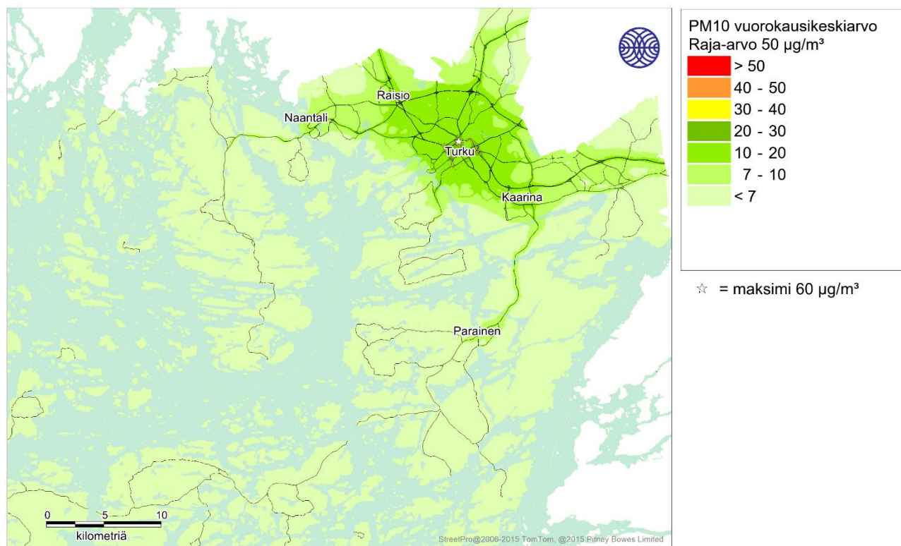
Kuva 14. Autoliikenteen, energiantuotannon, teollisuuden, laivaliikenteen ja asuinrakennusten puunpoltton päästöjen sekä pienhiukkasten alueellisen taustapitoisuuden (vuosikeskiarvona 4,4 µg/m³) aiheuttama hengitettävien hiukkasten vuorokausiraja-arvoon verrannollinen pitoisuus (µg/m³) Turun seudulla vuonna 2018.
