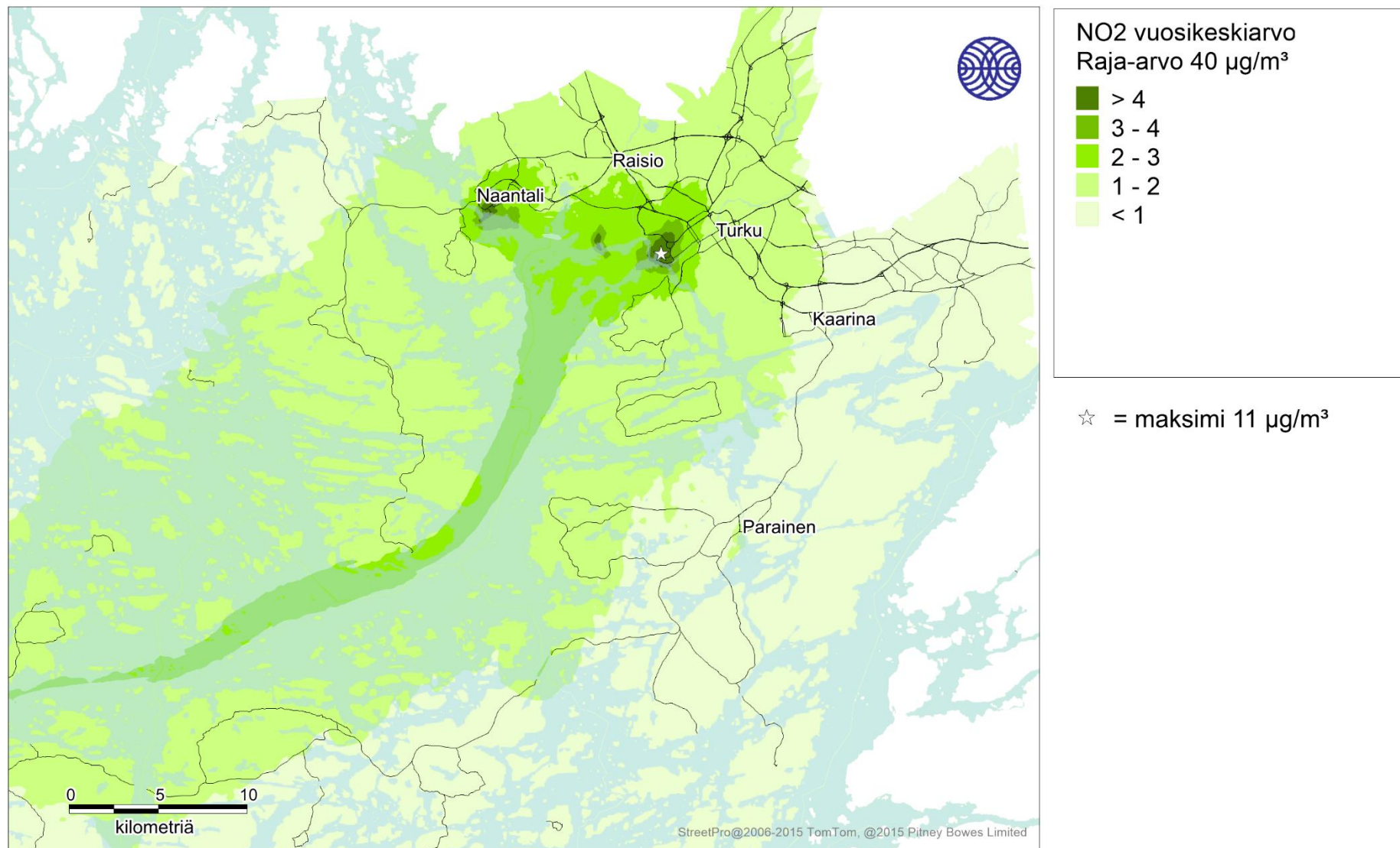
Kuva 13. Laivaliikenteen päästöjen aiheuttama typpidioksidin korkein vuosikeskiarvopitoisuus (µg/m³) tarkastelujaksolla 2016-2018.
