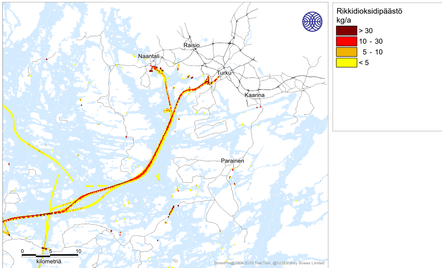
Kuva 73. Laivaliikenteen SO 2 -päästöt (kg/a/m) vuonna 2018.
