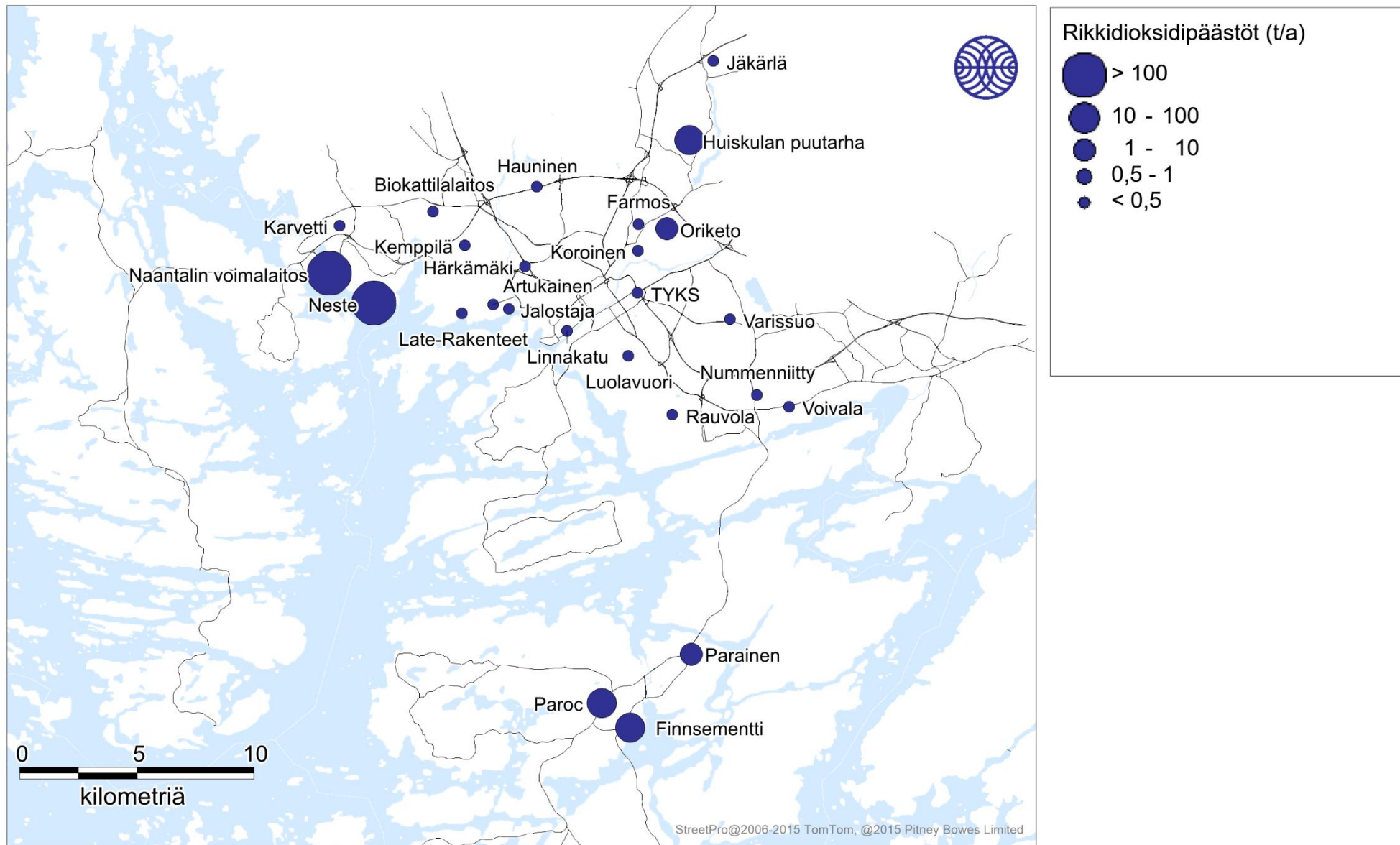
Kuva 69. Energiantuotannon ja teollisuuden rikkidioksidipäästöt (t/a) vuonna 2018.
