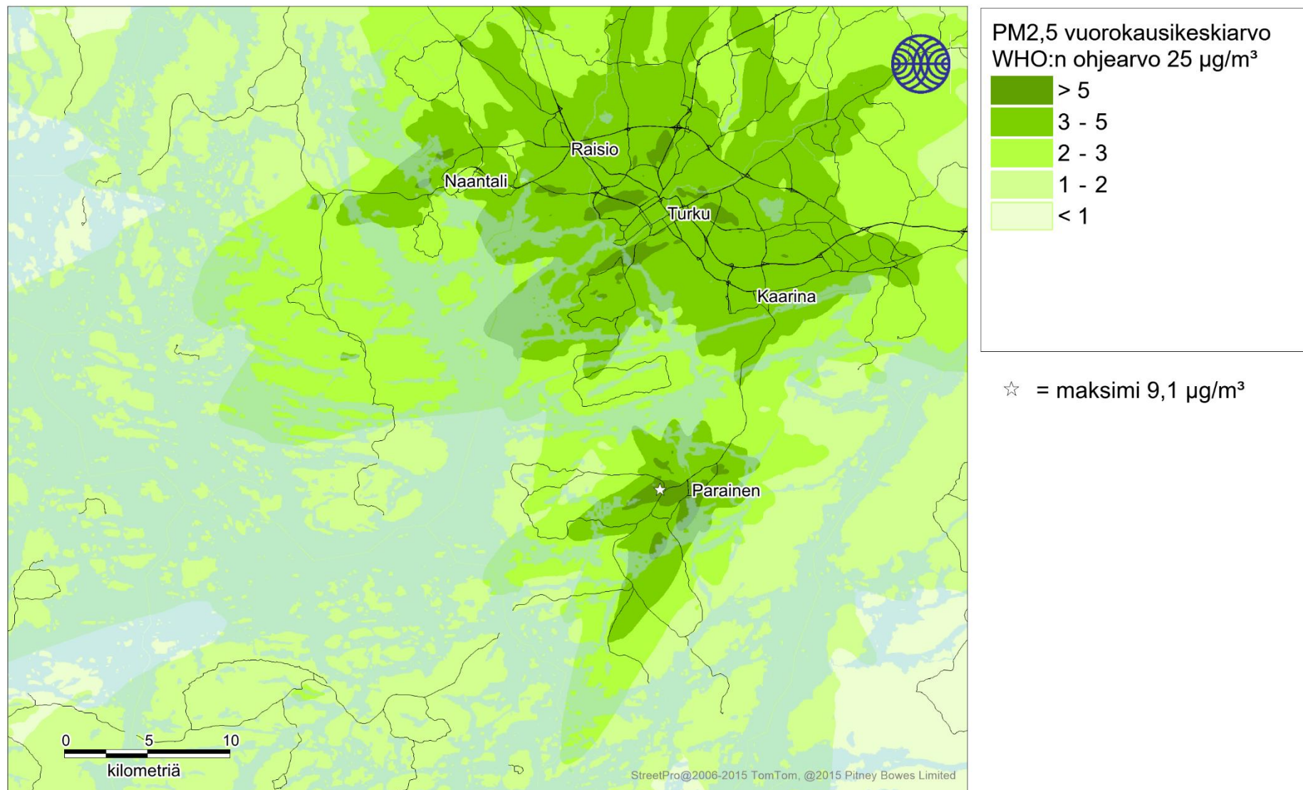
Kuva 37. Puunpolton päästöjen aiheuttama pienhiukkasten korkein WHO:n vuorokausiohjearvoon verrannollinen pitoisuus (µg/m³) tarkastelujaksolla 2016-2018.
