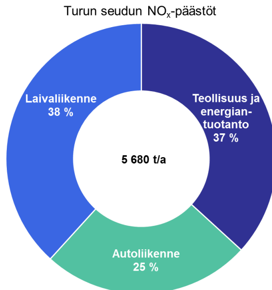
Kuva 39. Turun seudun typen oksidien kokonaispäästöt sekä eri päästölähteiden osuudet vuonna 2018.
