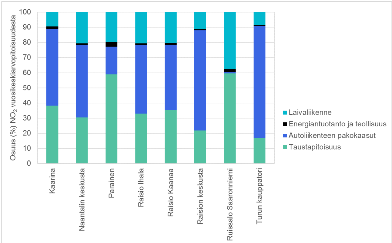
Kuva 31. Eri päästölähdesektoreiden osuus mallinnetuista tyyppidioksidin vuosikeskiarvopitoisuuksista ilmanlaadun mittauspisteissä vuonna 2018.
