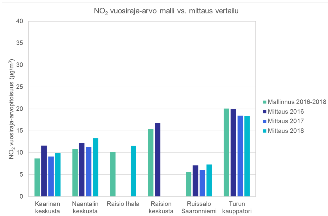
Kuva 22. Mallinnettujen ja mitattujen typidioksidin vuosiraja-arvoon (40 µg/m³) verrannollisten pitoisuuksien vertailu Turun seudun ilmanlaadun mittausasemilla.
