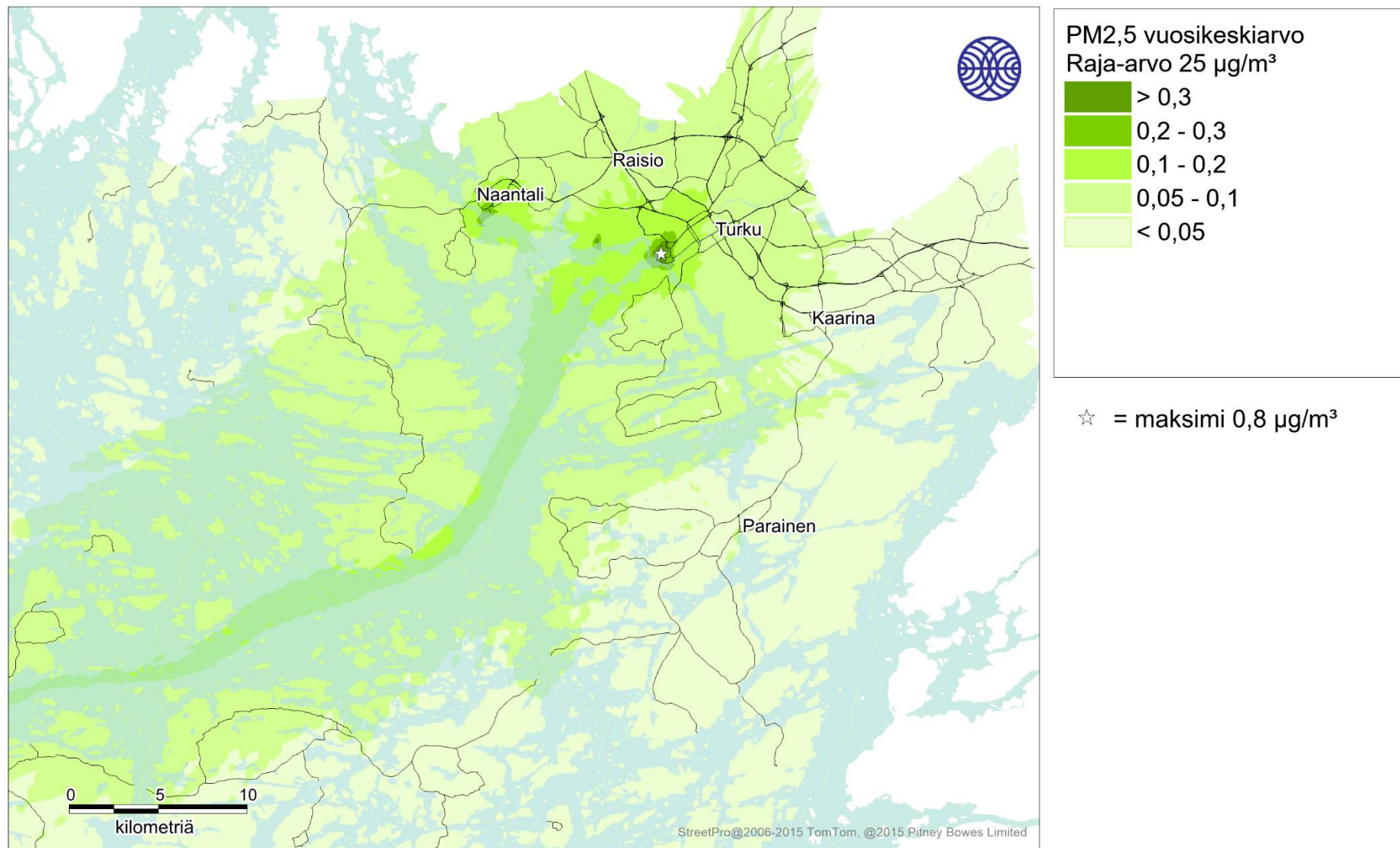
Kuva 31. Laivaliikenteen päästöjen aiheuttama pienhiukkasten korkein vuosikeskiarvopitoisuus (µg/m³) tarkastelujaksolla 2016-2018.
