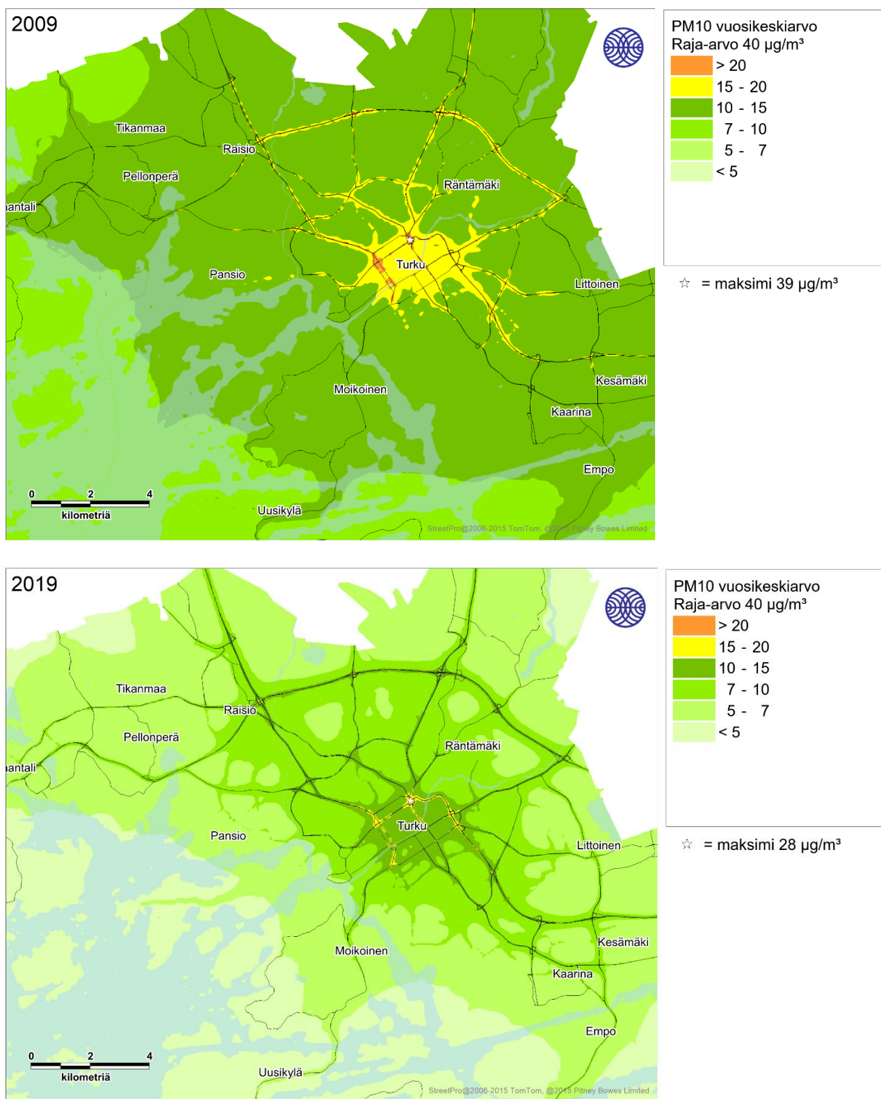
Kuva 36. Vuonna 2009 ja 2019 mallinnettu aiheuttama hengitettävien hiukkasten (PM 10 ) korkein vuosikeskiarvopitoisuus (µg/m³) Turun seudulla.
