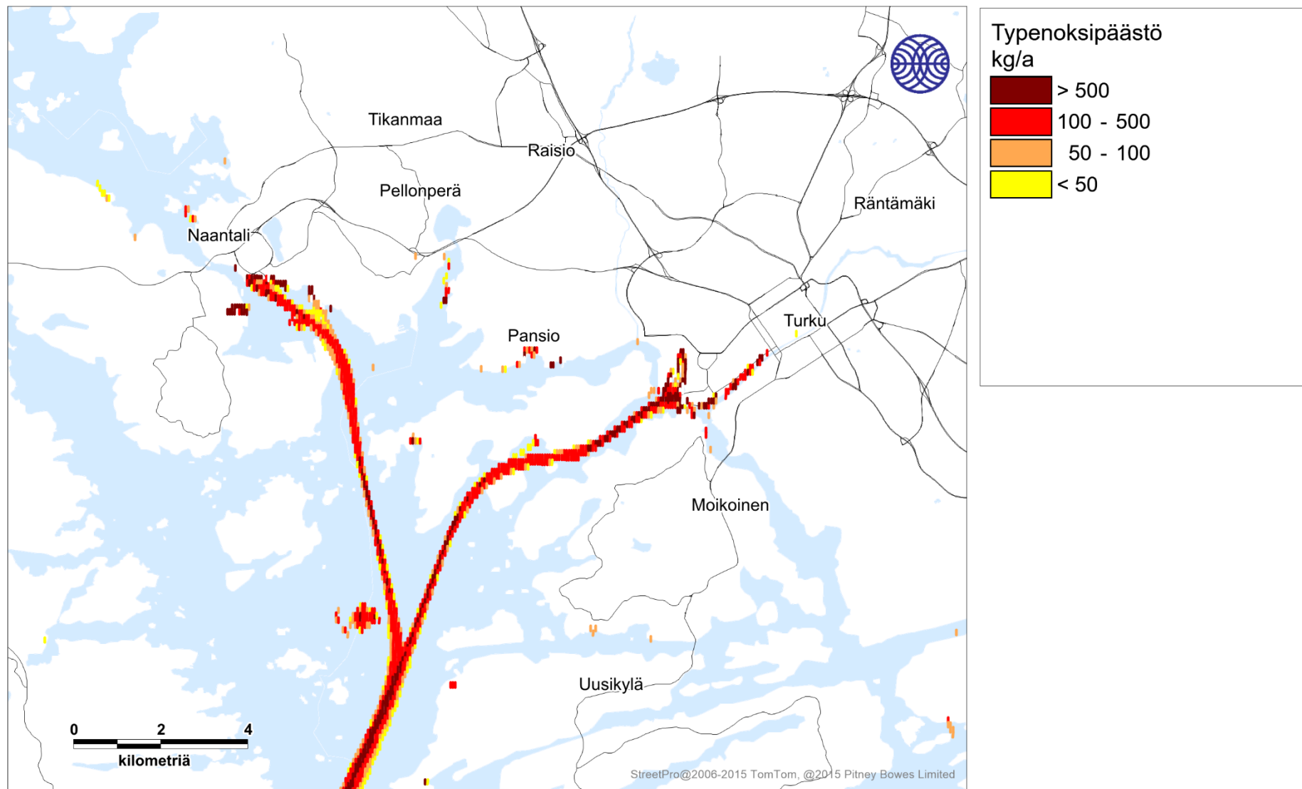
Kuva 71. Laivaliikenteen NOx-päästöt (kg/a/m) vuonna 2018.
