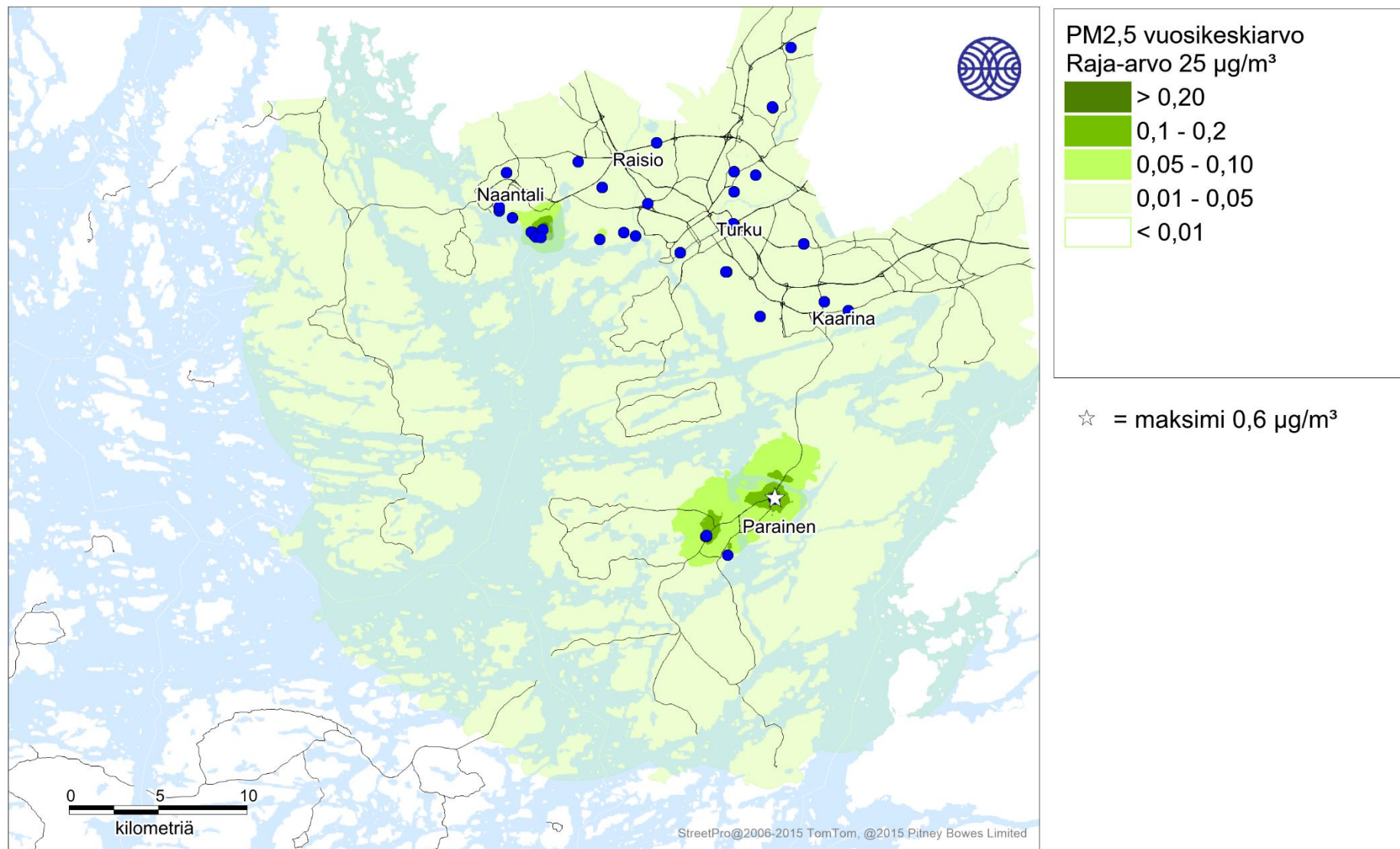
Kuva 27. Energiantuotannon ja teollisuuden päästöjen aiheuttama pienhiukkasten korkein vuosikeskiarvopitoisuus (µg/m³) tarkastelujaksolla 2016-2018.
